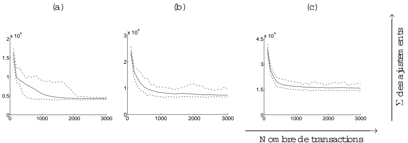
FIG. III.1: Évolution de la somme des ajustements au long des transactions de 3 simulations : (a) avec 4 individus, (b) avec 6 individus et (c) avec 7 individus ; la courbe en trait plein représente la moyenne des valeurs de la somme des ajustements pour l'ensemble des simulations, la courbe en pointillés schématise les valeurs minimales alors que les valeurs maximales sont illustrées par la courbe en traits discontinus.
