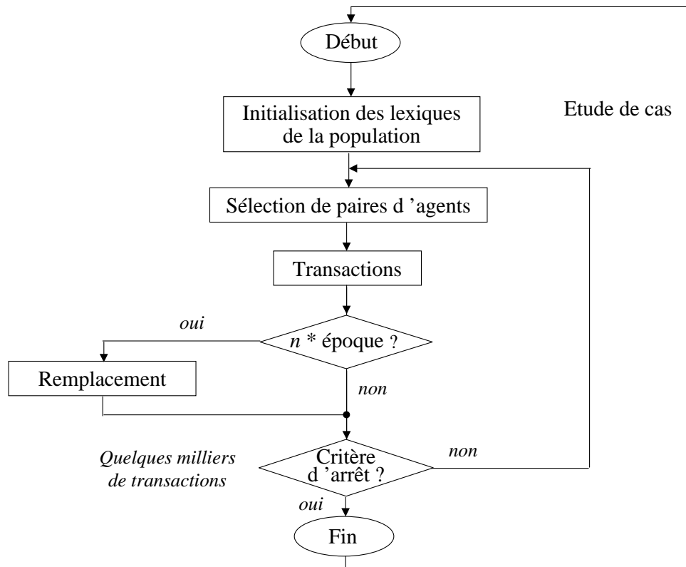
FIG. II.11: Organigramme d'une simulation type du modèle ESPECE.
