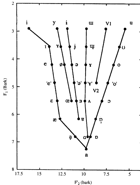
FIG. III.11: Prototypes vocaliques dans l'espace acoustique ( F_1 , F_2 ) (d'après Schwartz et al. (1997b)).
