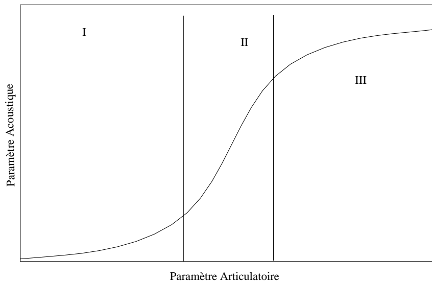
FIG. I.4: Non linéarité du passage d'un paramètre de commande articulatoire à un paramètre de sortie acoustique dans le postulat de base de la Théorie Quantique (d'après Stevens (1972)).
