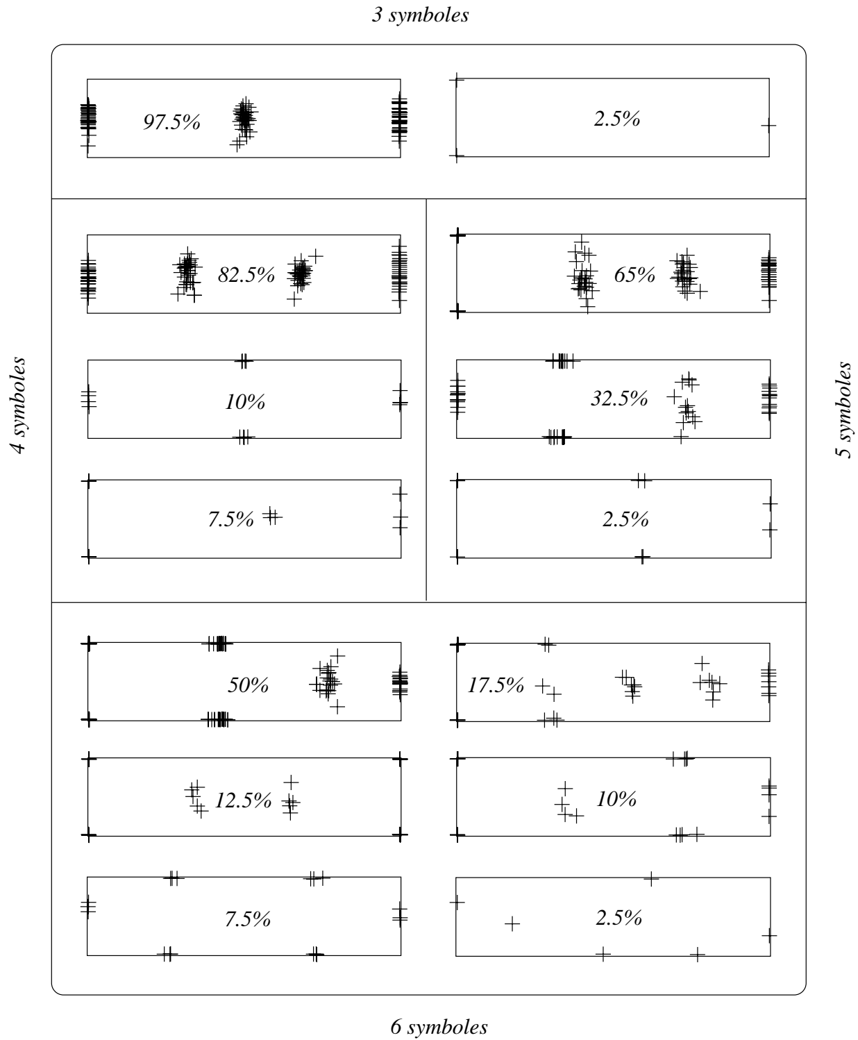
FIG. IV.6: Exploitation progressive de la seconde dimension dans des systèmes utilisant 3-, 4-, 5- et 6-symboles. Les pourcentages indiquent les statistiques sur 40 simulations effectuées.
