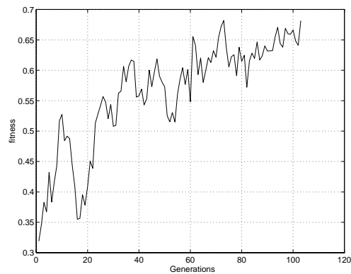
FIG. I.8: Évolution de la fitness pour une population de 12 robots (d'après Golin (1995)).
