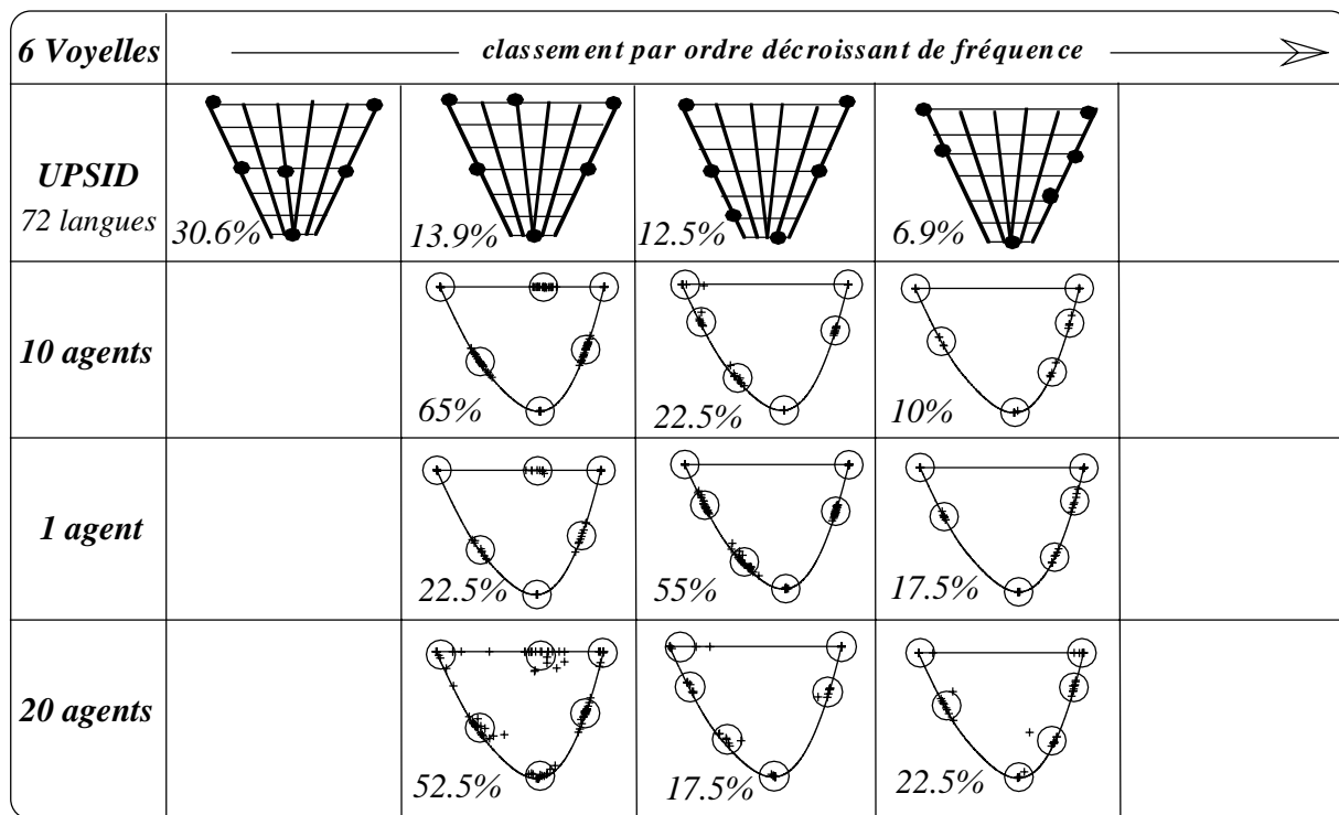
FIG. C.4: Distribution dans le triangle vocalique de voyelles de sociétés d'un, dix et vingt agents ayant un lexique de 6 voyelles.
