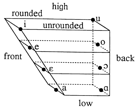
FIG. IV.1: Les dimensions des traits de base (d'après Ladefoged & Maddieson (1990)).
