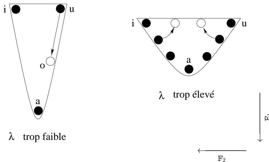
FIG. III.12: Effet du facteur \lambda : Une valeur trop élevée favorise les voyelles centrales, alors qu'une valeur trop petite pénalise la voyelle /u/.
