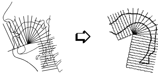
FIG. 1.7: Modèle de Mæda : de l'analyse à la génération de la coupe sagittale
