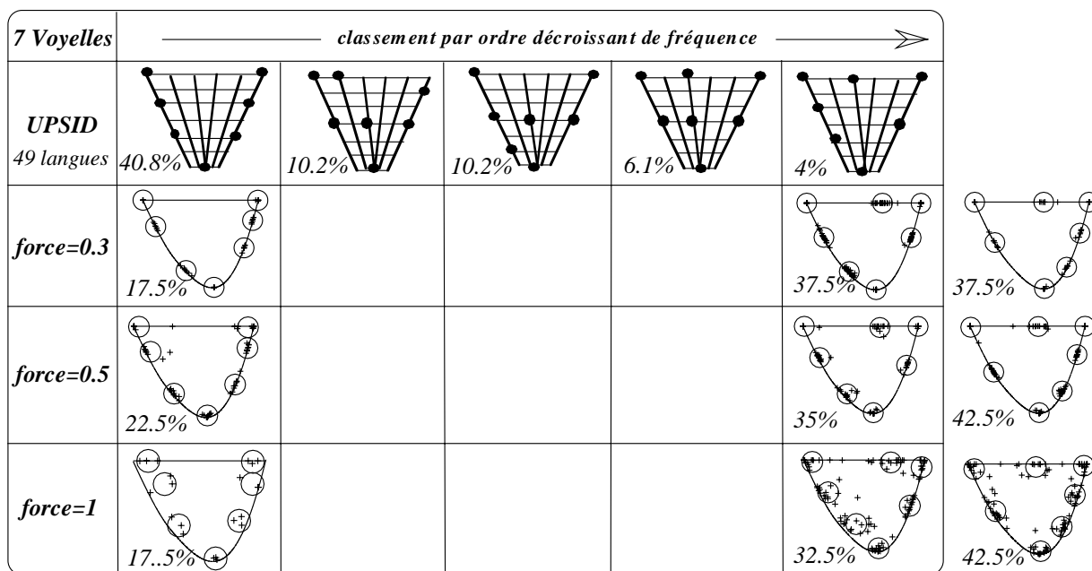
FIG. E.4: Distribution dans le triangle vocalique des voyelles d'une société de dix agents ayant un lexique de 7 voyelles avec des forces de répulsion égales à 0,3, 0,5 et 1.
