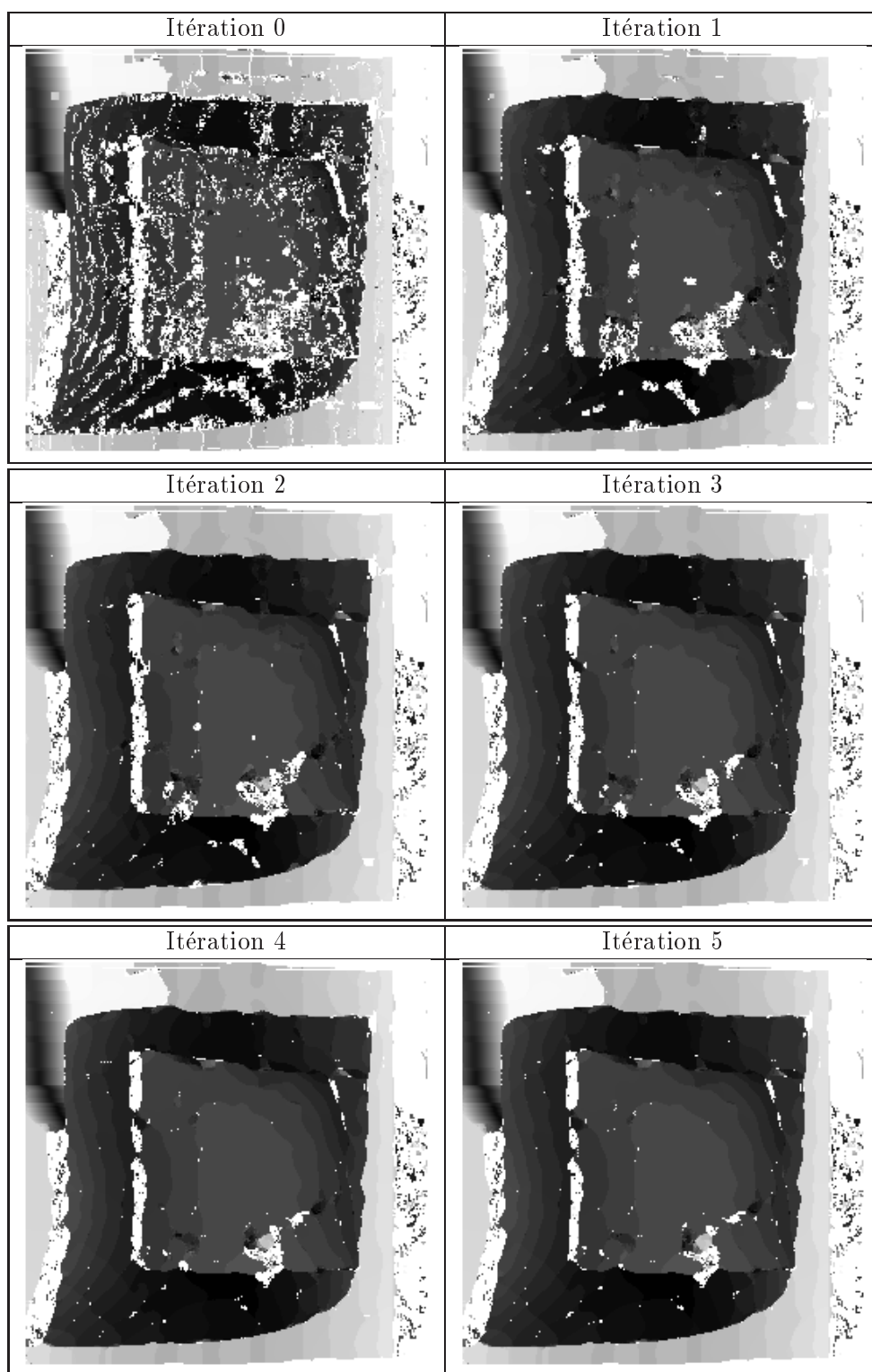
FIG. 3.43: Les cartes de disparité du couple (i m_0, i m_1) , à différents stades de régularisation.
