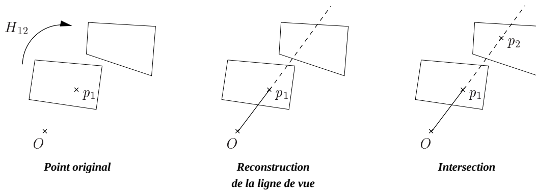
FIG. 2.5: Le transfert homographique d'un point peut être vu comme la reconstruction de la ligne de vue passant par ce point, suivie de sa reprojektion (intersection avec le nouveau plan-image).
