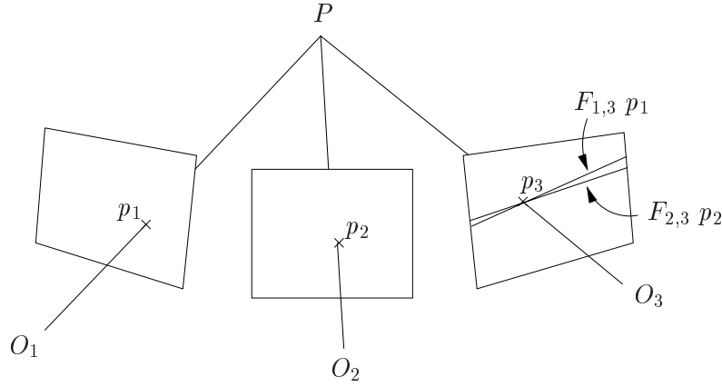
FIG. 2.3: Le transfert par intersection des épipolaires fonctionne mal pour les points P proches du plan trifocal (O_1O_2O_3) .
