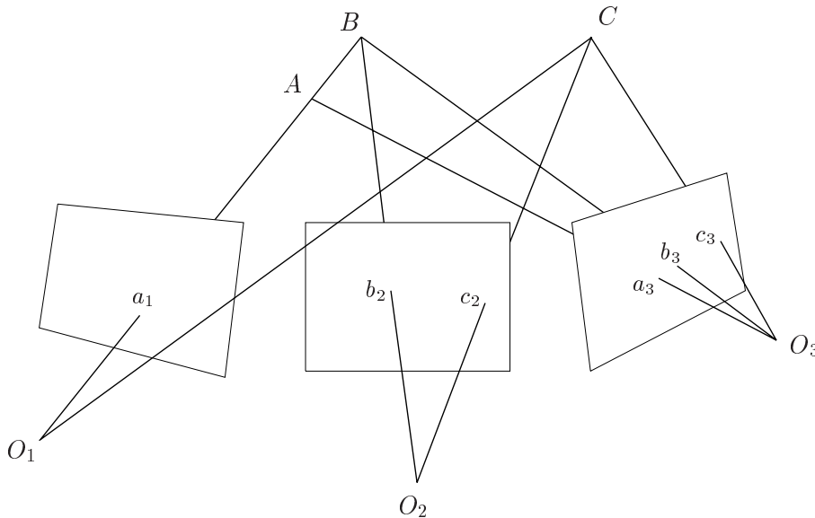
FIG. 3.1: Définition d'un appariement (voir texte) ; les appariements existants sont (a_1, a_3) , (a_1, b_2, b_3) et (c_2, c_3) .
