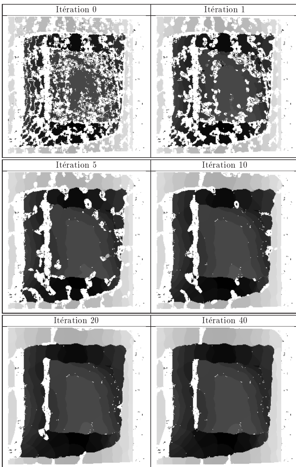
FIG. 3.37: Les cartes de disparité du couple (i m_0, i m_1) , à différents stades de régularisation.
