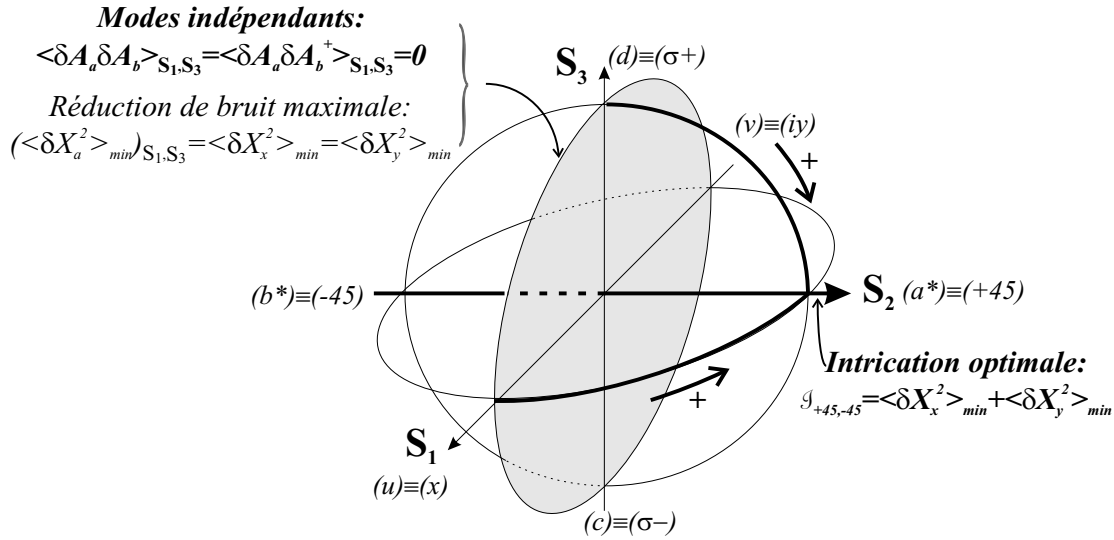
Fig. 5.12 – Propriétés quantiques du système dans la limite haute fréquence. La sphère de Poincaré est définie par rapport à la base (x, y) \equiv (x, -iy) . Les modes polarisés circulairement sont indépendants, de même pour les modes x et y . La meilleure intrication a lieu pour les modes polarisés à 45^\circ . Les flèches correspondent à une augmentation des corrélations lorsque l'on se déplace sur la sphère.
