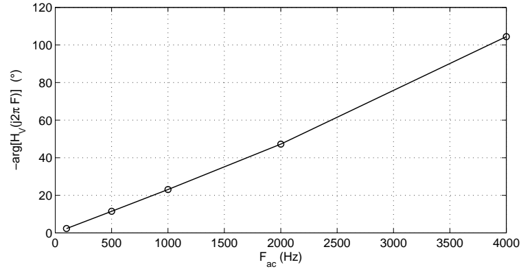
FIG. 5.8 – Évolution, en fonction de la fréquence, de la rotation de phase engendrée par un filtre passe-bas du troisième ordre de fréquence de coupure de 5 kHz.
