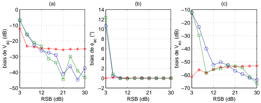
FIG. C.14 – Biais d'estimation des méthodes PDBE ( \square ), MLE ( \circ ) et EKF ( * ) en fonction du RSB. F_{ac} = 4000 Hz, V_{ac} = 1 mm/s, V_{ec} = 1,2 mm/s. (a) V_{ac} , (b) \phi_{ac} , (c) V_{ec} .
