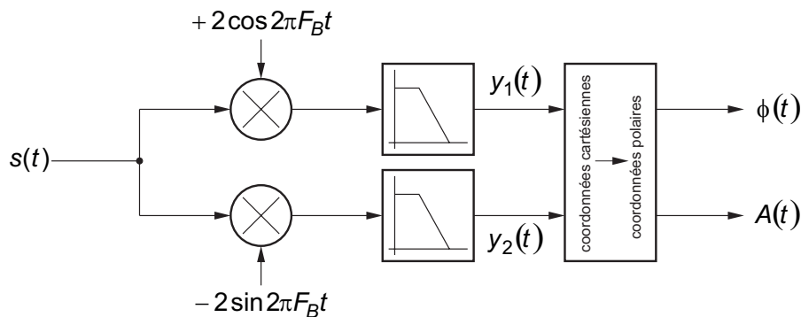
FIG. 2.13 – Schéma de principe d'un système de démodulation en quadrature.
