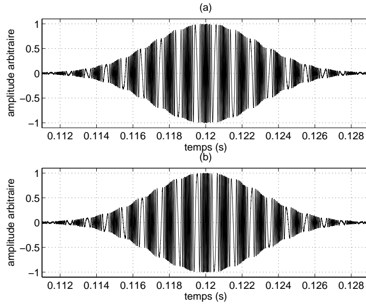
FIG. 2.18 – Visualisation des deux signaux d'observation en quadrature : signal en phase y_1(k) (a), signal en quadrature y_2(k) (b). F_{ac} = 1000 Hz, V_{ac} = 10 mm/s et V_{ec} = 12 mm/s.
