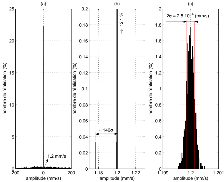
FIG. 3.19 – Répartition des résultats de l'estimation du paramètre V_{ec} pour trois échelles (a), (b) et (c) différentes. F_{ac} = 100 Hz, V_{ac} = 10 mm/s, V_{ec} = 1,2 mm/s, RSB = 3 dB.
