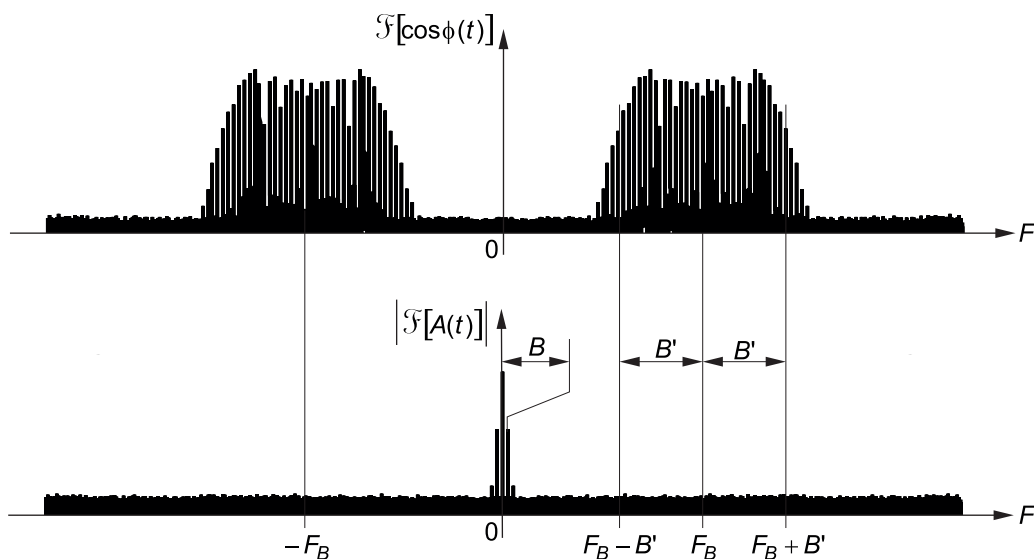
FIG. 2.17 – Comparaison des largeurs spectrales de A(t) et de \cos \phi(t) .
