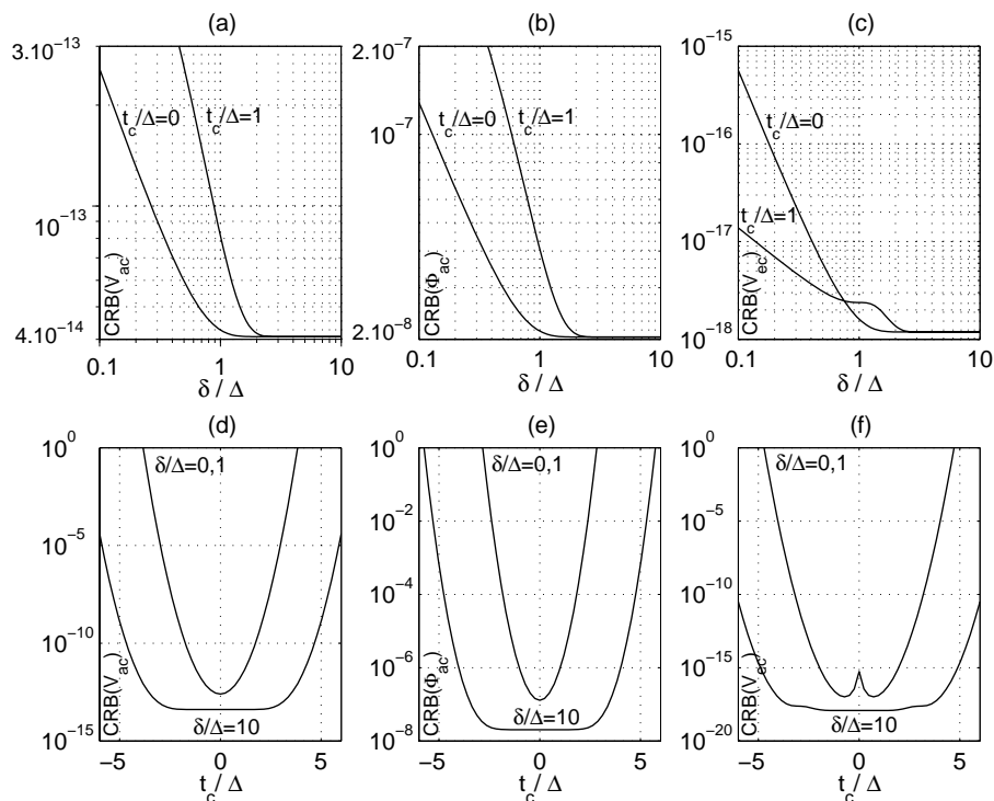
FIG. 3.2 – Influence de la valeur relative t_c/\Delta de la position du centre de la fenêtre d'analyse sur \text{CRB}(V_{ac}) (a), \text{CRB}(\phi_{ac}) (b) et \text{CRB}(V_{ec}) (c). Influence de la durée relative d'analyse \delta/\Delta sur \text{CRB}(V_{ac}) (d), \text{CRB}(\phi_{ac}) (e) et \text{CRB}(V_{ec}) (f).
