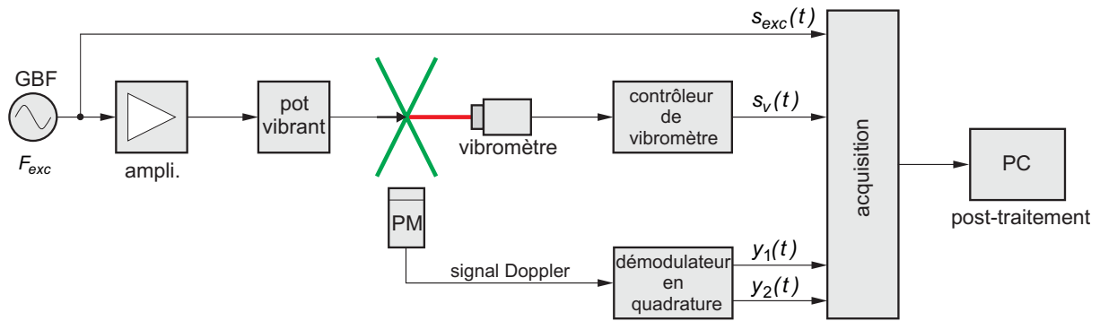
FIG. 5.3 – Organisation du dispositif expérimental de mesure de la vitesse d'une pointe d'aiguille.
