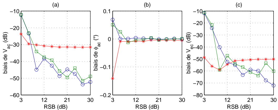
FIG. C.15 – Biais d'estimation des méthodes PDBE ( \square ), MLE ( \circ ) et EKF ( * ) en fonction du RSB. F_{ac} = 4000 Hz, V_{ac} = 10 mm/s, V_{ec} = 1,2 mm/s. (a) V_{ac} , (b) \phi_{ac} , (c) V_{ec} .
