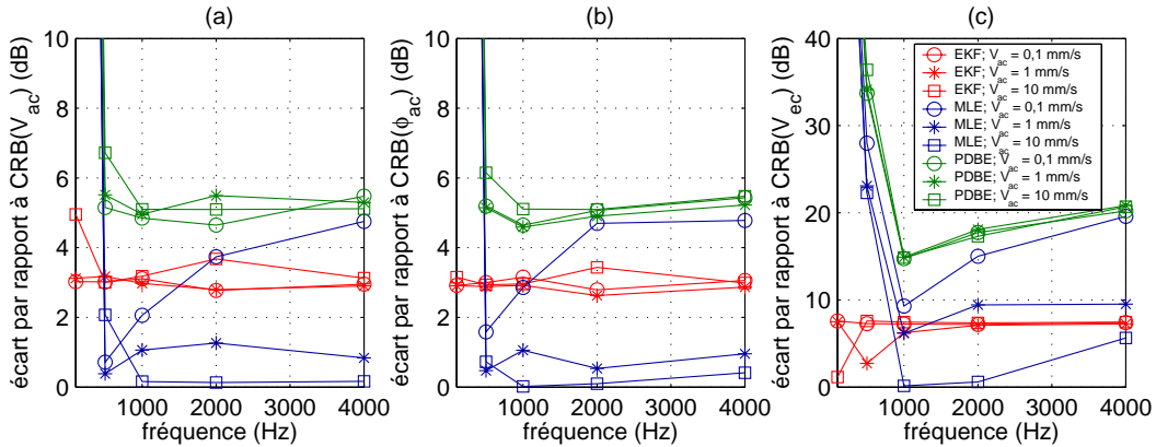
FIG. 4.5 – Variations d'estimation des méthodes PDBE ( \square ), MLE ( \circ ) et EKF ( * ) en fonction de F_{ac} . RSB = 30 dB.
