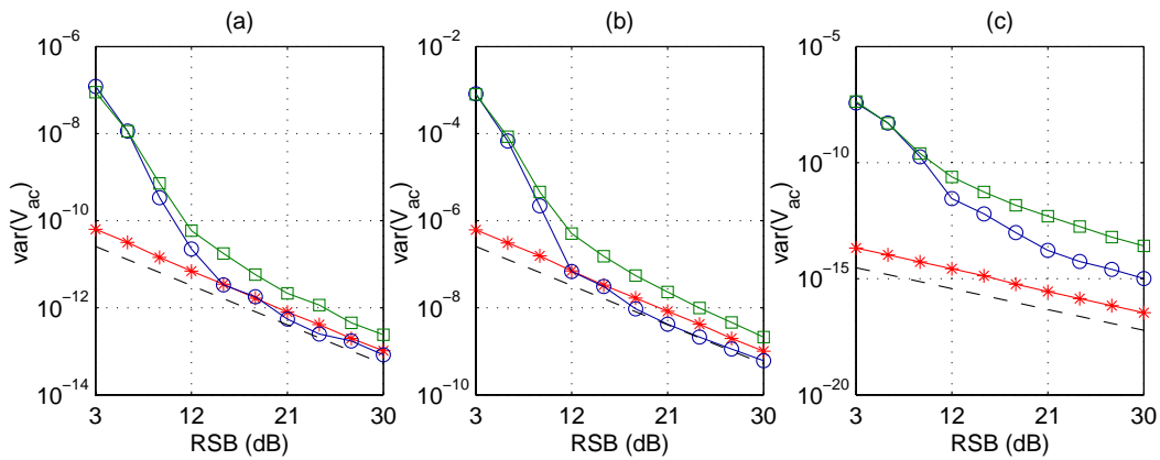
FIG. C.21 – Variance d'estimation des méthodes PDBE ( \square ), MLE ( \circ ), EKF ( * ) et CRB (--) en fonction du RSB. F_{ac} = 500 Hz, V_{ac} = 10 mm/s, V_{ec} = 1,2 mm/s.
