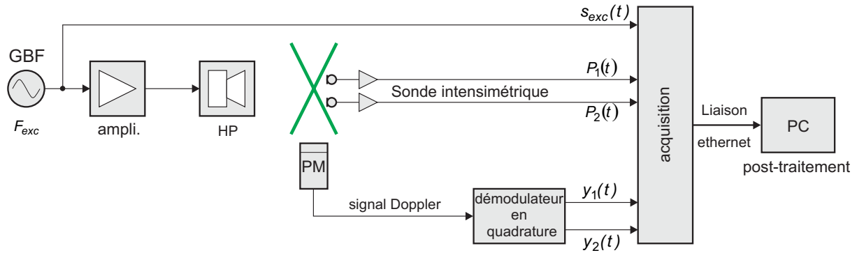
FIG. 5.10 – Organisation du dispositif expérimental de mesure de la vitesse particulaire acoustique rayonnée par un haut-parleur.
