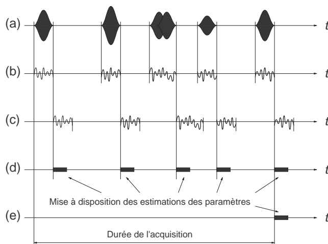
FIG. 2.14 – Notion d'estimation en temps réel: (a) Séquence Doppler - (b) Estimation en temps réel de la vitesse acoustique - (c) Estimation en ligne de la vitesse acoustique - (d) Estimation en ligne des paramètres de la vitesse acoustique - (e) Estimation différée des paramètres de la vitesse acoustique.
