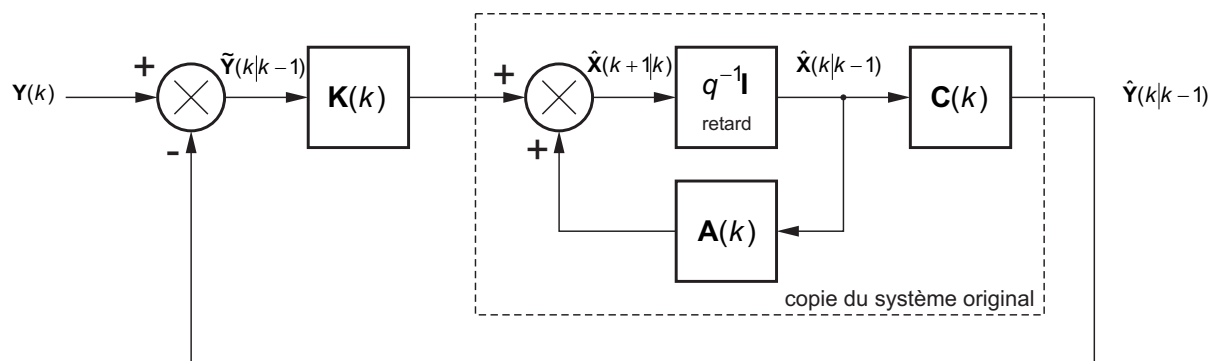
FIG. 3.12 – Représentation graphique de l'algorithme de Kalman.
