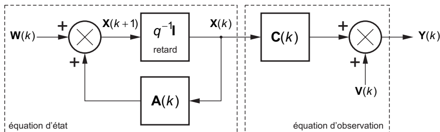
FIG. 3.11 – Schéma général d'un modèle de signal dans l'espace d'état.
