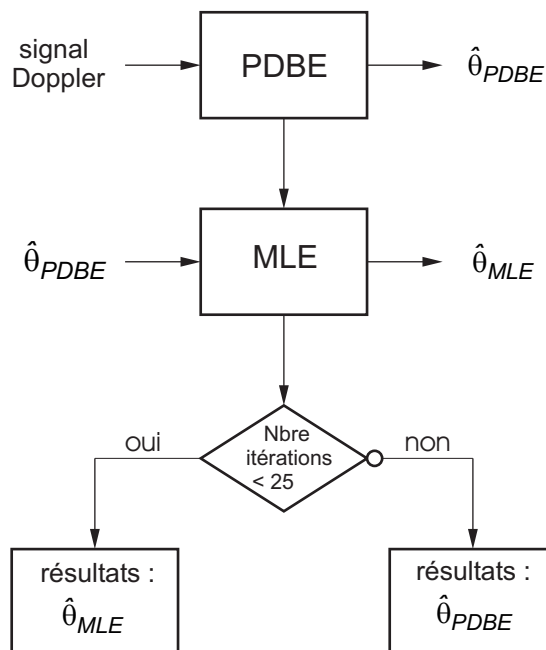
FIG. 3.9 – Principe de la procédure d'estimation par MLE initialisée par la méthode PDBE.
