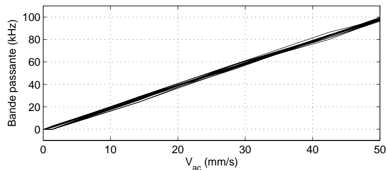
FIG. 2.11 – Bandes passantes à -3 dB simulées en fonction de la vitesse acoustique pour différentes valeurs de la fréquence F_{ac} comprises entre 500 Hz et 4000 Hz.
