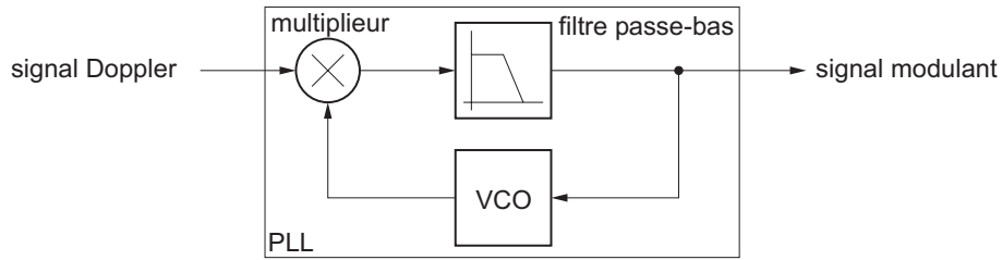
FIG. 2.12 – Schéma de principe d'une boucle à verrouillage de phase (PLL).
