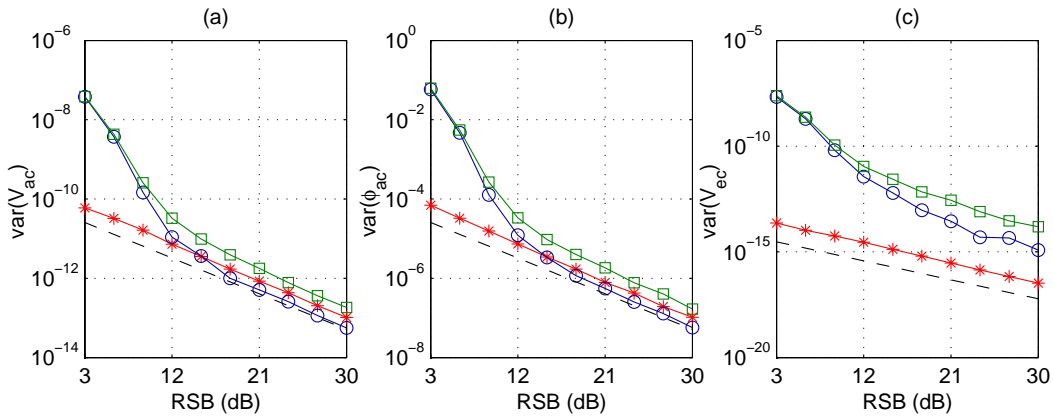
FIG. C.20 – Variance d'estimation des méthodes PDBE ( \square ), MLE ( \circ ), EKF ( * ) et CRB (--) en fonction du RSB. F_{ac} = 500 Hz, V_{ac} = 1 mm/s, V_{ec} = 1,2 mm/s.
