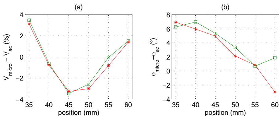
FIG. 5.20 – Erreurs relatives entre les amplitudes des vitesses mesurées et les valeurs estimées par mesure de pression (a) et erreurs de phase (b). EKF (*) et PDBE ( \square ). F_{ac} = 2000 Hz.
