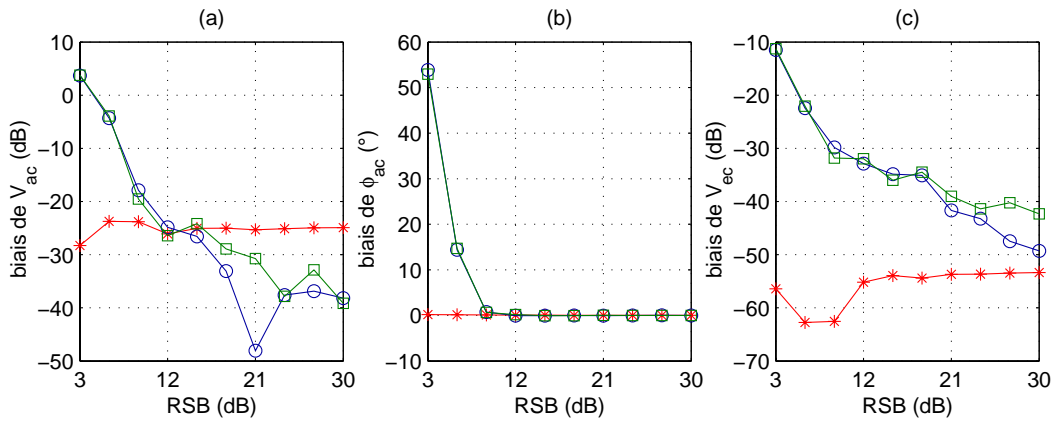
FIG. C.4 – Biais d'estimation des méthodes PDBE ( \square ), MLE ( \circ ) et EKF ( * ) en fonction du RSB. F_{ac} = 500 Hz, V_{ac} = 0,1 mm/s, V_{ec} = 1,2 mm/s. (a) V_{ac} , (b) \phi_{ac} , (c) V_{ec} .
