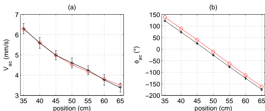
FIG. 5.15 – Profils des amplitudes (a) et de la phase (b) de la vitesse acoustique mesurées par ALD et estimées par PDBE (noir) et à partir de deux pressions (rouge). F_{ac} = 1000 Hz.
