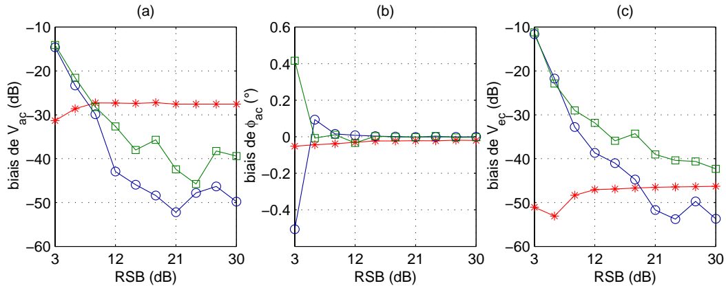
FIG. C.5 – Biais d'estimation des méthodes PDBE ( \square ), MLE ( \circ ) et EKF ( * ) en fonction du RSB. F_{ac} = 500 Hz, V_{ac} = 1 mm/s, V_{ec} = 1,2 mm/s. (a) V_{ac} , (b) \phi_{ac} , (c) V_{ec} .
