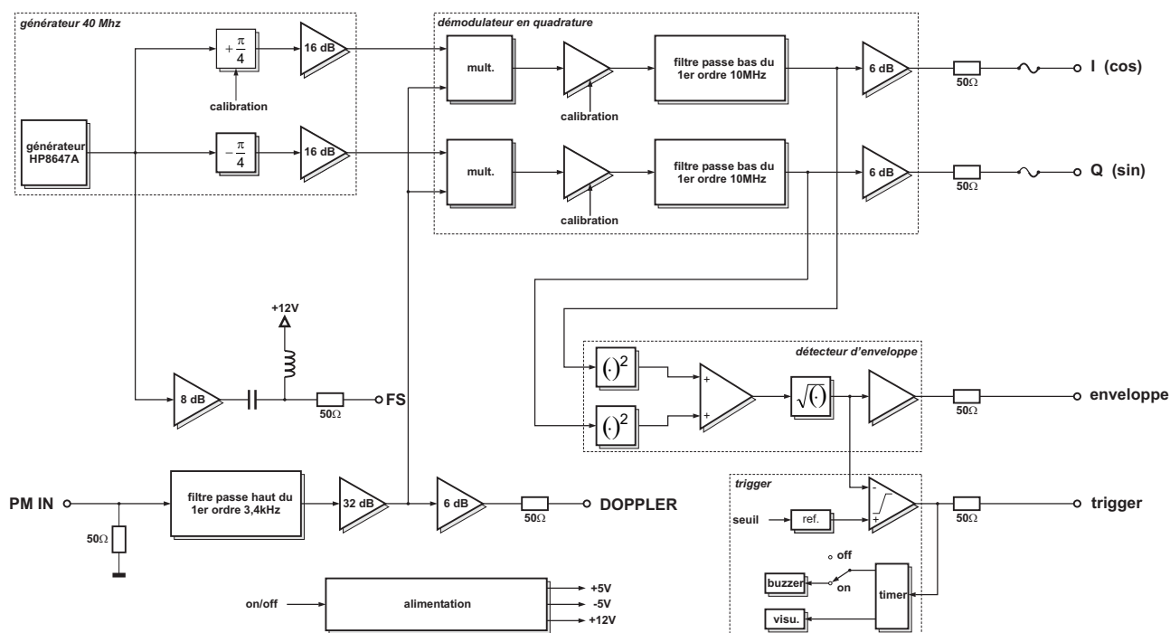
FIG. 5.2 – Organisation du démodulateur en quadrature 40 MHz.
