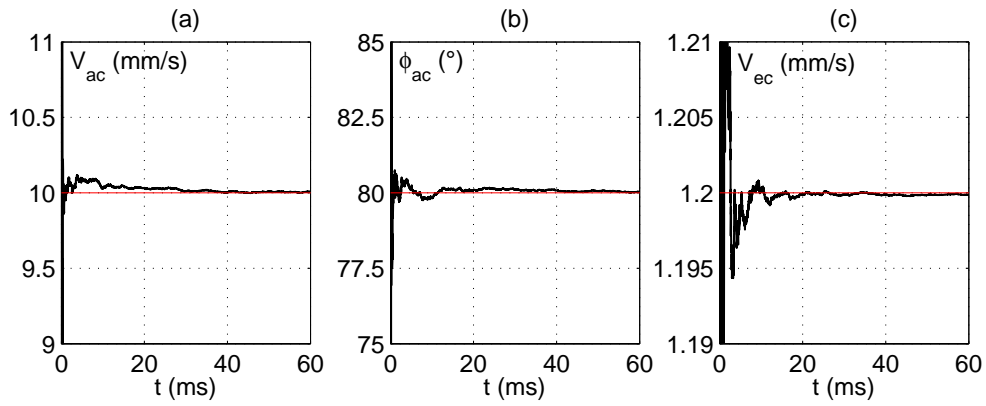
FIG. 3.16 – Exemple d'estimation des paramètres de la vitesse acoustique par EKF. V_{ac} = 10 mm/s, \phi_{ac} = 80^\circ et V_{ec} = 1,2 mm/s, RSB = 3 dB.
