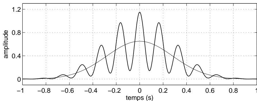
FIG. 2.7 – Allure du signal Doppler (-) pour t_0 = 0 , K = 0,5 , M = 1,3 , \beta = 250 \text{ m}^{-1} , V_x = 10 \text{ mm/s} , D = 600 \text{ m}^{-1} et \phi_0 = 0 ; piédestal (-).
