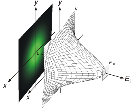
FIG. 2.6 – Répartition radiale de l'intensité lumineuse dans un faisceau laser fonctionnant en mode TEM 00 .
