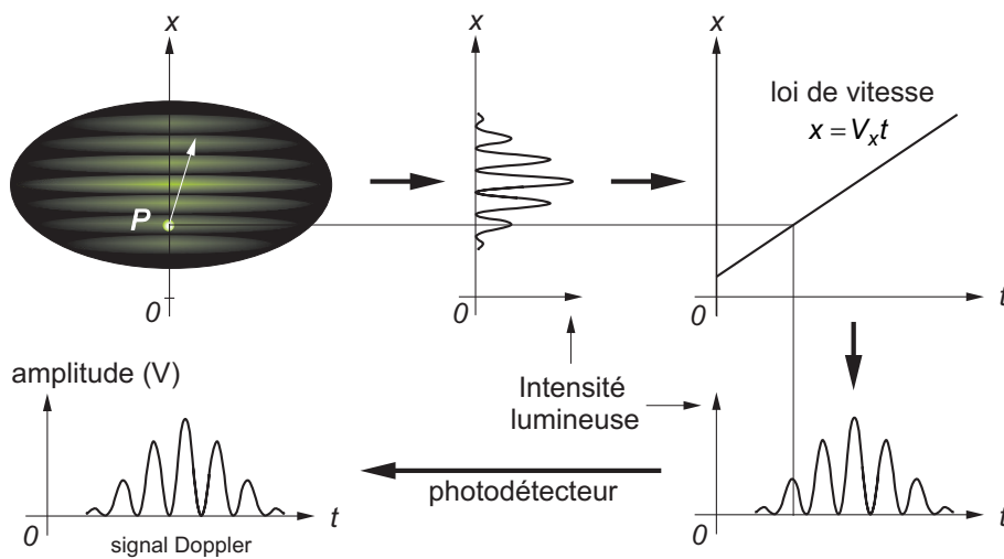
FIG. 2.4 – Formation du signal Doppler dans le cas où la vitesse particulaire est constante.
