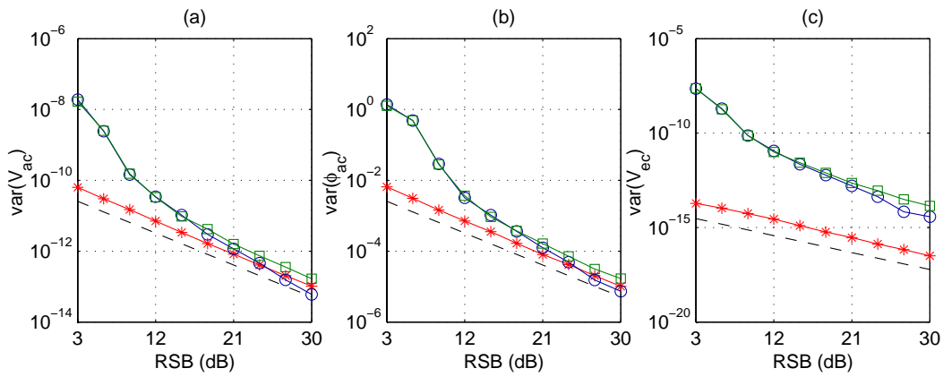
FIG. C.19 – Variance d'estimation des méthodes PDBE ( \square ), MLE ( \circ ), EKF ( * ) et CRB (--) en fonction du RSB. F_{ac} = 500 Hz, V_{ac} = 0,1 mm/s, V_{ec} = 1,2 mm/s.
