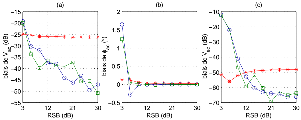
FIG. C.8 – Biais d'estimation des méthodes PDBE ( \square ), MLE ( \circ ) et EKF ( * ) en fonction du RSB. F_{ac} = 1000 Hz, V_{ac} = 1 mm/s, V_{ec} = 1,2 mm/s. (a) V_{ac} , (b) \phi_{ac} , (c) V_{ec} .
