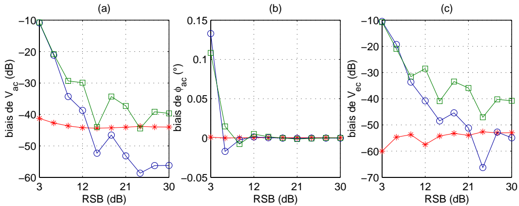
FIG. C.6 – Biais d'estimation des méthodes PDBE ( \square ), MLE ( \circ ) et EKF ( * ) en fonction du RSB. F_{ac} = 500 Hz, V_{ac} = 10 mm/s, V_{ec} = 1,2 mm/s. (a) V_{ac} , (b) \phi_{ac} , (c) V_{ec} .
