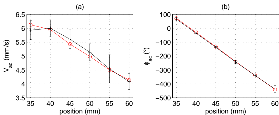
FIG. 5.19 – Profils des amplitudes (a) et de la phase (b) de la vitesse acoustique mesurées par ALD et estimées par EKF (noir) et à partir de deux pressions (rouge). F_{ac} = 2000 Hz.
