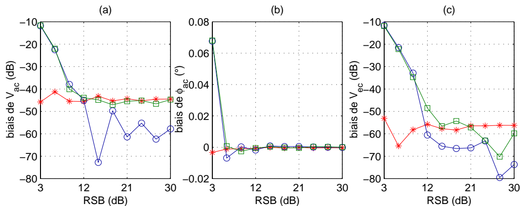
FIG. 4.2 – Biases relatifs d'estimation des méthodes PDBE ( \square ), MLE ( \circ ) et EKF ( * ) en fonction du RSB. F_{ac} = 1000 Hz, V_{ac} = 10 mm/s, V_{ec} = 1,2 mm/s. (a) V_{ac} , (b) \phi_{ac} , (c) V_{ec} .
