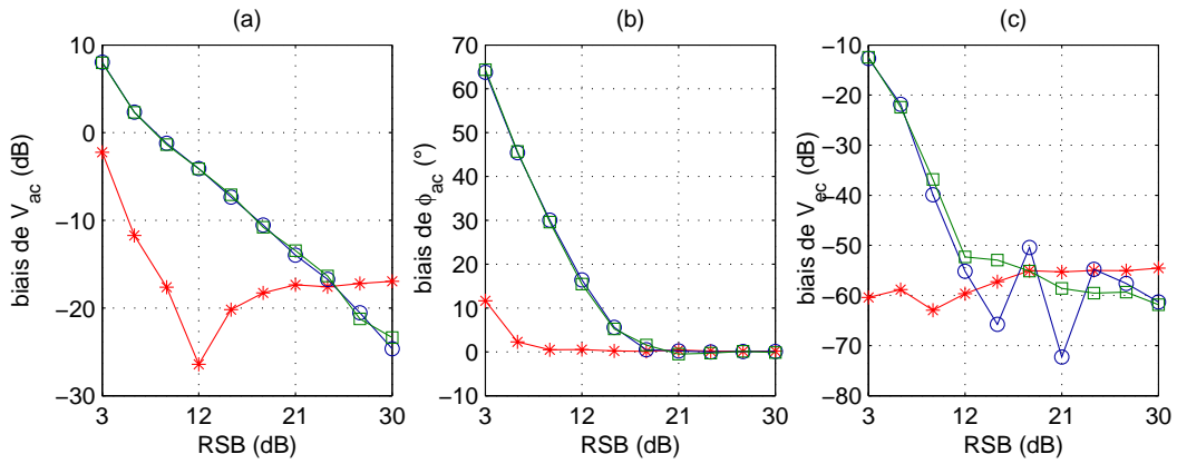
FIG. C.13 – Biais d'estimation des méthodes PDBE ( \square ), MLE ( \circ ) et EKF ( * ) en fonction du RSB. F_{ac} = 4000 Hz, V_{ac} = 0,1 mm/s, V_{ec} = 1,2 mm/s. (a) V_{ac} , (b) \phi_{ac} , (c) V_{ec} .
