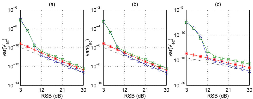
FIG. C.24 – Variance d'estimation des méthodes PDBE ( \square ), MLE ( \circ ), EKF ( * ) et CRB (- -) en fonction du RSB. F_{ac} = 1000 Hz, V_{ac} = 10 mm/s, V_{ec} = 1,2 mm/s.
