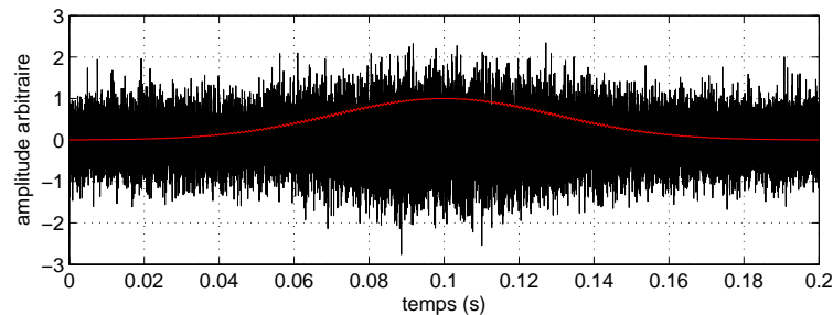
FIG. 4.1 – Signal d’observation en phase y_1(t) pour \text{RSB} = 3 dB et l’enveloppe réelle correspondante en rouge. F_{\text{ac}} = 1000 Hz, V_{\text{ac}} = 10 mm/s et V_{\text{ec}} = 1,2 mm/s.
