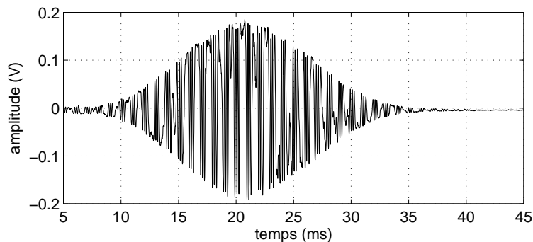
FIG. 5.14 – Composante en phase y_1(t) du signal Doppler. Résultat expérimental obtenu pour F_{ac} = 1000 Hz.
