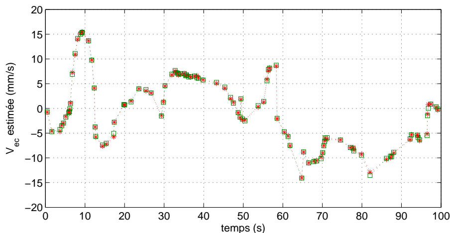
FIG. 5.21 – Exemple de vitesse d'écoulement mesuré expérimentalement. EKF (*) et PDBE ( \square ). F_{ac} = 1000 Hz.
