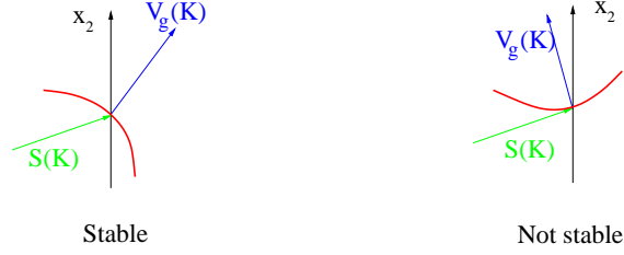
FIG. 3.1: Deux configurations différentes. Gauche: le vecteur lenteur \mathcal{S} et la vitesse de groupe \mathbf{V}_g sont orientés dans le même sens par rapport à l'axe Ox_2 . Droite: \mathcal{S} et \mathbf{V}_g ne sont pas orientés dans le même sens par rapport à l'axe Ox_2 .
