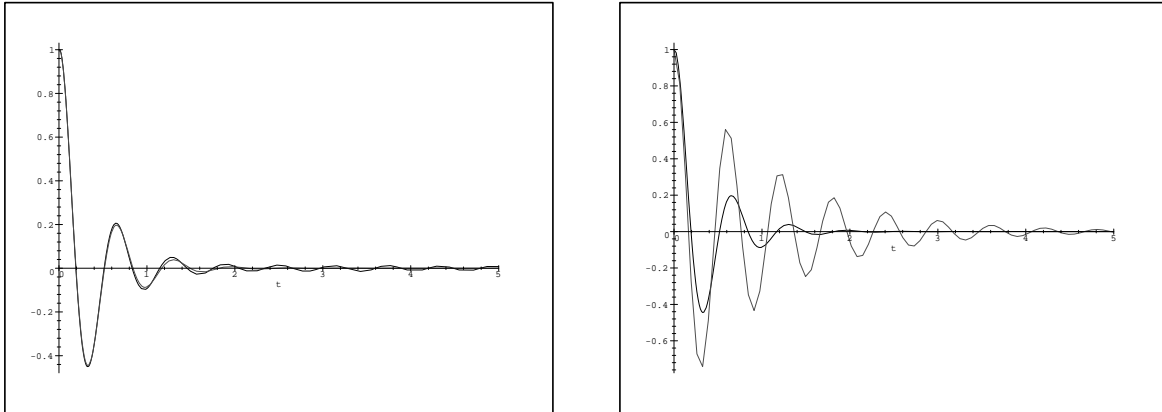
Figure 3.8: Variation de la position relative de deux particules en fonction du temps. A gauche, on utilise un pas de temps adaptatif, l'erreur commise est de 0.00006. A droite on utilise un pas de temps constant. Les deux exemples tournent à la même vitesse car on a choisi le pas constant égal au pas de temps moyen utilisé par l'approche adaptative. L'erreur commise dans ce cas est égale à 0.003. Les paramètres dynamiques sont: \lambda = 100 , \mu = 5 , \tau_m = 0.065 et, \epsilon_e = 0.01 .
