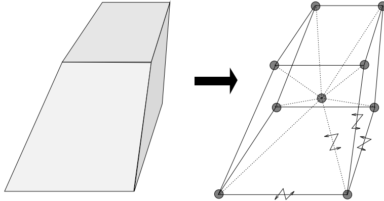
Figure 6.1: La discrétisation automatique décompose un polyèdre en plusieurs hexaèdres, chacun est défini par 8 particules.
