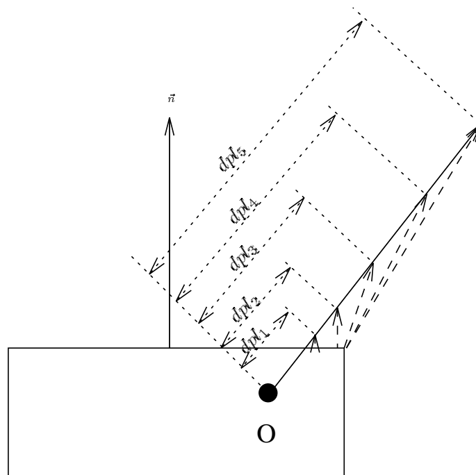
Figure 4.6: Plus le déplacement est petit, plus la direction de contact, obtenue après ce déplacement, est proche de sa valeur réelle.
