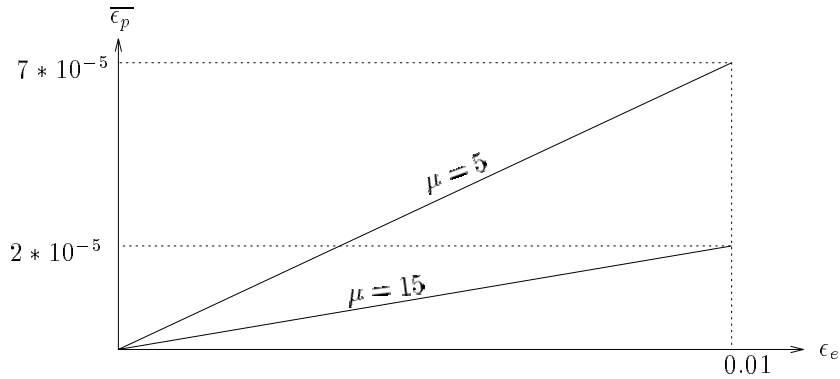
Figure 3.9: Valeur de l'erreur commise en position \epsilon_p en fonction de l'erreur commise en énergie \epsilon_e pendant 10 secondes et pour deux valeurs différentes du facteur de la viscosité \mu . Ce résultat est obtenu à l'aide de MAPLE.
