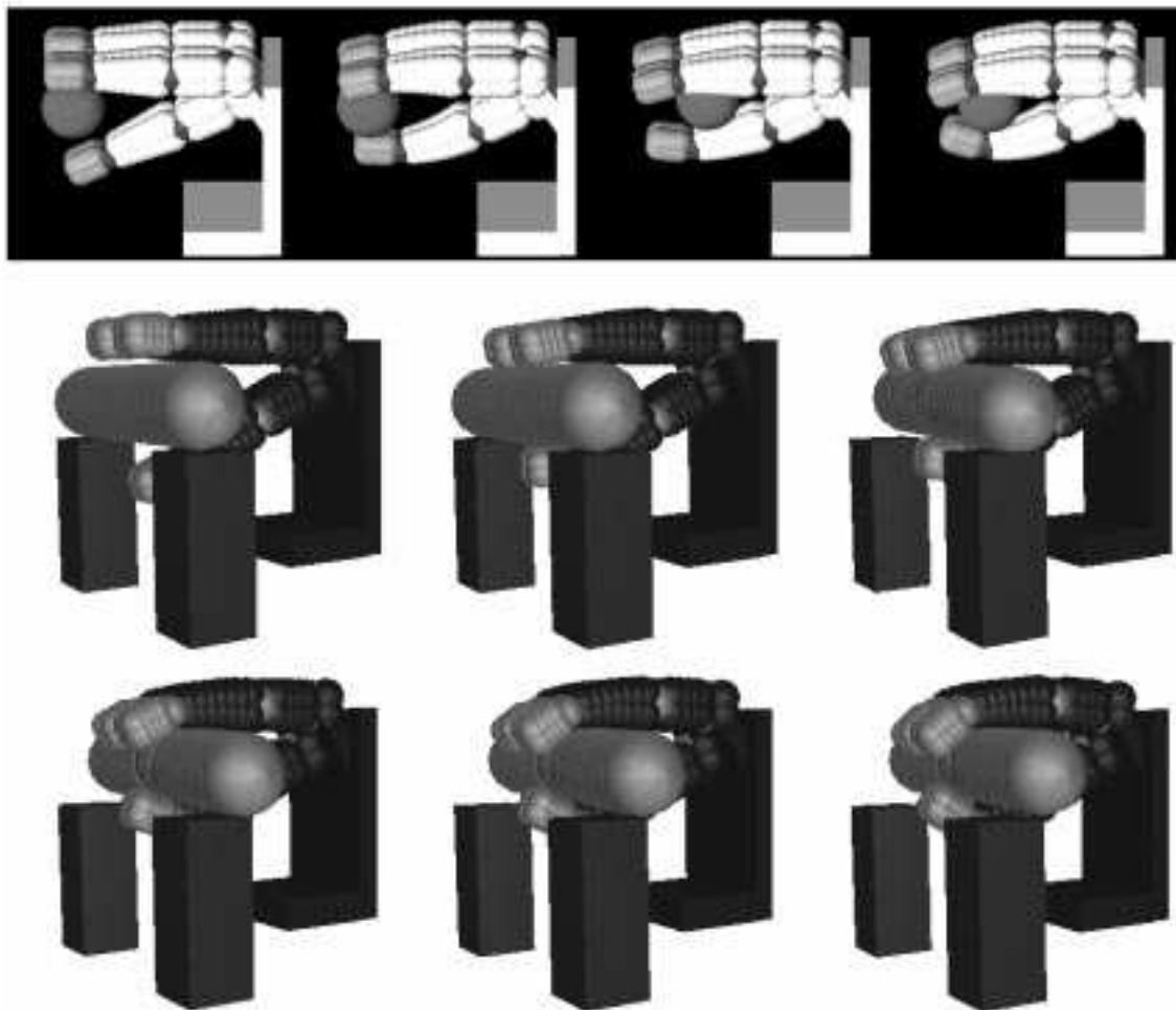
Figure 5.10: La saisie par la paume de la main rend la saisie plus stable.
