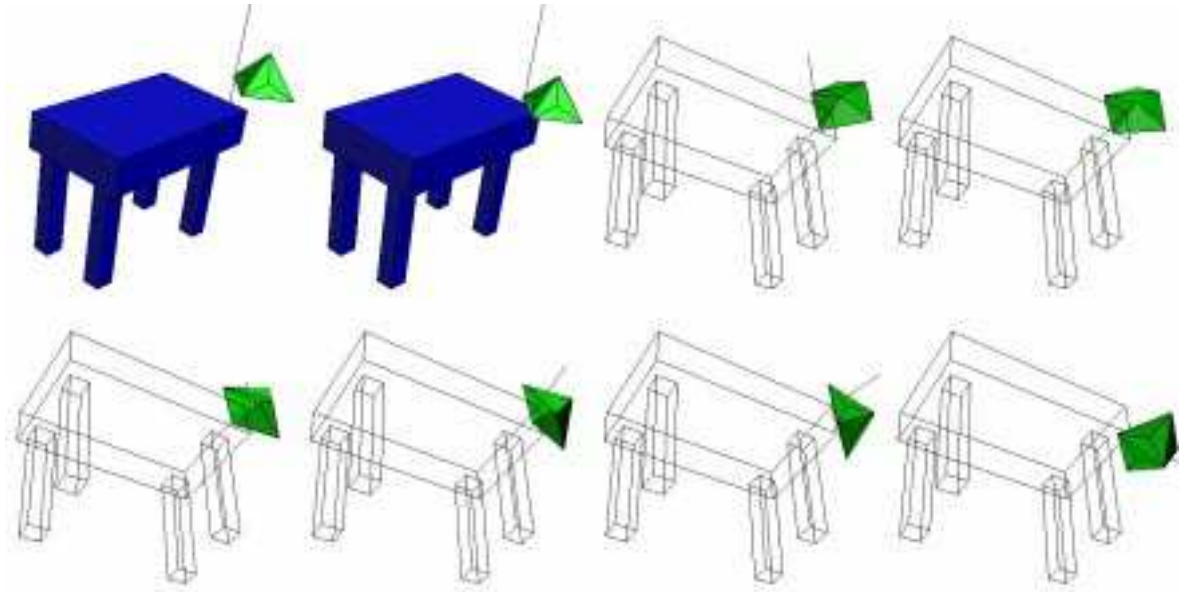
Figure 4.19: L'évolution de \vec{n}_{A/B} pendant la collision. La direction du contact est représentée par une ligne noire. Au début cette direction est perpendiculaire à la surface de la table. A cause de la force de la collision et à la force de la pesanteur, la pyramide bascule sur le sommet et la direction de contact passera par ce sommet.
