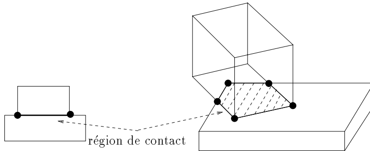
Figure 4.12: Quand deux objets sont en contact permanent, les facettes sont dans le même plan et on peut facilement calculer la zone du contact [4].
