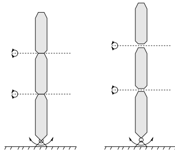
Figure 6.11: Une chaîne articulée.
