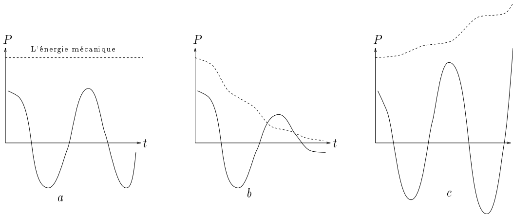
Figure 3.4: (a) Un système isolé sans dissipation interne de l'énergie: E_m est constante. (b) Un système isolé avec dissipation interne de l'énergie: E_m diminue. (c) Un système non isolé: E_m peut augmenter.
