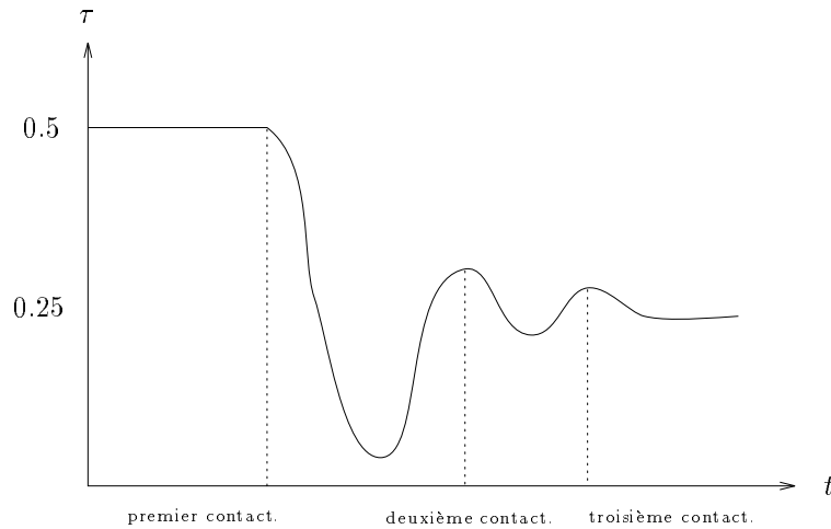
Figure 3.7: L'évolution de \tau quand une balle chute sur le sol. Remarquons que \tau diminue quand la balle touche le sol et augmente de nouveau quand la balle quitte le sol. Remarquons aussi, que la valeur de cette diminution dépend de la valeur de la force de la collision qui est plus importante quand la balle est plus rapide.
