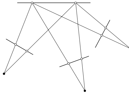
FIG. 7.6: Détermination des points cycliques avec 3 caméras linéaires calibrées.
