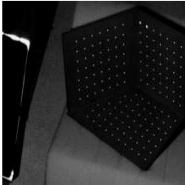
FIG. 6.7: La mire de calibrage.
