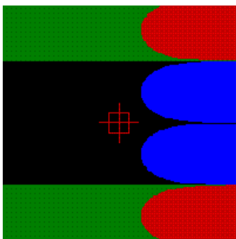
FIG. 4.13: "clearcut region" pour f(z) = \text{Exp}(z)
