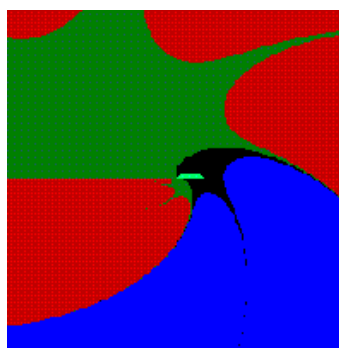
FIG. 4.18: "clearcut region" pour f(z) = z^{3+2i}
