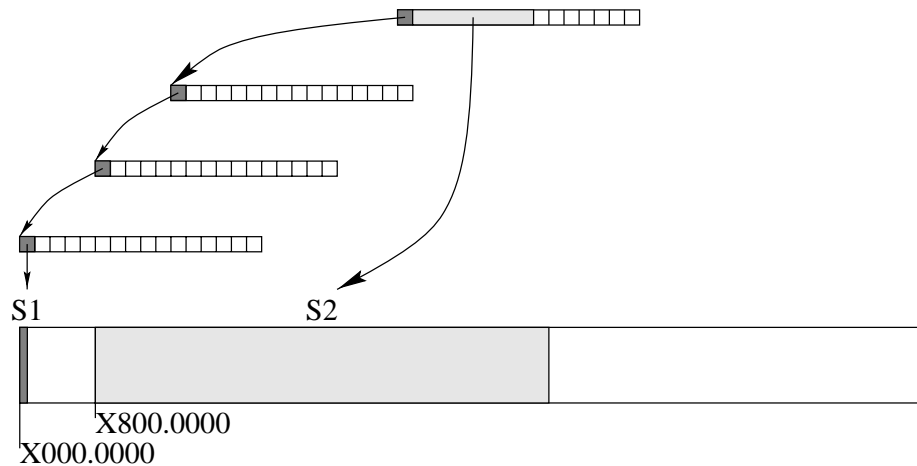
Figure III-7 : Exemple de buddy-system de base 16 couvrant 16 bits d'adresse
