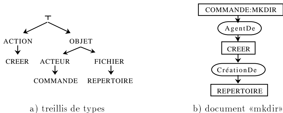
Figure 2.7. Exemple de représentation dans ELEN
