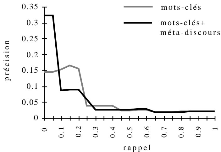
Figure 4.3. Précision/rappel pour les requêtes n os 7, 12, 16, et 23 de la CACM
