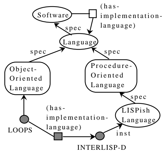
a) taxonomie des concepts
