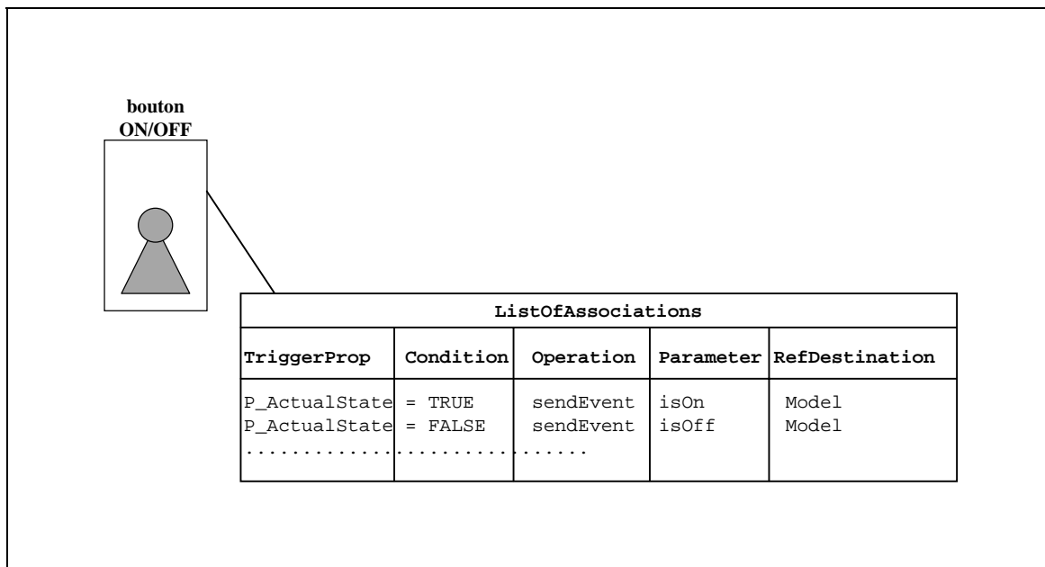
Figure 11-20 : Stockage des associations dans l'objet origine
