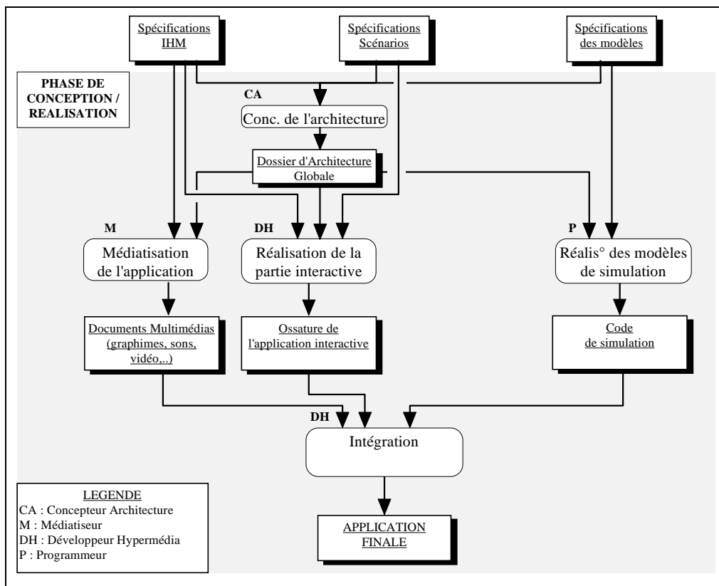
Figure 4-7 : La phase de conception-réalisation
