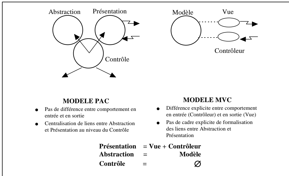
Figure 9-9 : Modèle PAC et Modèle MVC
