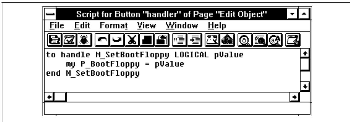
Figure 11-6 : Exemple de code OpenScript
