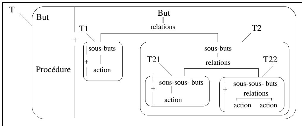
Figure 8-5 : Une définition de tâche selon S. Balbo, adaptée de [NOR 92].
