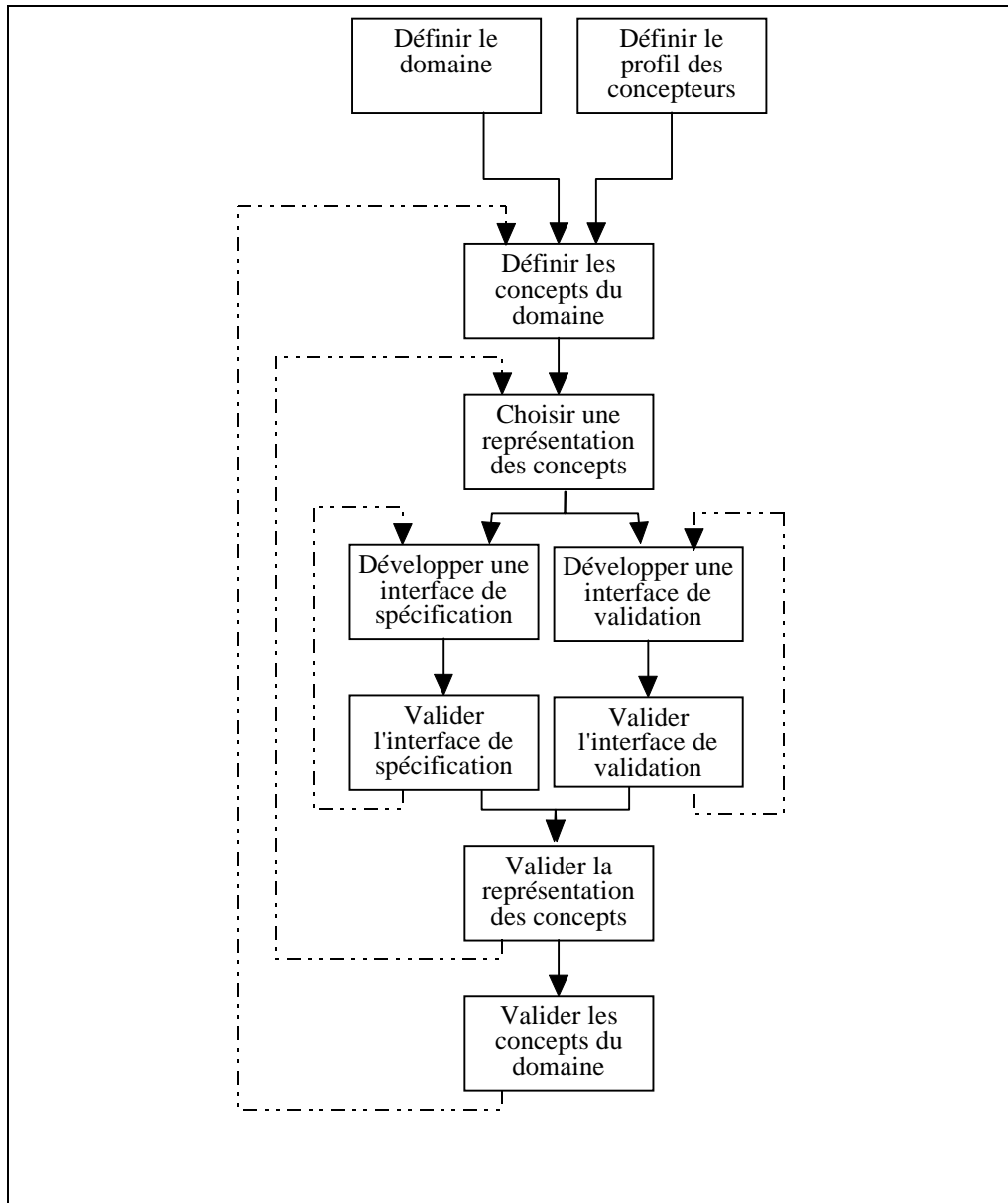
Figure 6-5 : La démarche de validation des concepts dans chaque espace de travail
