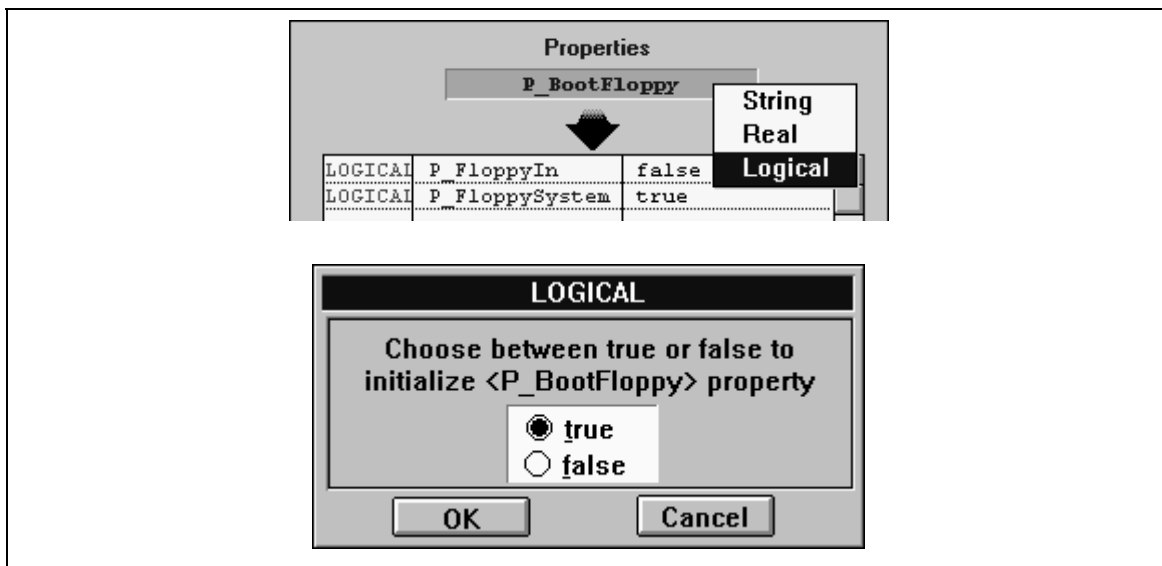
Figure 11-5 : Définition d'une propriété, de son type et de sa valeur initiale
