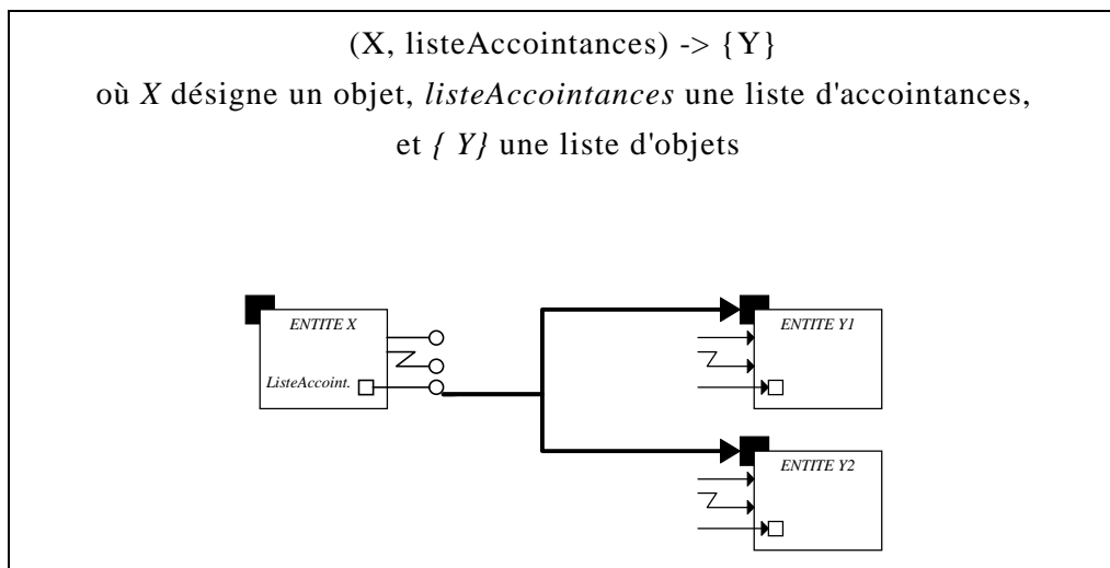
Figure 10-8 : X communique avec ses accointances Y1 et Y2
