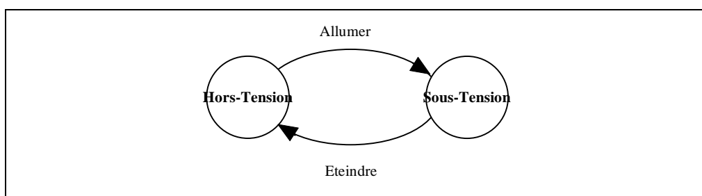
Figure 7-12 : Un exemple d'automates à états finis
