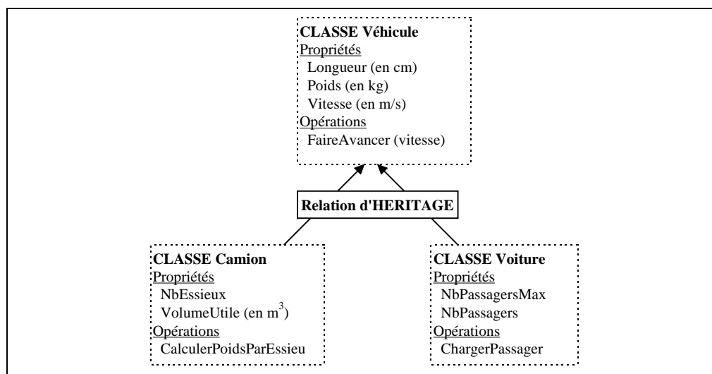
Figure 7-11 : La relation d'héritage
