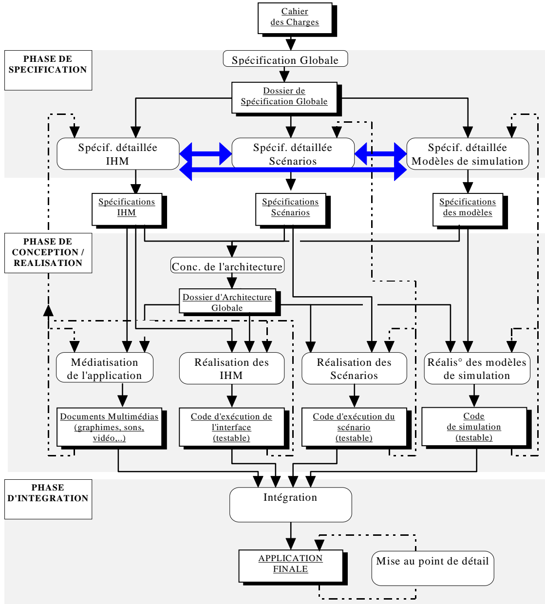
Figure 4-10: Une optimisation provisoire du cycle de développement
