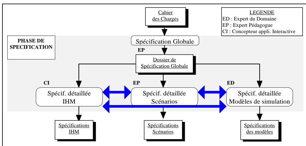
Figure 4-6 : La phase de spécification
