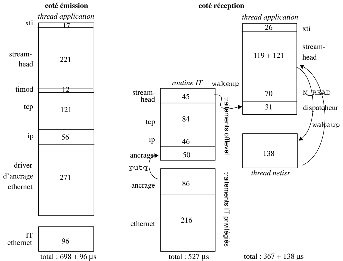
Figure 29: Temps de traitement d'un segment TCP de 1024 octets avec la pile démultiplexée.
