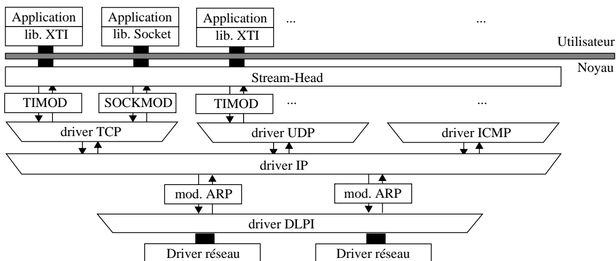
Figure 13: Extrait de la pile TCP/IP sous Streams.
