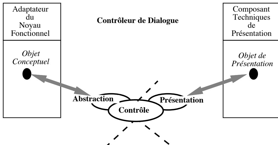
Figure 6.7 : Un agent PAC du Contrôleur de Dialogue.
