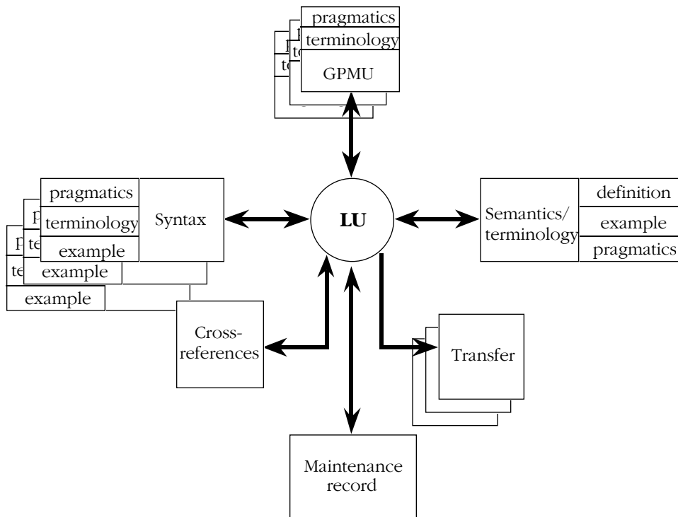
Figure 2.20 : Vue générale d'une LU (Lexical Unit) de MULTILEX
