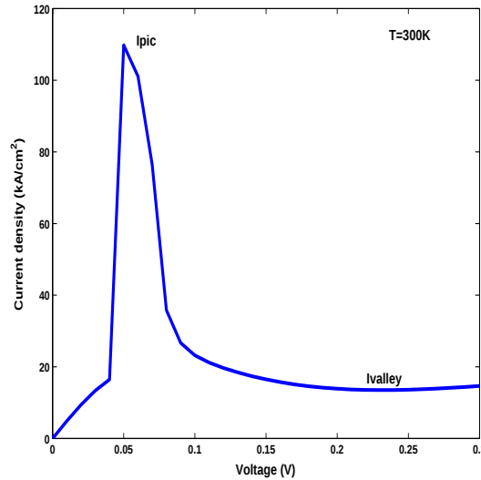
FIG. 8: La courbe caractéristique courant-tension de la diode InAs/AlSb/GaSb/AlSb/InAs à effet tunnel résonnant interbande lorsque T = 300K avec une largeur des barrières AlSb est de 10\text{\AA} et celle du puits GaSb de 30\text{\AA} .
