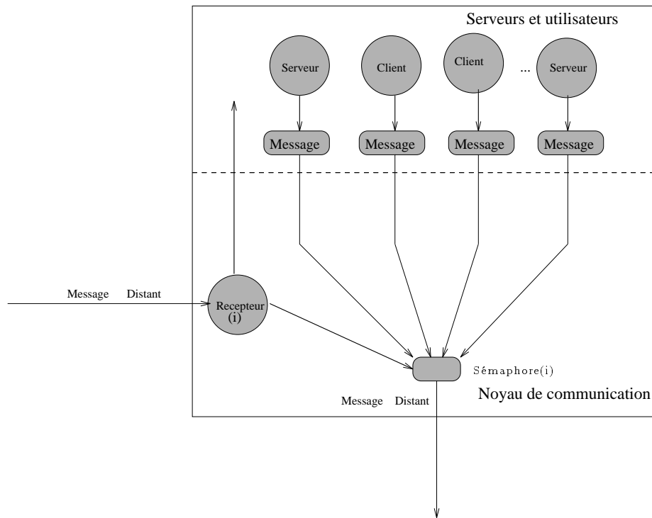
Figure 4.11: Noyau de communication avec plusieurs émetteurs.
