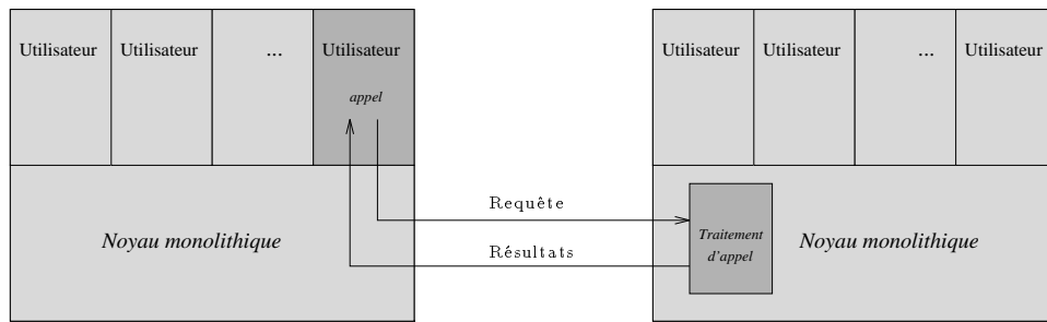
Figure 4.2: Organisation typique d'un noyau monolithique parallèle.
