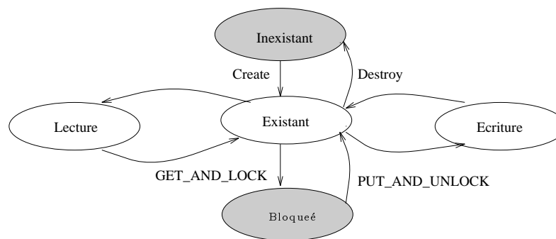
Figure 4.17: Graphe d'état des portes Data.
