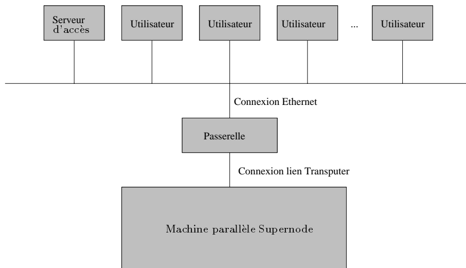
Figure 5.1: Organisation générale de l'environnement matériel.
