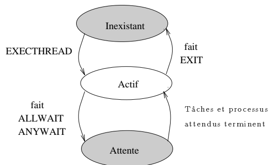
Figure 4.14: Graphe d'état des processus.
