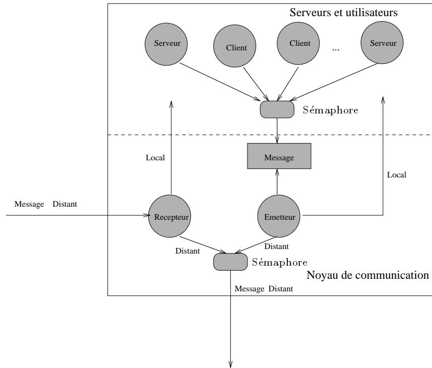
Figure 4.10: Noyau de communication avec un seul émetteur.
