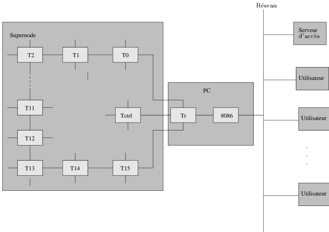
Figure 5.2: La machine Supernode configurée en anneau.
