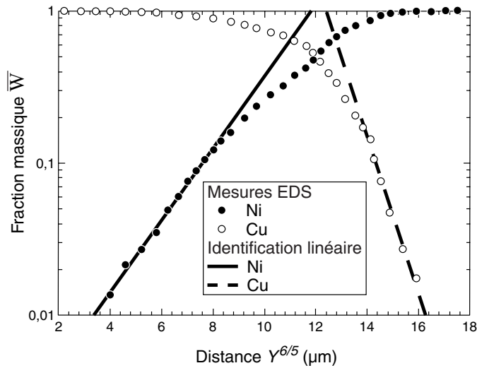
Figure 3.16 – Estimation des coefficients de diffusion aux joints de grains à l'extrémité des profils de concentration. Diffusion à 550°C/24h sur échantillon spécifique (figure 3.11a). Identification linéaire (équation (3.50)) dans le diagramme ( Y^{6/5} , \ln \overline{W}_X ).
