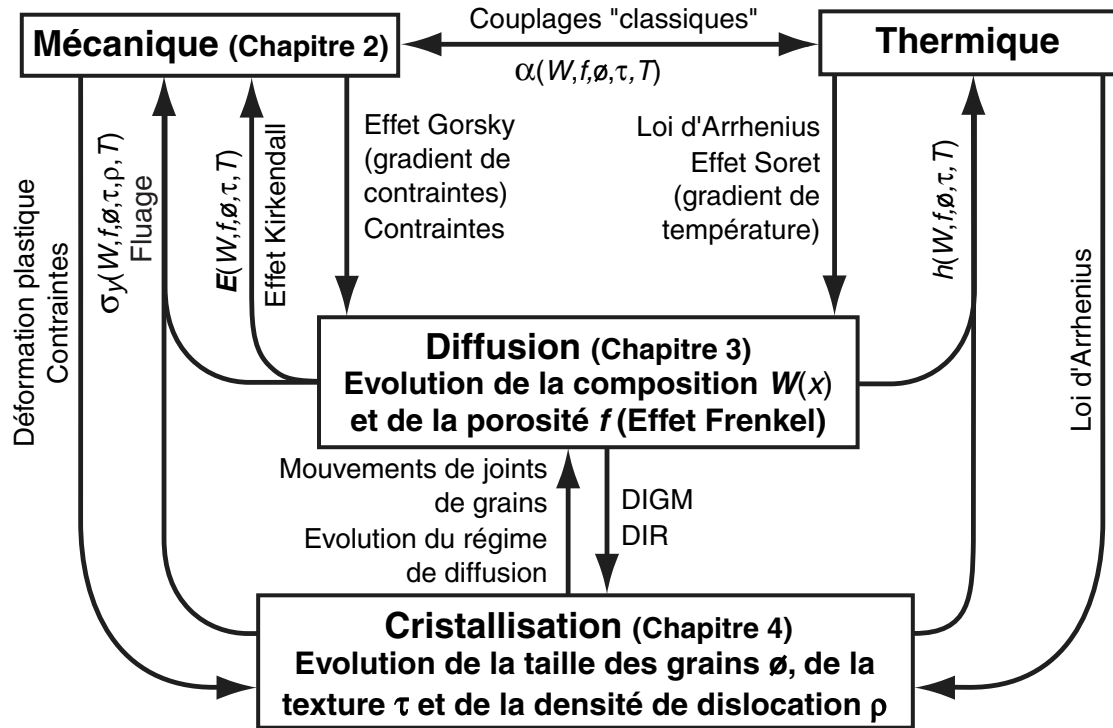
Figure 1.13 – Schéma général des couplages supposés entre les transferts thermiques, le comportement mécanique, la diffusion et la cristallisation et intervenant dans le vieillissement des soufflets obtenus par galvanoplastie dans leur environnement d'utilisation (voir le texte pour plus de détails et le tableau 1.2 [Arnould et al. , 2002b]).
