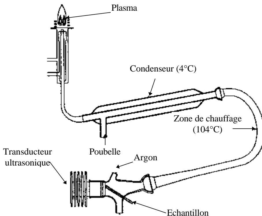
Figure II-8: Schéma du Nébuliseur Meinhart (a) et du nébuleur ultrasonique (b).
