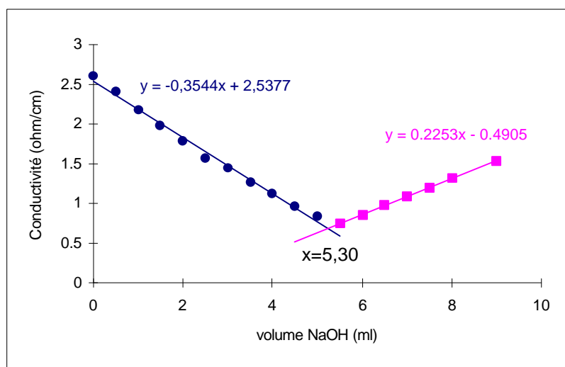
Figure II-4: Droites de dosage conductimétrique de H 2 SO 4 (25 ml) par NaOH (0,1N). Le volume équivalent calculé à l'intersection des droites de dosage est de 5,30 ml, ce qui correspond à une concentration en H + de 1,1 10 -2 mol/L.
