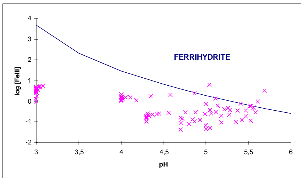
Figure II-13: log des concentrations en fer total trouvées dans nos diverses expériences en fonction du pH. La ligne pleine correspond à la saturation en fer pour la ferrihydrite.
