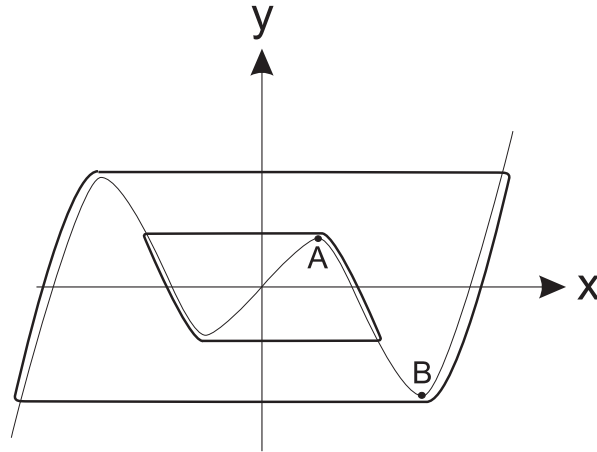
FIG. IV-19 – Forme des cycles limites du système (IV.2-11) quand \epsilon \rightarrow \infty . Les cycles limites ne peuvent couper la courbe y = F(x) que dans un seul sens car celle-ci est semi-perméable.
