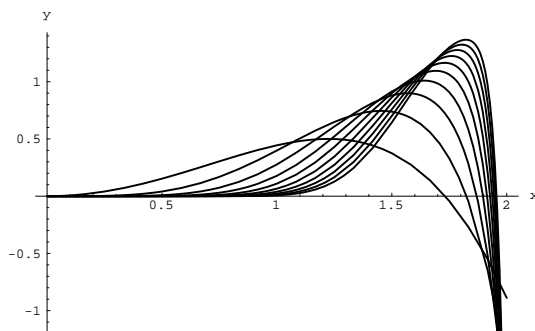
FIG. II-18 – Courbes y = \frac{R_n}{k_n} pour 2 \leq n \leq 20 pour le système (II.2-3) avec \epsilon = 1 . La courbe avec n = 20 est celle qui a son maximum le plus haut.
