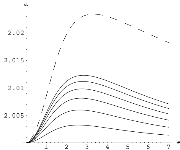
FIG. III-6 – Courbes \hat{R}_n(a, \epsilon) = 0 pour n = 2 à n = 16 . La courbe en pointillé est calculée par intégration numérique des équations (III.3-1). L'axe horizontal est a = 2 .
