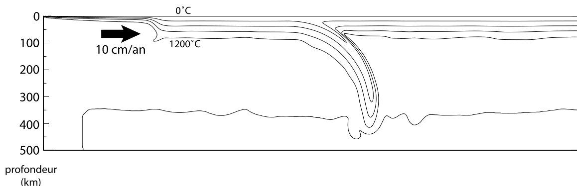
Figure 1.3 - Structures thermiques des plaques, subduite et chevauchante, obtenues en modélisation numérique (document de Diane Arcay). On impose une convergence de 10 cm/an aux deux plaques océaniques. Les isothermes sont tous les 300°C.
