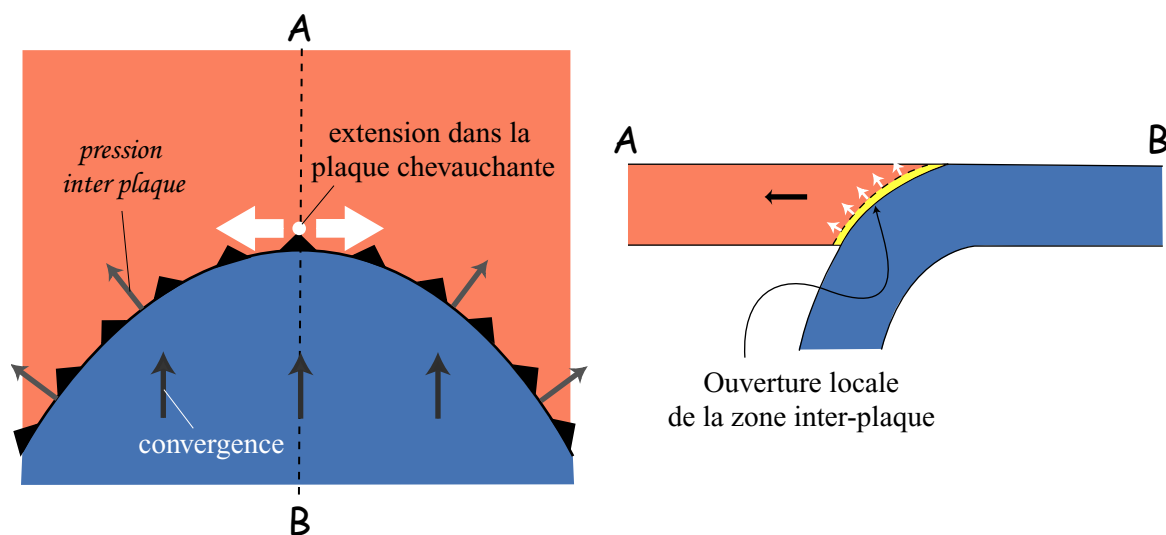
Figure 4.1 – Schéma de l'effet d'une subduction convexe
