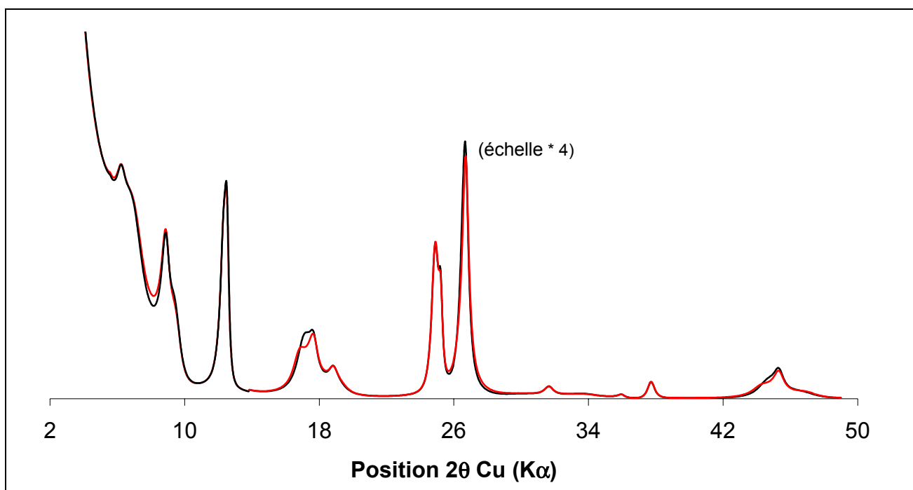
Figure 5.23 : Comparaison entre la simulation obtenue pour l'échantillon E, avec le modèle à une phase en noir (voir texte), et le modèle à deux phases en rouge.
