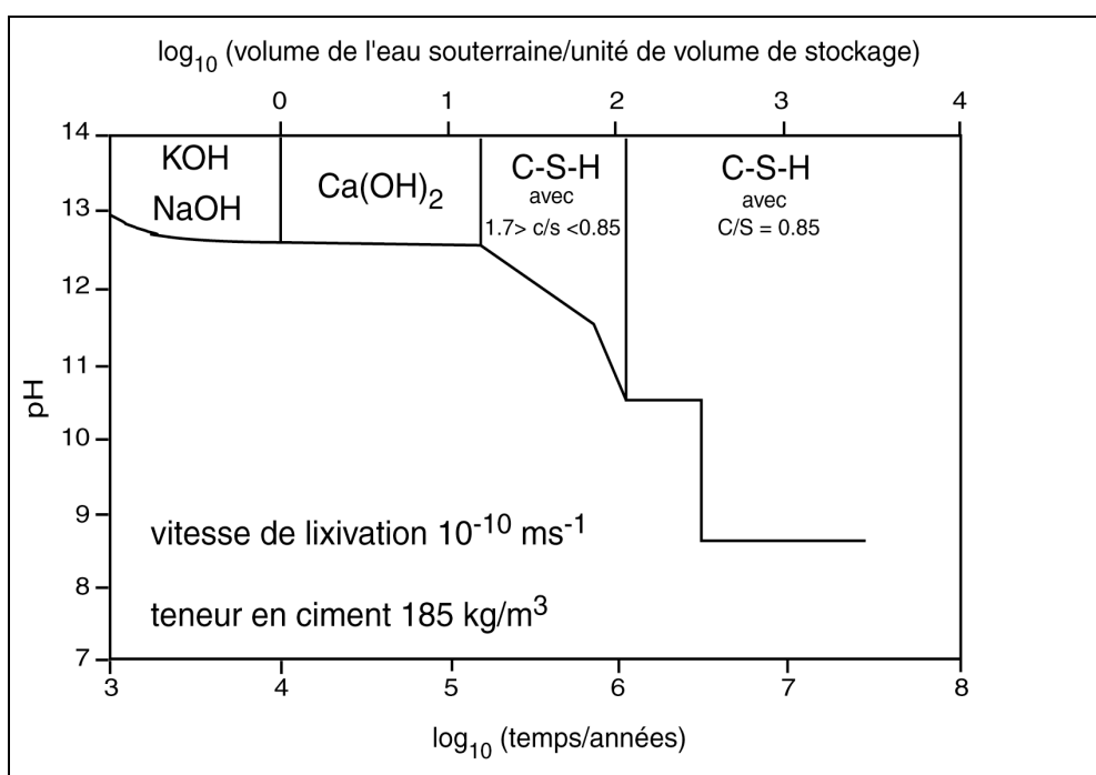
Figure 7.1: Estimation du temps de décomposition du ciment Portland en fonction du pH de l'eau contenue dans ses pores. Modèle sphérique de stockage de 20 m de rayon contenant 185 kg/m 3 de ciment Portland situé dans un environnement à faible flux souterrain (d'après Atkinson, 1985). Jusqu'à 10 4 ans, la chimie du système est contrôlée par les hydroxydes de sodium et de potassium du ciment, jusqu'à 10 5 ans elle l'est par
