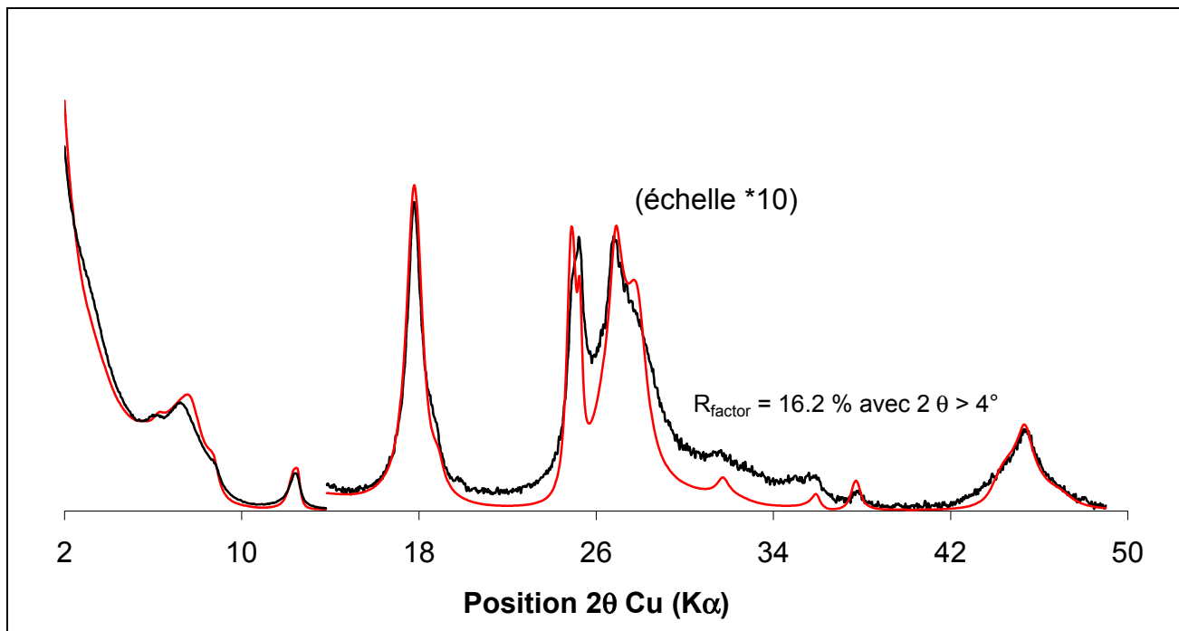
Figure 5.20 : Echantillon D saturé Ca+AD. En noir, le diffractogramme expérimental, en rouge, celui simulé en utilisant N=15 pour Int_2 (voir texte).
