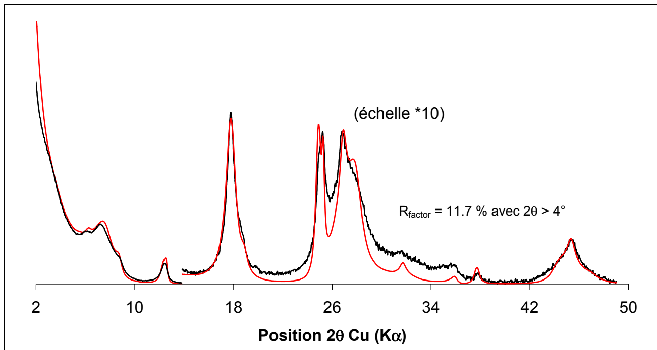
Figure 5.19 : Echantillon D saturé Ca+AD. En noir, le diffractogramme expérimental, en rouge, celui simulé en utilisant N=8 pour \text{Int}_2 (voir texte).
