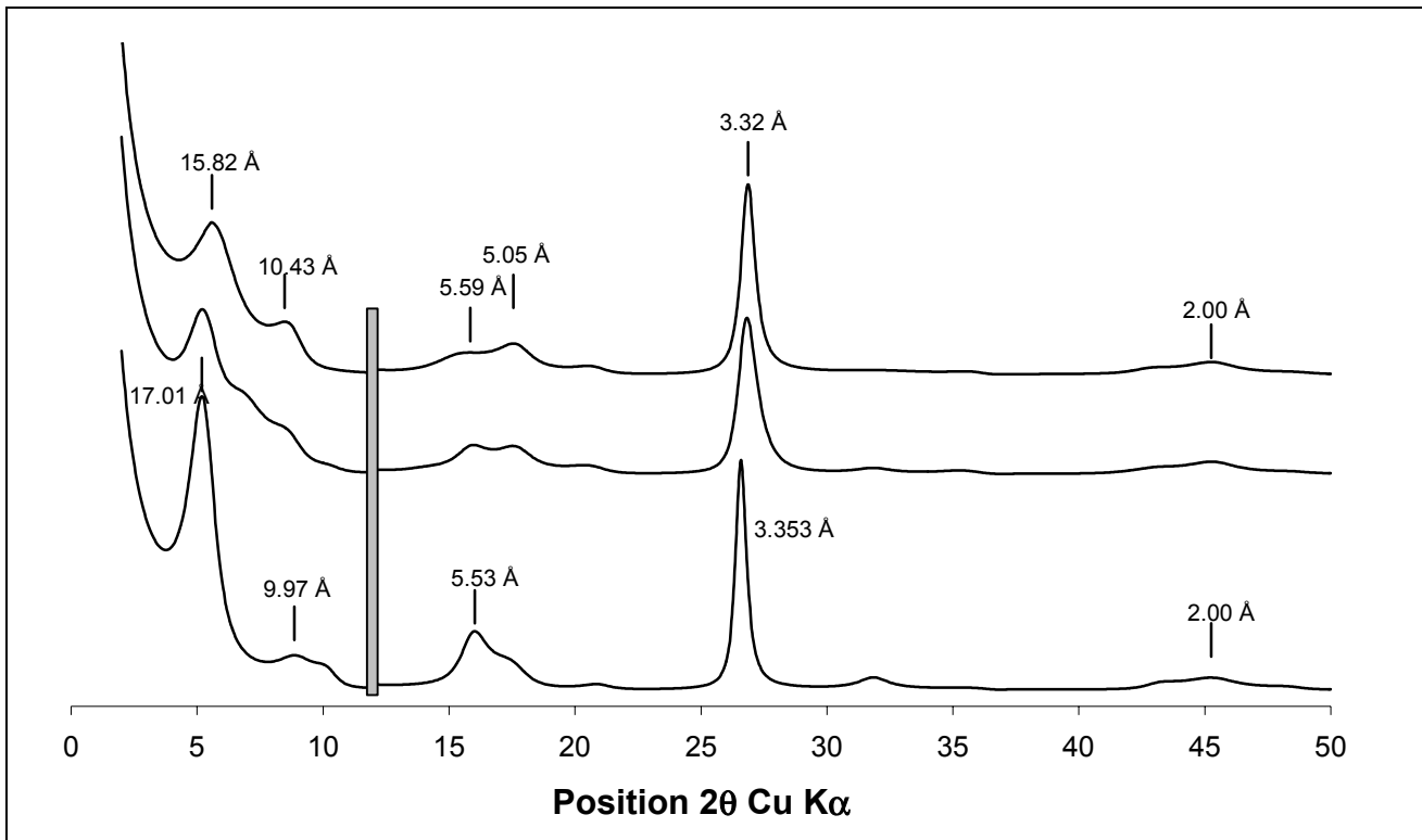
Figure 2.17 : R = 1 ségrégation. En haut, le modèle à trois composants correspondant au cas numéro 1 (voir texte), au milieu, le cas numéro 2, en bas, l'interstratifié à deux composants. La partie grisée indique un changement d'échelle (*3).
