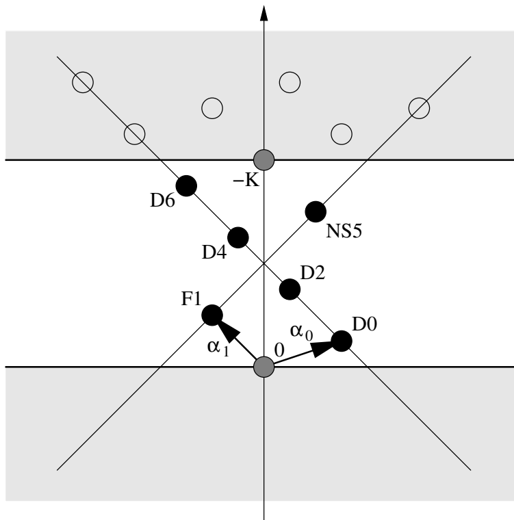
FIG. 2.2 – Diviseurs de degré et genre positifs de la surface \mathbb{P}_1^2 et objets BPS correspondants dans la théorie IIA.
