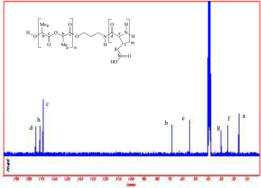
Figure 6 Spectre RMN 13 C du copolymère à blocs PLLA-b-PGAdans le DMSO d6
