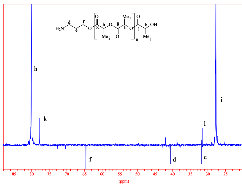
Figure 12 Spectre RMN ^{13}\text{C} séquence DEPT du PLLA-NH _2 dans le CDCl _3
