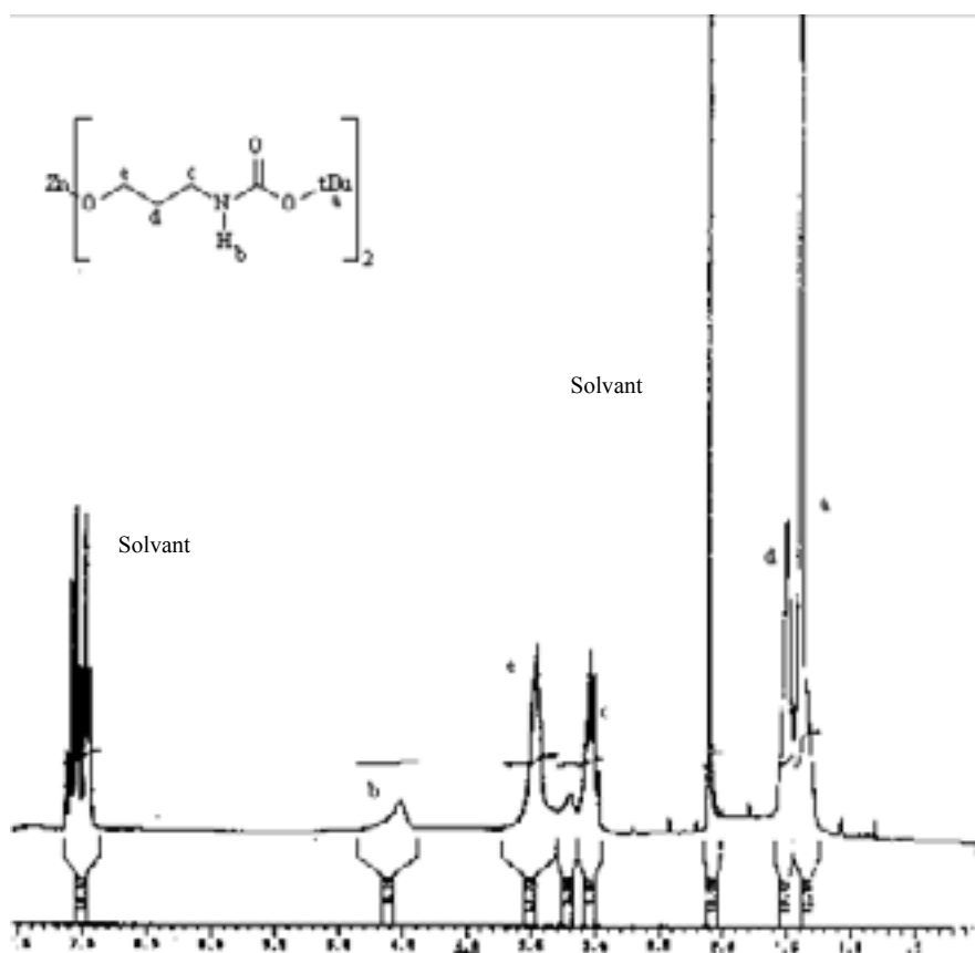
Figure 2 Spectre RMN ^1\text{H} du N-(terbutylcarbamate)propanolate de zinc [2] dans le toluène d8
