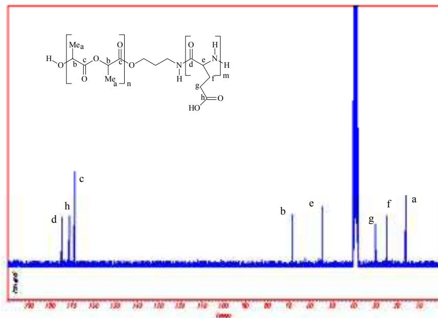
Figure 6 Spectre RMN ^{13}\text{C} du copolymère à blocs PLLA-b-PGA dans le \text{DMSO-d}_6
