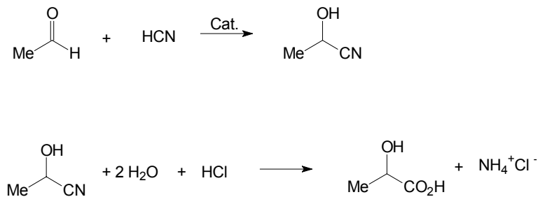
Figure 2 Synthèse de l'acide lactique
