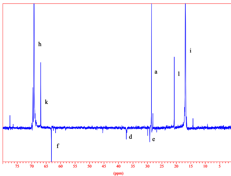
Figure 8 Spectre RMN ^{13}\text{C} séquence DEPT du PLLA dans le \text{CDCl}_3
