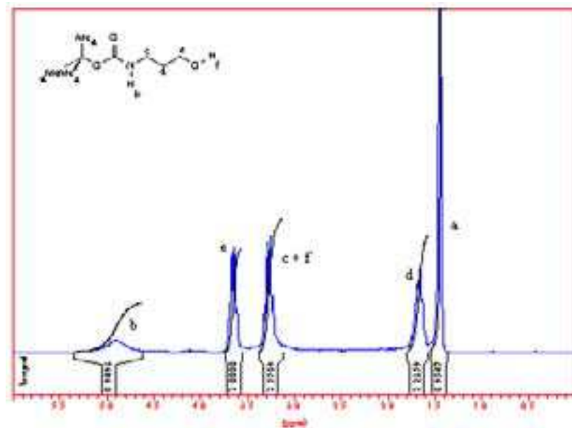
Figure 1 Spectre RMN ^1\text{H} du N-(terbutylcarbamate)propanolate [1] dans le \text{CDCl}_3
