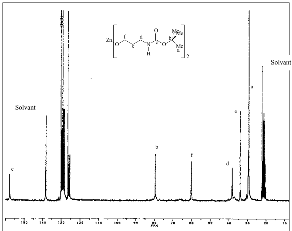
Figure 3 Spectre RMN ^{13}\text{C} du N-(terbutylcarbamate)propanolate de zinc [2] dans le toluène d8
