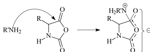
Schéma 22 Zwitterion de résonance formé lors de l'attaque du NCA par une amine primaire
