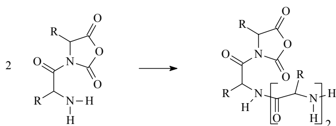
Schéma 29 3 ème cas de propagation selon le mécanisme du monomère activé
