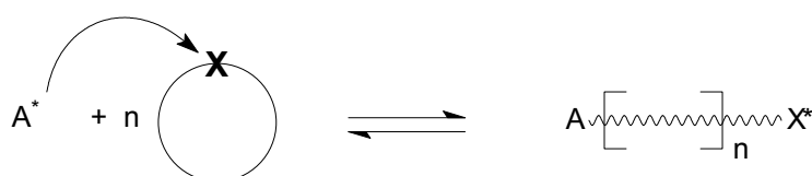
Schéma 5 Schéma général d'une polymérisation par ouverture de cycle
