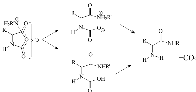
Schéma 23 Décarboxylation du zwitterion
