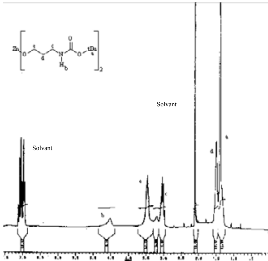
Figure 2 Spectre RMN ^1\text{H} du N-(terbutylcarbamate)propanolate de zinc [2] dans le toluène d8
