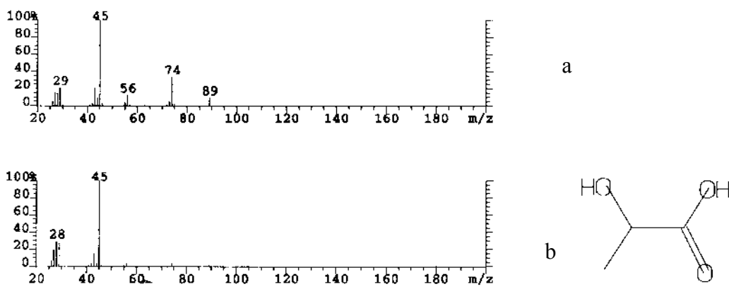
Figure 5 Spectrométrie de masse du 2 ème pic de la Figure 3
