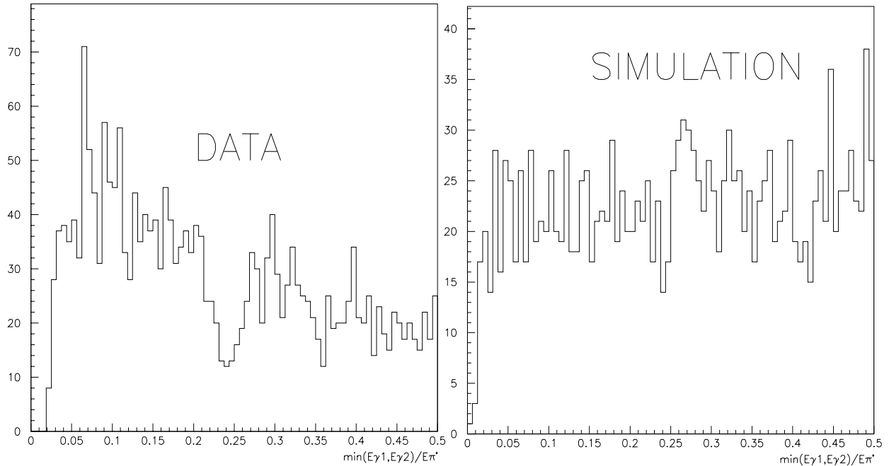
FIG. 5.22 – Distribution du rapport \frac{\min(E_{\gamma 1}, E_{\gamma 2})}{E_{\pi^0}} dans le cas des données expérimentales. FIG. 5.23 – Distribution du rapport \frac{\min(E_{\gamma 1}, E_{\gamma 2})}{E_{\pi^0}} dans le cas de la simulation.
