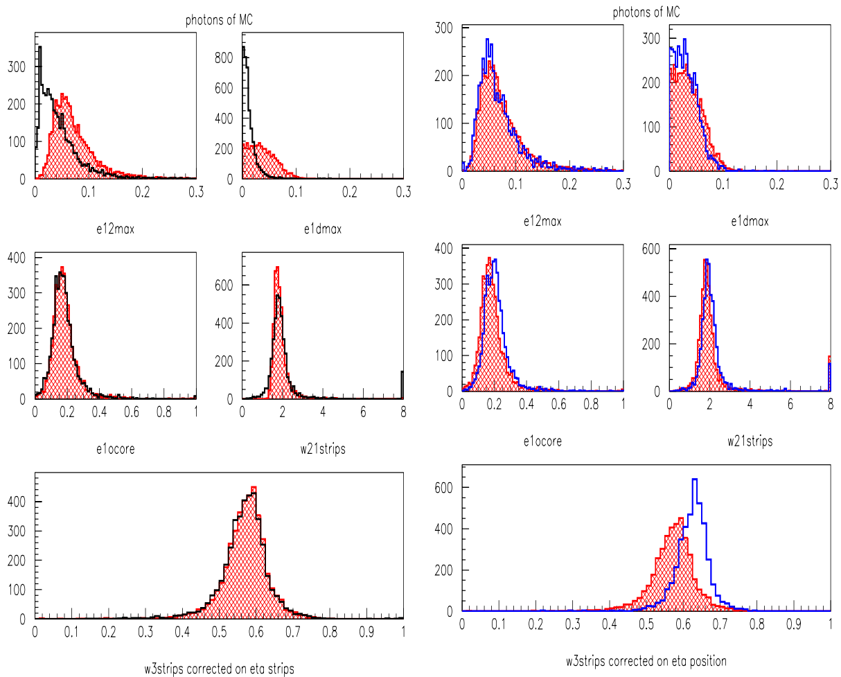
FIG. 5.11 – Variables utilisées pour calculer le facteur de rejet \gamma/\pi^0 dans le cas de la simulation en introduisant l'effet de la diaphonie entre cellules (histogrammes hachés) et sans diaphonie (histogrammes vides) à 0 < Pt_\gamma < 50\text{GeV}/c , \eta = 28 et \phi = 10 . Dans les 2 cas, nous avons pris en compte le bruit électronique.
