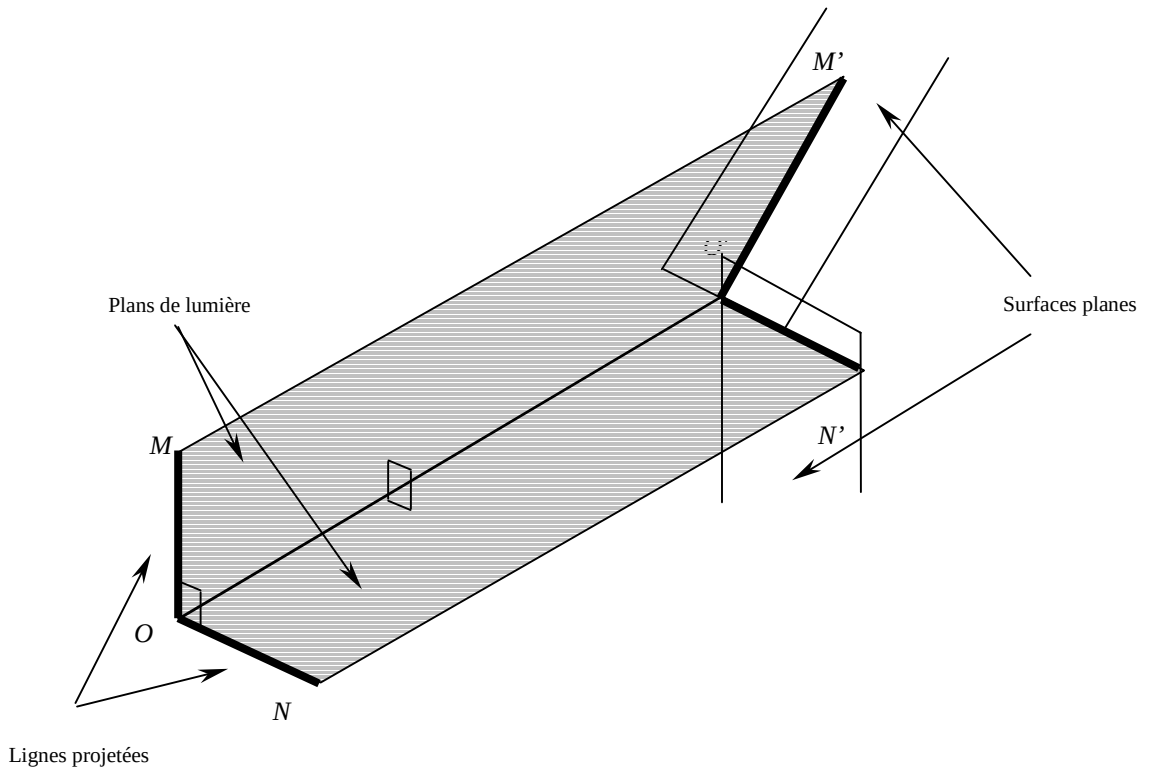
Figure 59. Contraintes d'orthogonalité
