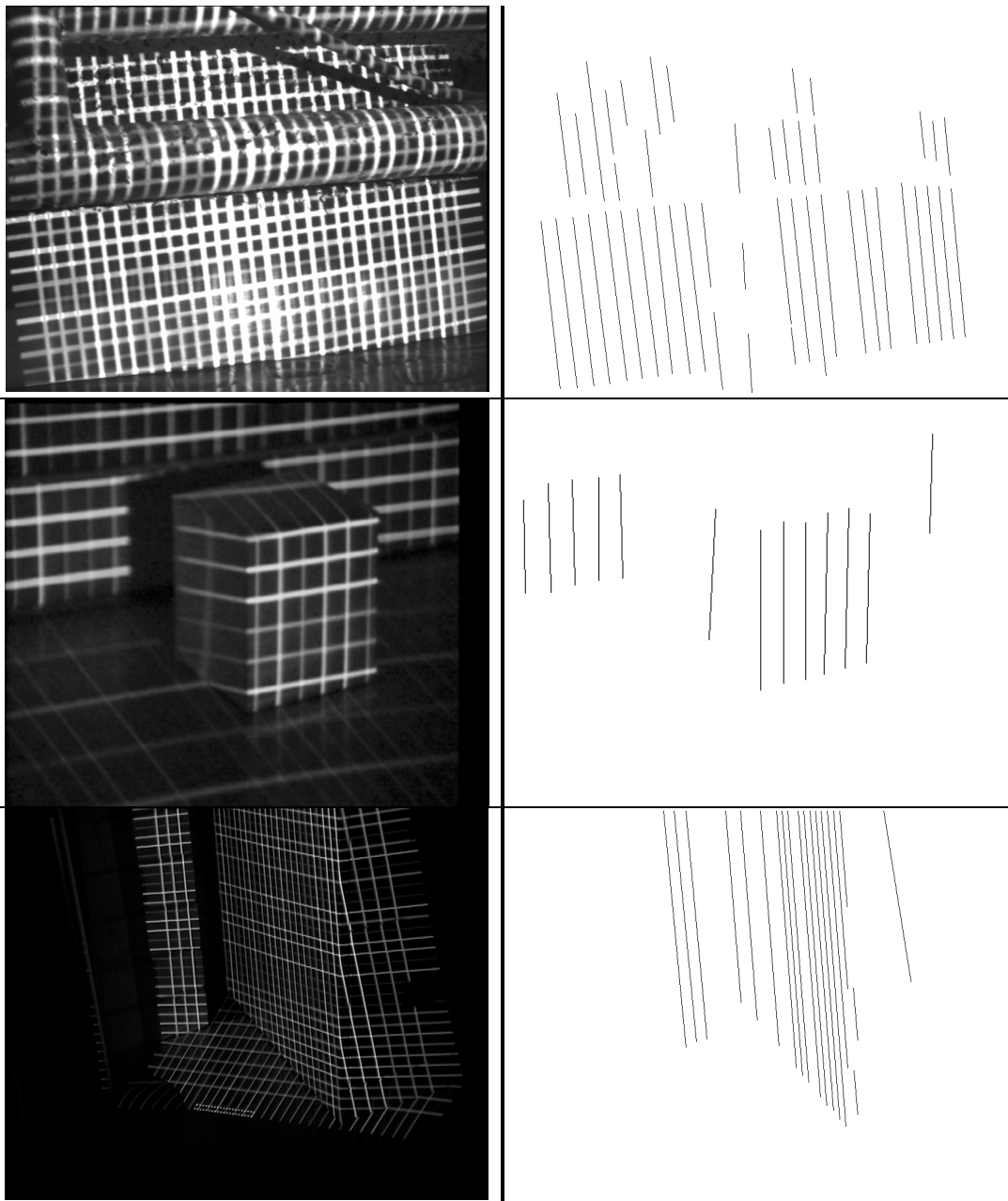
Figure 70. Détection des obstacles. A gauche : la scène. A droite : les obstacles détectés.
