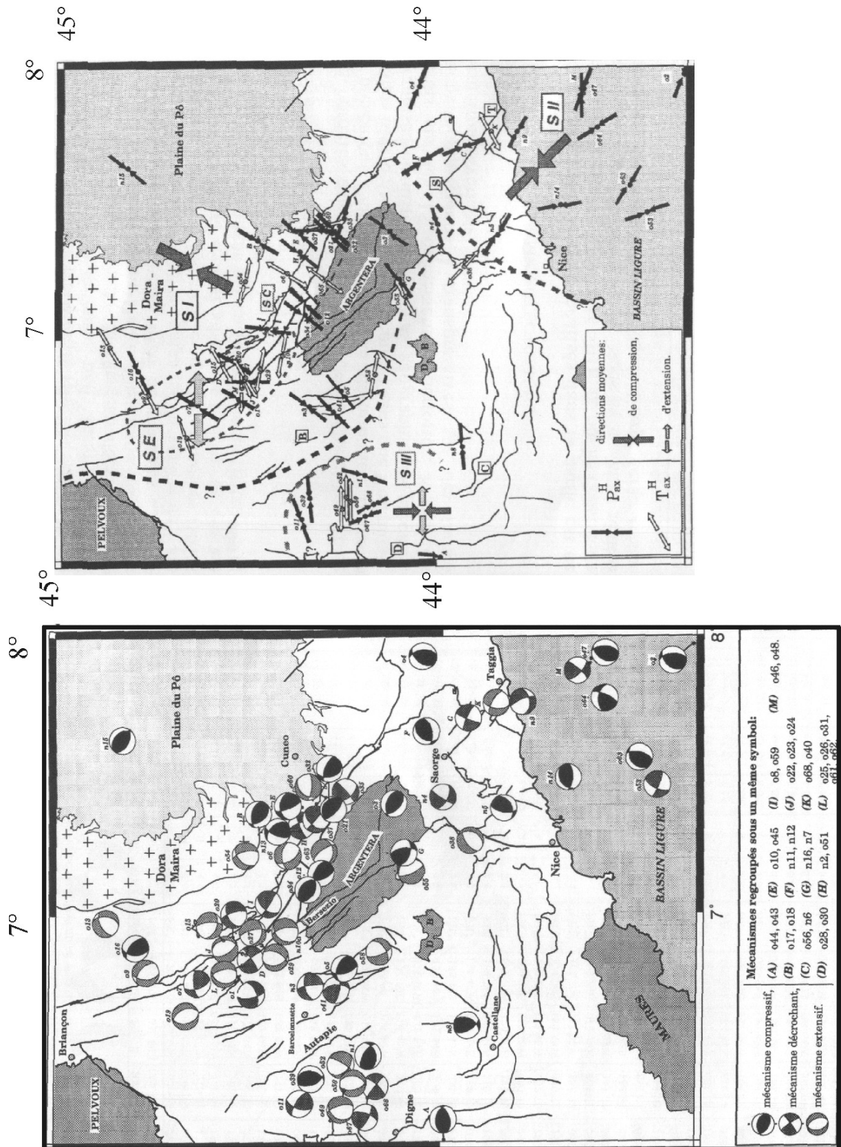
Figure 21 : Répartition des mécanismes au foyer dans la région Argentera et le bassin Ligure (à gauche) et des axes de déformation déduits de ces mécanismes (P et T) (à droite) (d'après Madeddu et al. , 1996).
