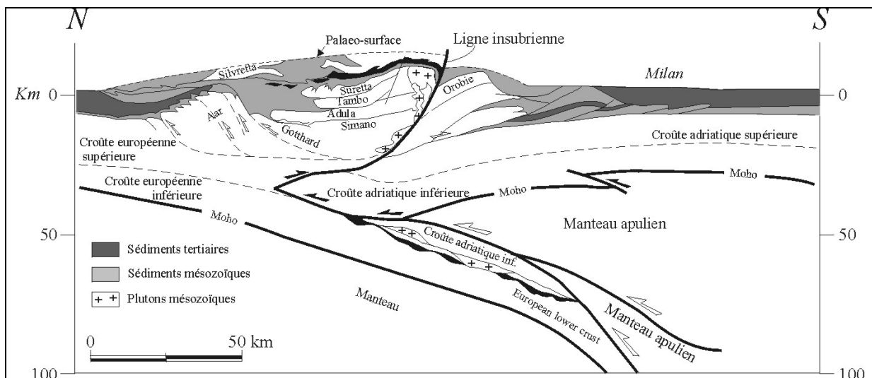
Figure 10 : Interprétation structurale du profil sismique réflexion profonde dans les Alpes centrales (d'après Pfiffner et al. , 1997).
