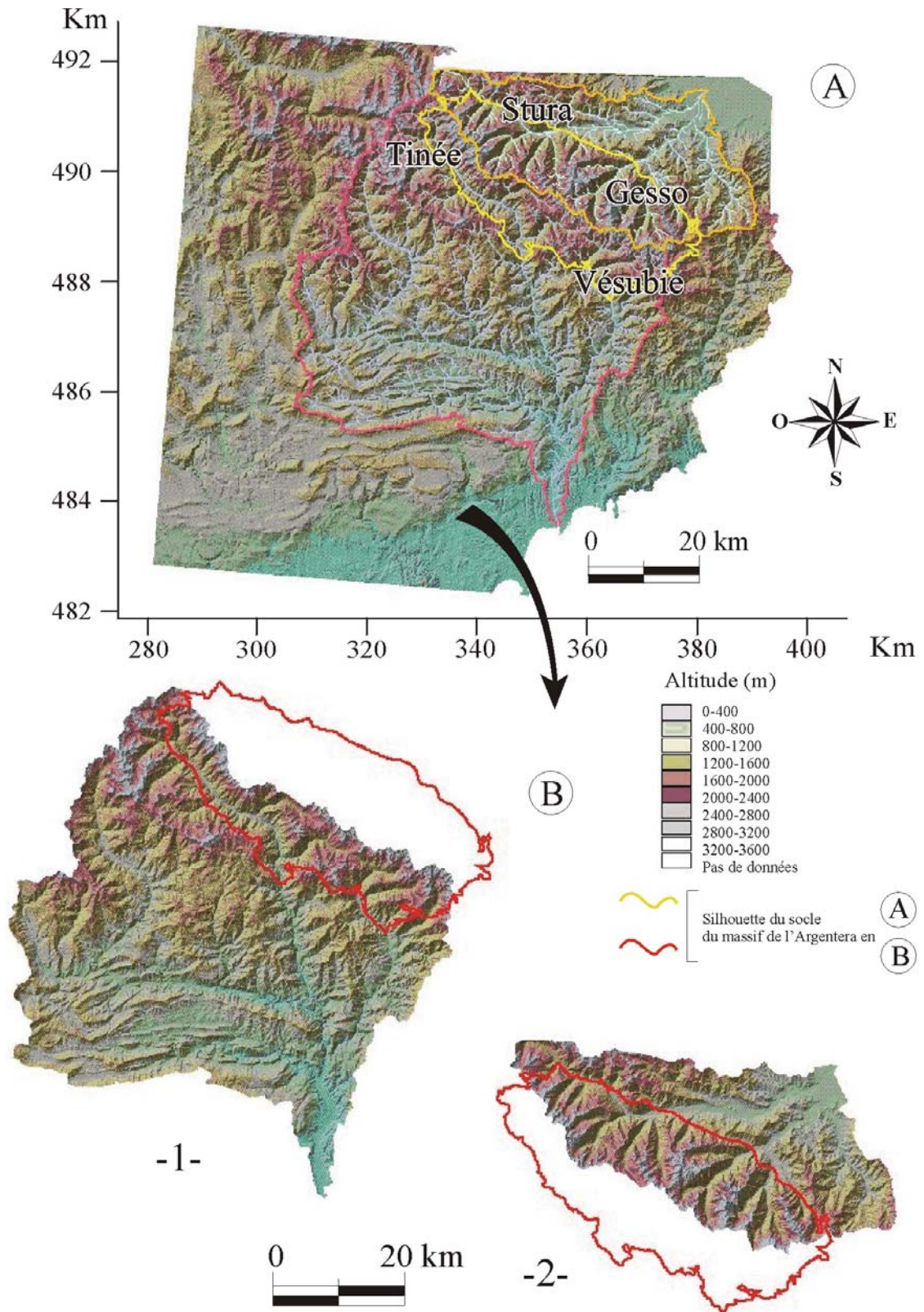
Figure 68 : Géométrie des bassins versants sur le socle de l'Argentera.
