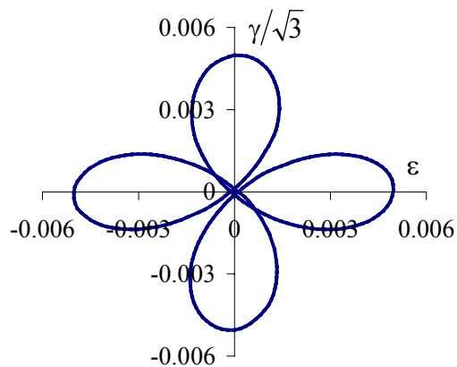
Trajet dans le plan (\epsilon, \gamma/\sqrt{3})
