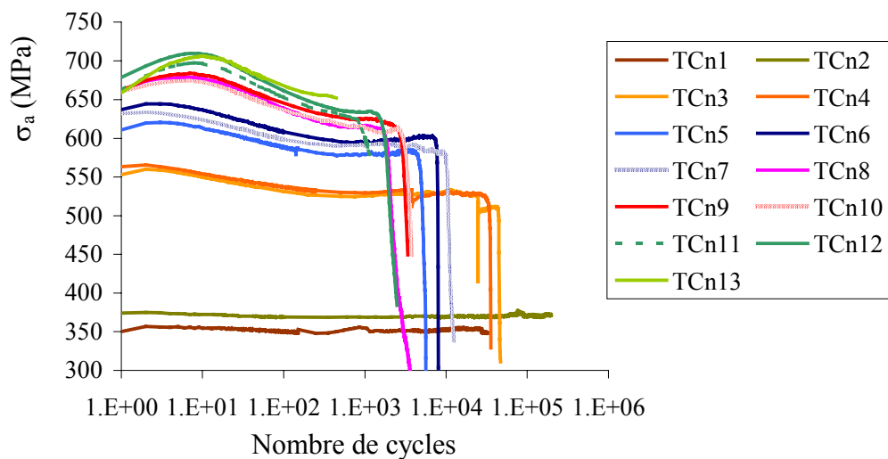
Figure II-13 : Courbes de durcissement/adoucissement cyclique
