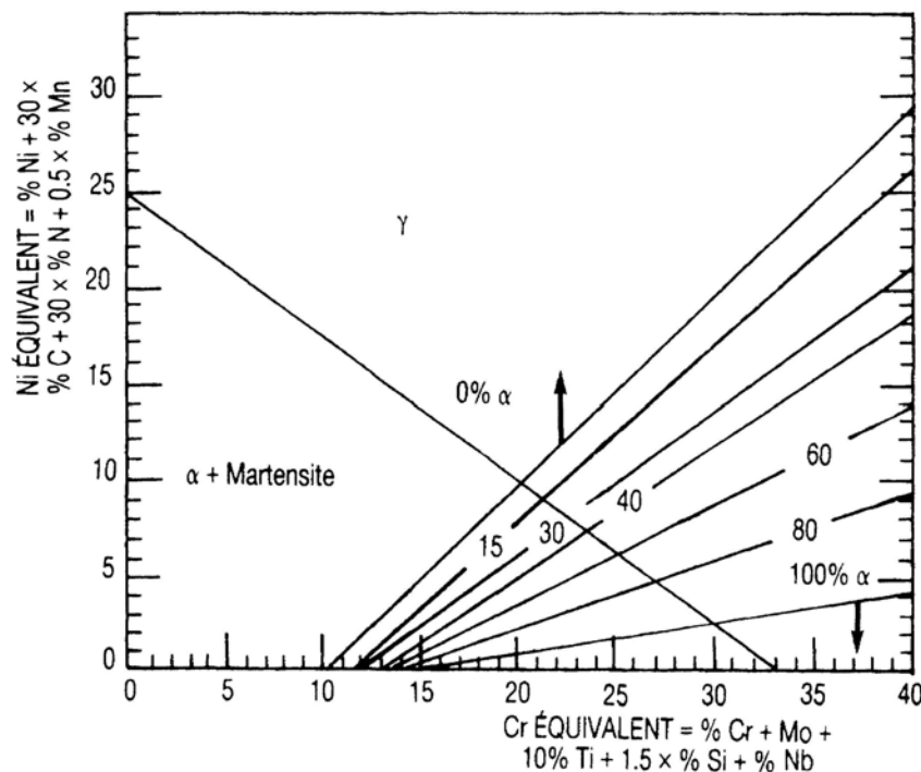
Figure I-3 : Diagramme de Schaeffler pour des aciers inoxydables corroyés, modifié pour tenir compte de l'influence de l'azote cité par [Lacombe 1990]
