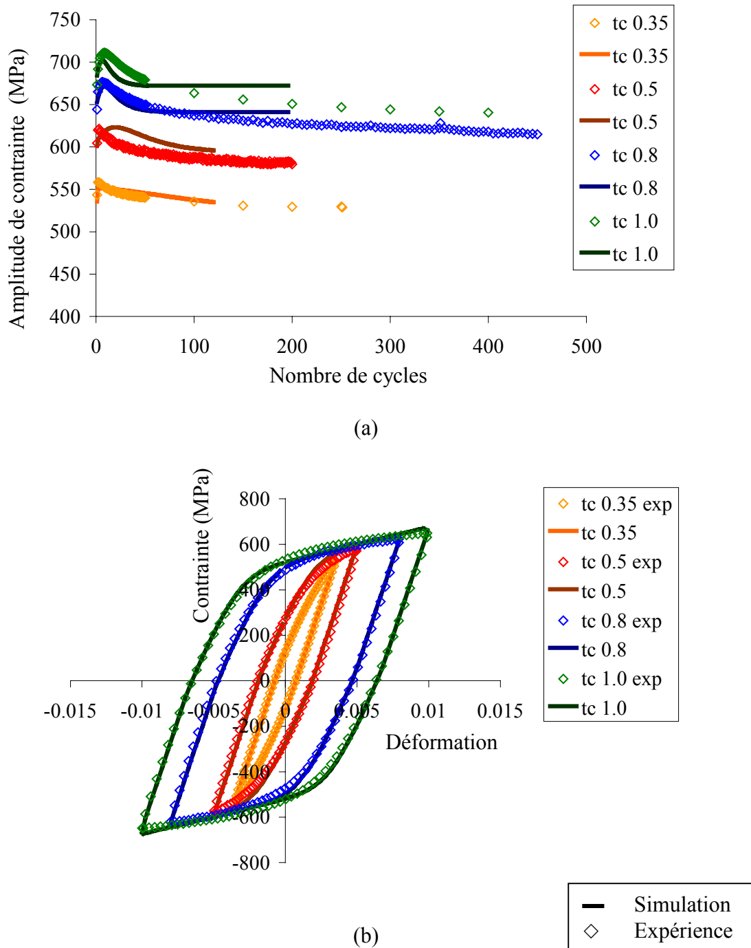
Figure IV-4 : Comparaison des résultats du modèle CINL avec les résultats expérimentaux ayant servi à l'identifier (identification B)
