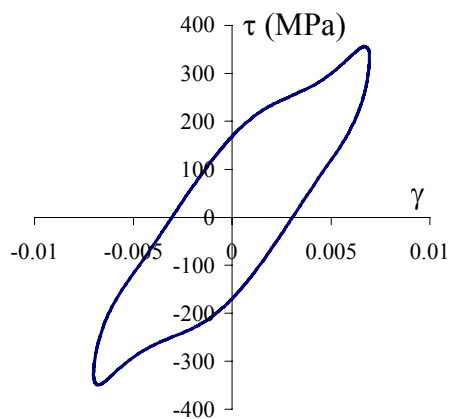
Boucle d'hystérésis dans la direction de cisaillement
