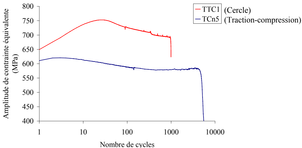
Figure II-24 : Courbes de durcissement/adoucissement cyclique pour les trajets cercle et traction-compression à 0,5% d'amplitude de déformation équivalente
