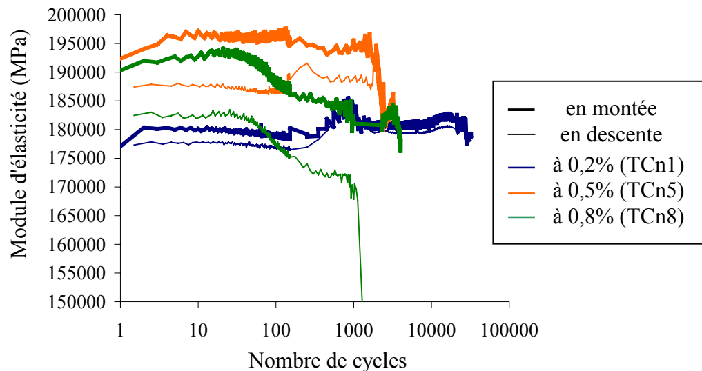
Figure II-18 : Evolution du module d'élasticité pour 3 niveaux d'amplitude de déformation imposée au cours des cycles de traction-compression
