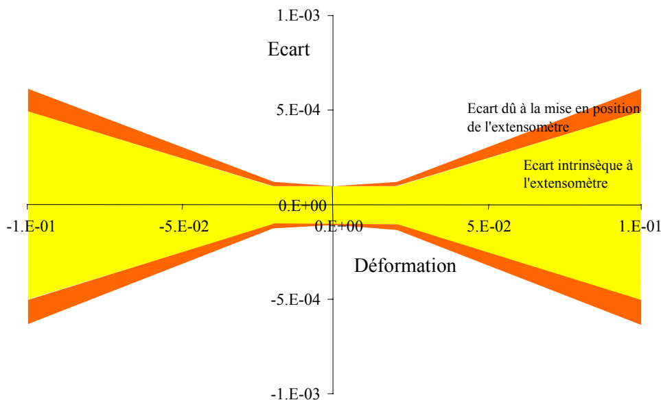
Figure B-2 : Ecarts dans la mesure de la déformation axiale
