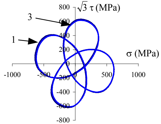
Réponse dans le plan (\sigma, \sqrt{3} \tau)
