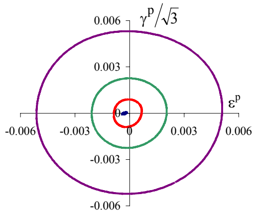
Réponses dans le plan (\epsilon^p, \gamma^p/\sqrt{3})
