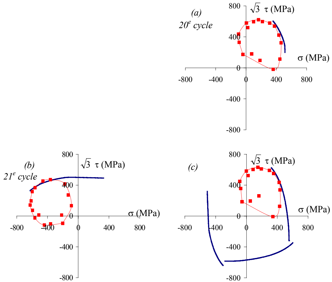
Figure III-30 : Surfaces de plasticité mesurées sous un chargement carré (Surf4) à 0,5 % d'amplitude à divers changements de direction pendant les 20^{\text{e}} et 21^{\text{e}} cycles (dernier sommet du 20^{\text{e}} cycle, premier et dernier sommet du 21^{\text{e}} cycle)
