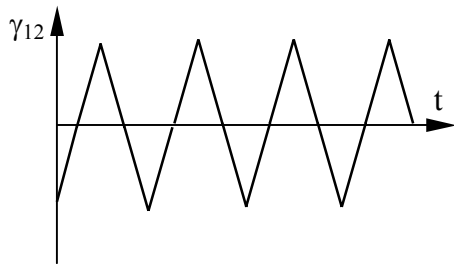
chargeement périodique triangulaire
