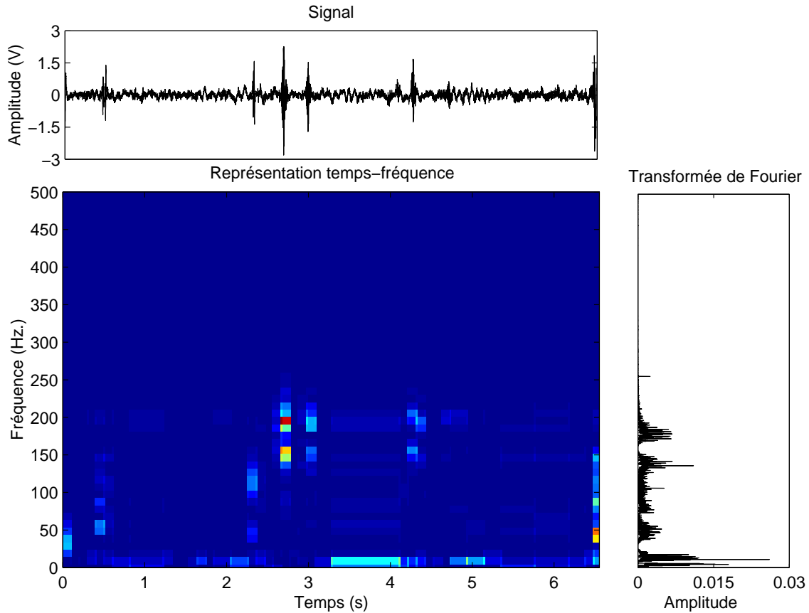
FIG. 3.3 – Représentation temps-fréquence
