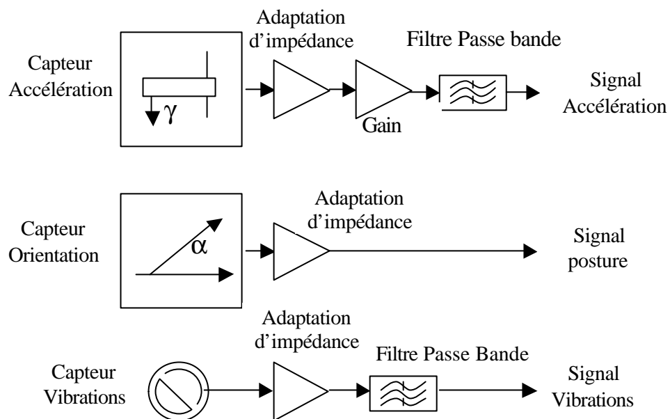
Figure 25 : synoptique de l'actimètre : conditionnement des capteurs.
