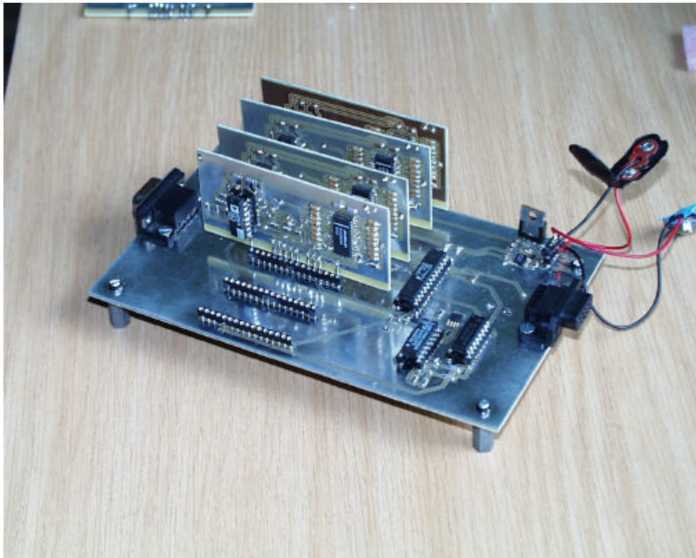
Figure 31 : carte d'acquisition principale avec quatre modules de conditionnement.
