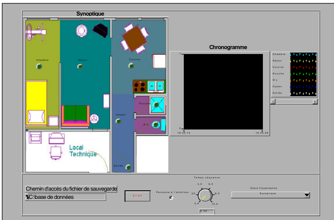
Figure 13 : premier logiciel de supervision.
