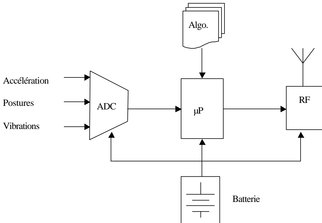
Figure 26 : synoptique de l'actimètre : partie traitement des information.
