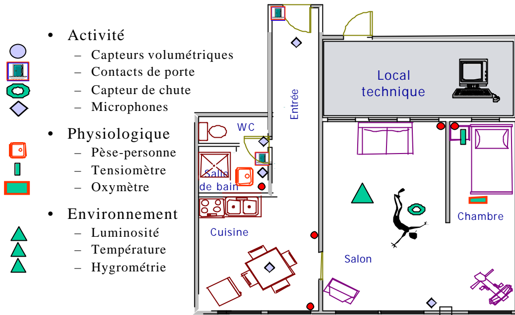
Figure 16 : position des capteurs dans l'habitat.
