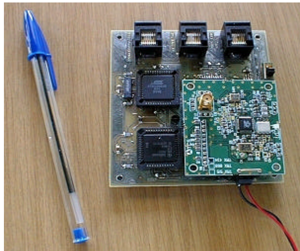
Figure 12 : photo du prototype.
