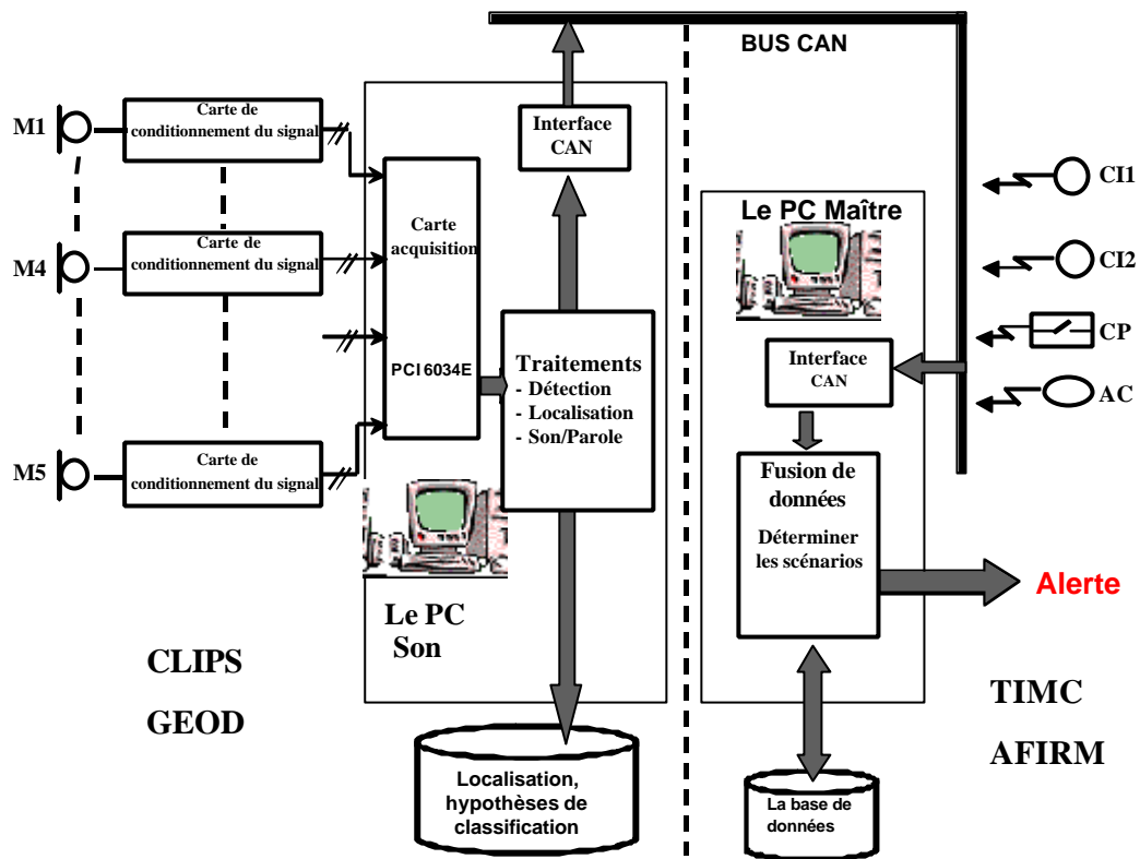
Figure 88 : communication entre le PC maître et le PC esclave.
