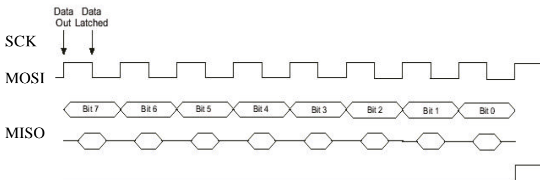
Figure 72 : chronogramme de fonctionnement de la liaison SPI.
