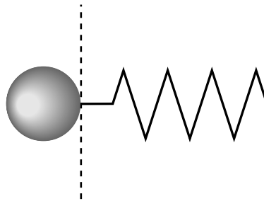
Figure I.1: Schéma d'une molécule amphiphile
