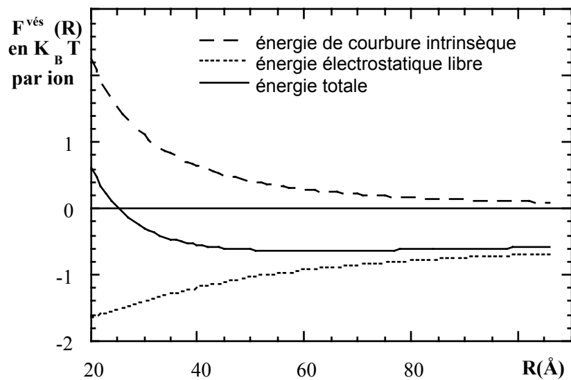
Figure V.13: Énergie libre en fonction du rayon moyen pour les paramètres \Phi=1.2\% , \Omega=0.60 et \Gamma=5.0\% en pointillés: énergie libre de la double couche électrique en traits: contribution d'élasticité de courbure intrinsèque en ligne continue: énergie totale (somme)
