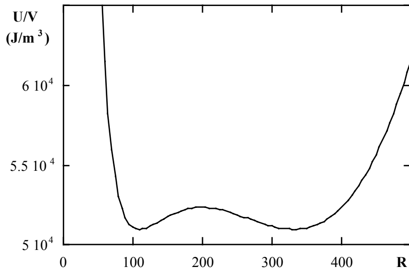
Figure D.2: Energie électrostatique par unité de volume en fonction du rayon moyen des vésicules (selon l'équation (D2)) pour \Phi=8.3\% , \Gamma=3.55\% , \tilde{\kappa}=5.6 k_B T
