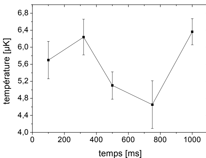
FIG. 3.13 – Evolution de la température suivant la direction ( Ox ) entre 100 ms et 1 s.
