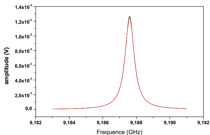
FIG. 6.5 – Fréquence de résonance de la cavité sphérique polie (Signal en réflexion). On utilise une antenne de 3 mm de long, et une fente de couplage de 1 \times 6\text{ mm} (couplage non optimum). La fréquence de résonance est désaccordée de 5,03 MHz de la résonance hyperfine du Cs.
