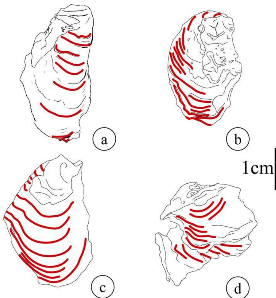
Figure 5-10 : Localisation des prélèvements effectués sur les Neopycnodonte cochlear actuels pour l'analyse des isotopes stables du Carbone et de l'Oxygène (en rouge): a) coquille prélevées sur la station UNEP7; IGR 25560 ; b, c et d) coquilles np1, np2 et np3 prélevées sur la station KC32; IGR 25561, IGR 25512 et IGR 25510.
