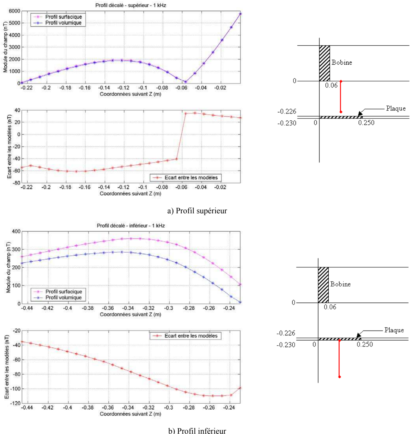
Figure 78 : Module de la composante suivant Z du champ magnétique le long du second profil. Confrontation entre les résultats du modèle numérique ( en bleu ) et du modèle analytique local ( en violet ). On présente sur le graphe inférieur l'écart entre les valeurs des deux modèles. On distingue en a) les valeurs du module le long du profil supérieur et en b) les valeurs obtenues le long du profil inférieur.
