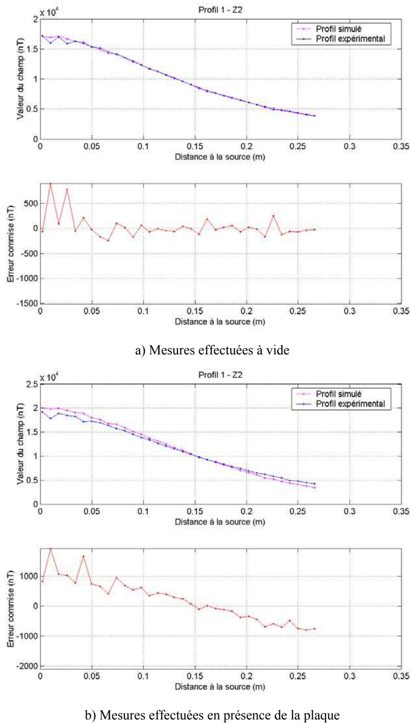
Figure 67 : Composante suivant Z du champ magnétique à l'altitude Z2 le long du profil d'axe Oz, axe de la bobine. Le bord de plaque se situe en x = 0.25 m. Confrontation entre les résultats du modèle éléments finis (en rouge) et les mesures expérimentales (en bleu). On présente sur le graphe inférieur l'écart entre les valeurs expérimentales et simulées. On distingue en a) les mesures effectuées à vide et en b) celles effectuées en présence de la plaque conductrice.
