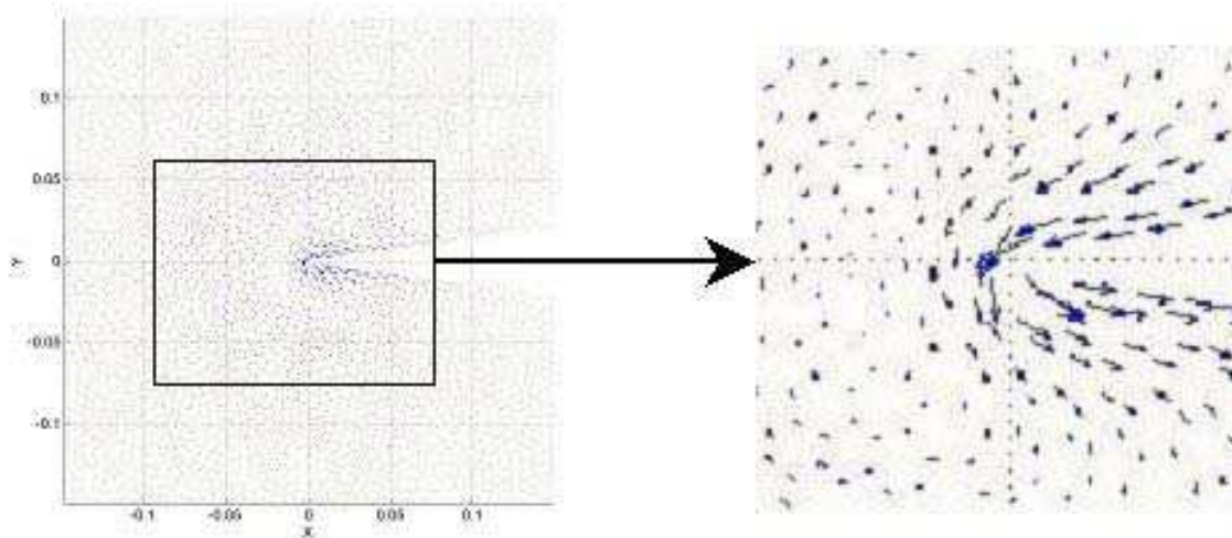
Figure 40 : Représentation vectorielle des courants de Foucault
