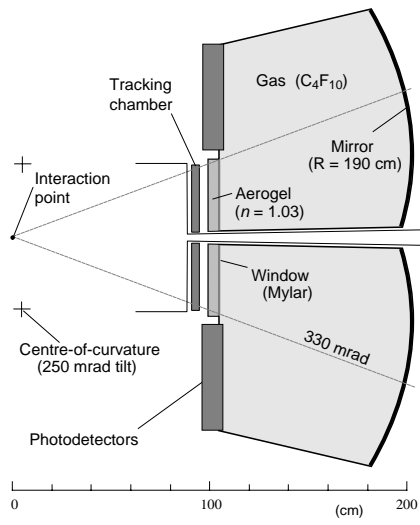
FIG. 6.5: Schéma du détecteur RICH 1.
