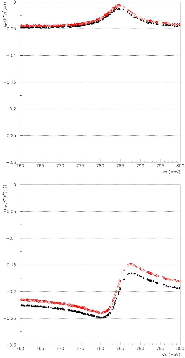
FIG. 5.11: Paramètre de violation de CP , a_{CP}(m) , en fonction de la masse invariante du système (\pi^+\pi^-) au voisinage du \omega pour le canal B^+ \rightarrow K^{*+}\rho^0(\omega) . Les paramètres utilisés sont, en haut (en bas), q^2/m_b^2 = 0.3(0.5) , N_c^{eff} = 2.84(2.82) , \rho = 0.229 , \eta = 0.325 . Les triangles pleins correspondent au modèle BSW des facteurs de forme et les cercles vides au modèle GH.
