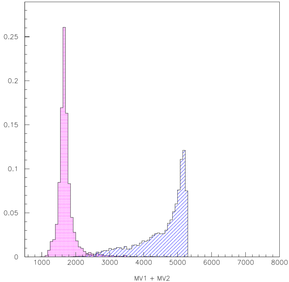
FIG. 7.12: Somme des masses (en MeV) des combinaisons K^+\pi^- et \pi^+\pi^- obtenues à partir des quatre particules provenant d'un B^0 . La distribution en plein correspond aux particules correctement associées, celle en hachuré aux particules mal associées. Ces distributions proviennent de la modélisation Monte-Carlo présentée aux chapitres 4 et 5.
