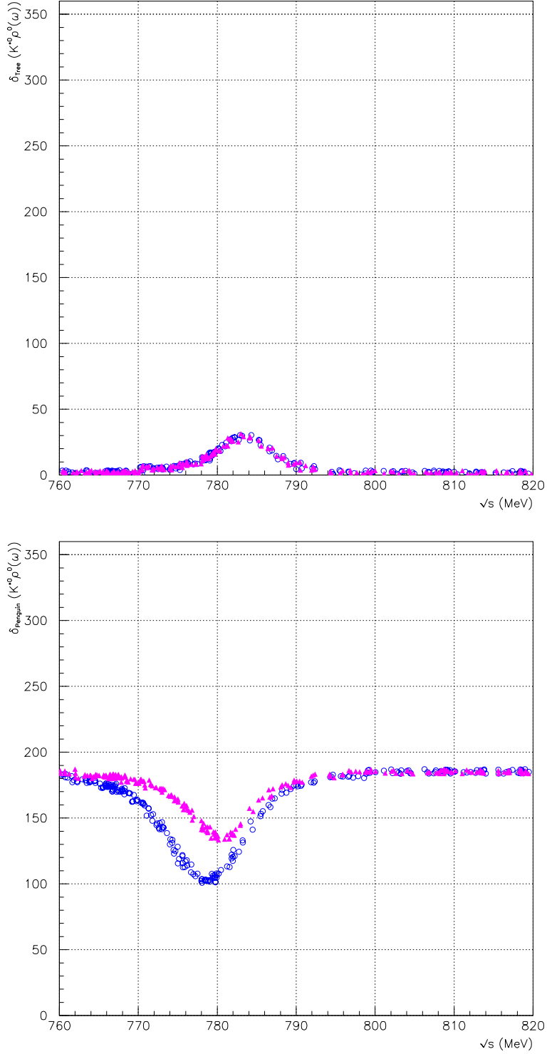
FIG. 5.15: Angles \delta_{Tree} du diagramme Tree (en haut) et \delta_{Penguin} du diagramme Penguin (bas) en fonction de la masse invariante du système ( \pi^+\pi^- ) pour le canal B^0 \rightarrow K^{*0}\rho^0(\omega) . Les paramètres utilisés sont le modèle BSW et q^2/m_b^2 = 0.3 . Les ronds représentent N_c^{eff} = 2 , les triangles N_c^{eff} = 2.84 .
