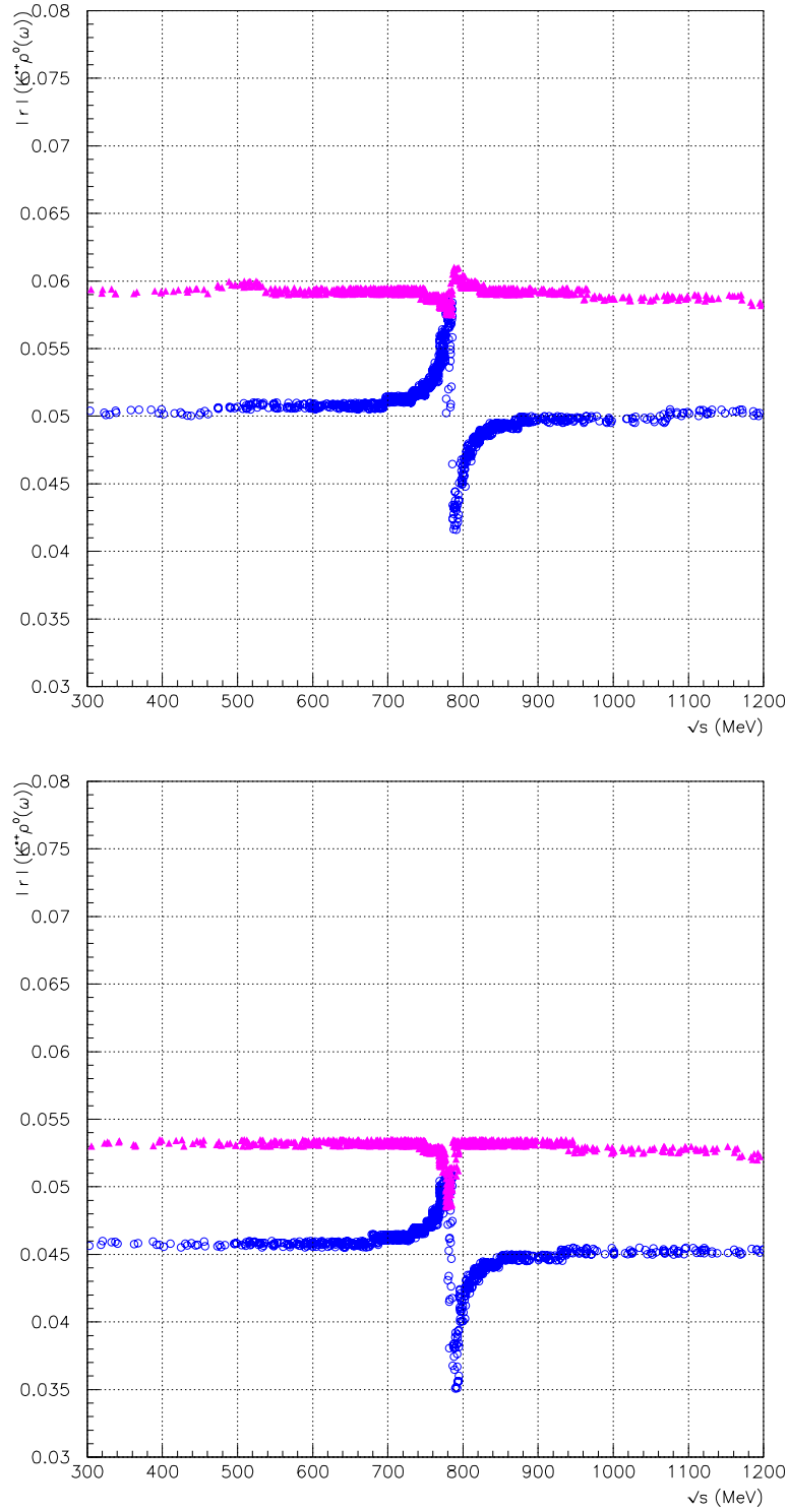
FIG. 5.21: rapport r' entre le module des amplitudes fortes Tree et Penguin en fonction de la masse invariante du système (\pi^+\pi^-) pour le canal B^+ \rightarrow K^{*+} \rho^0(\omega) . Les paramètres utilisés sont le modèle BSW et q^2/m_b^2 = 0.3(0.5) en haut (en bas). Les ronds représentent N_c^{eff} = 2 , les triangles N_{c\ max}^{eff} = 2.84(2.82) .
