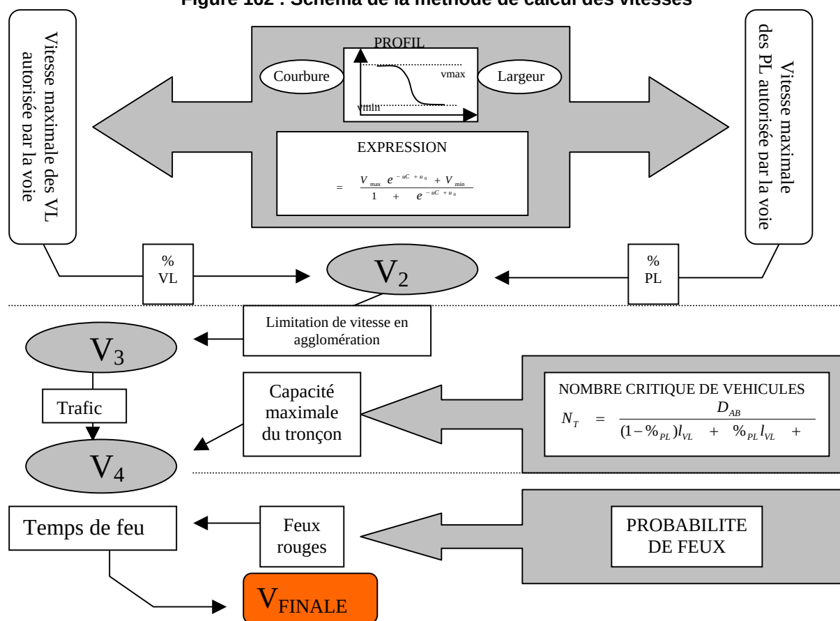
Figure 162 : Schéma de la méthode de calcul des vitesses
