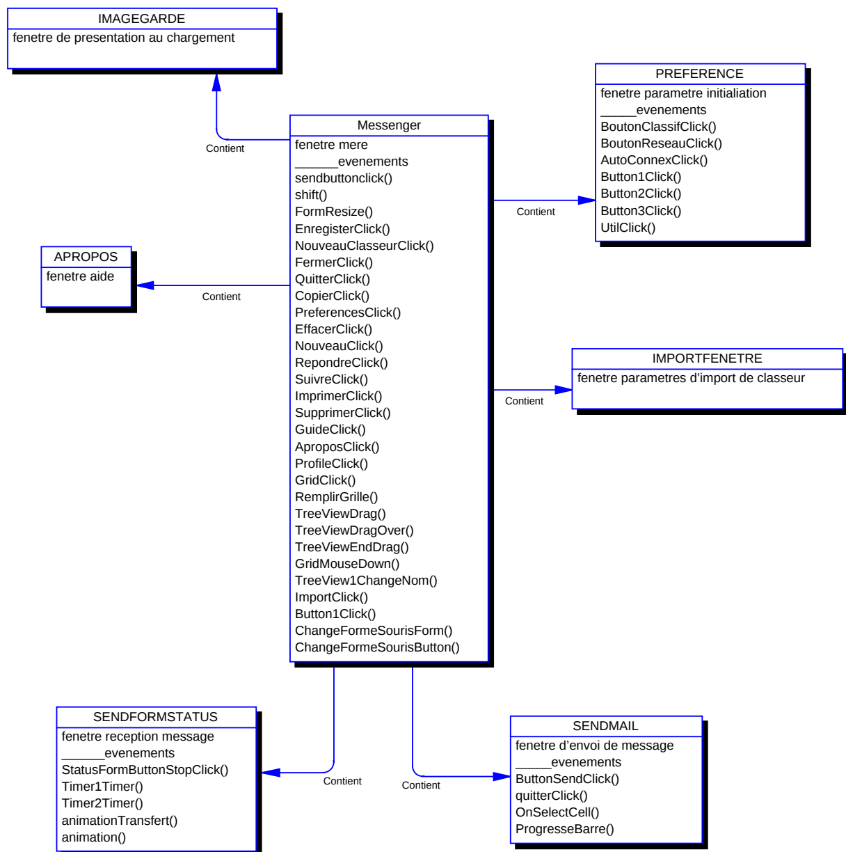
Figure 5.10 Schéma conceptuel des fenêtres graphiques dans Enaïm
