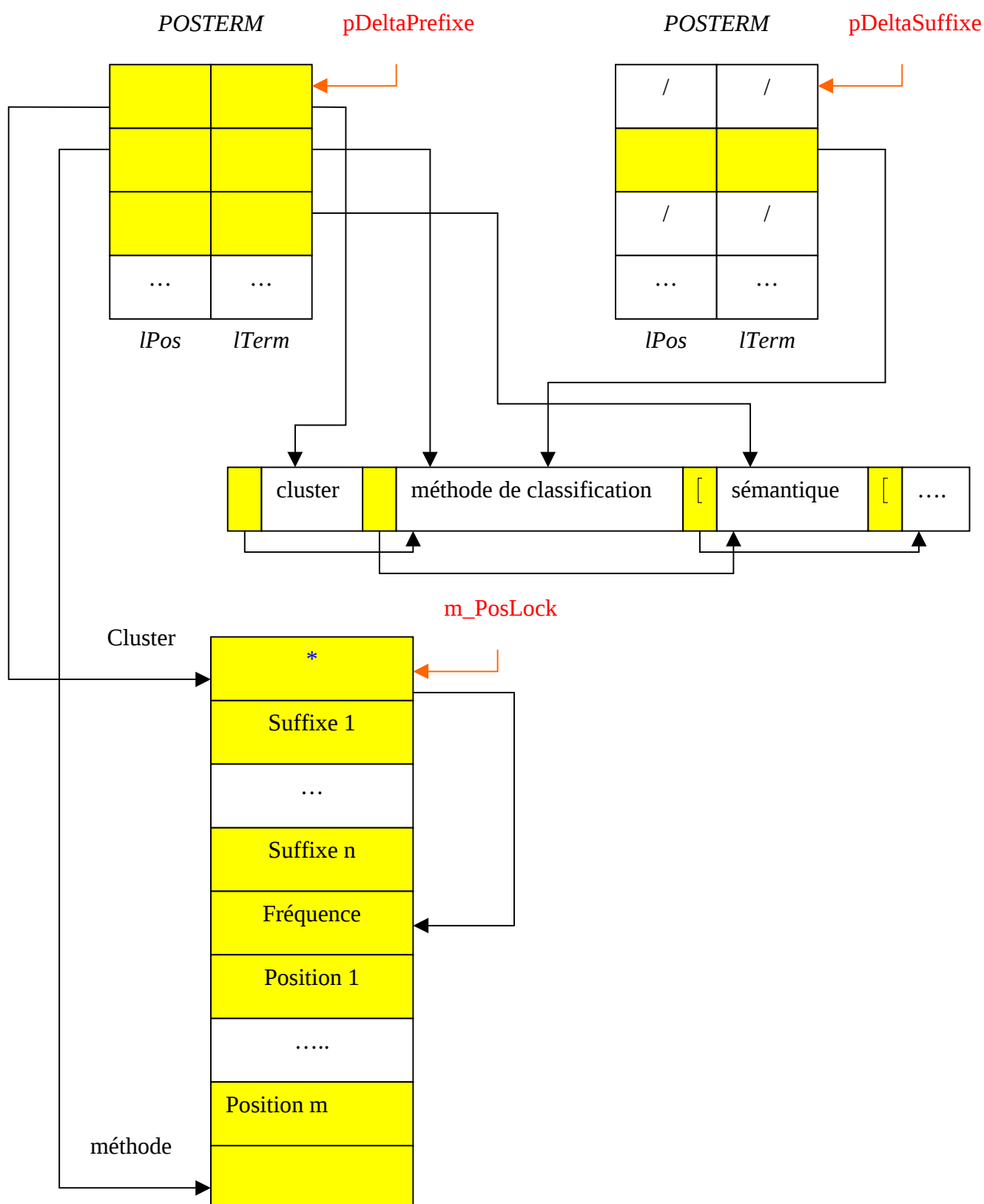
Figure 5 Stockage des termes (monotermes ou multitermes)
