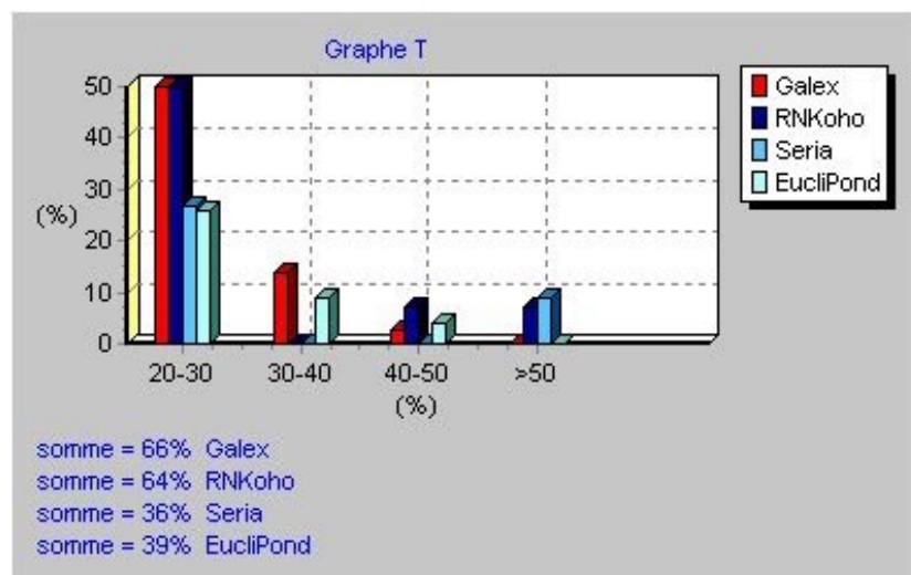
Figure 4.12 Nombre de classes par intervalle de Tmax.
