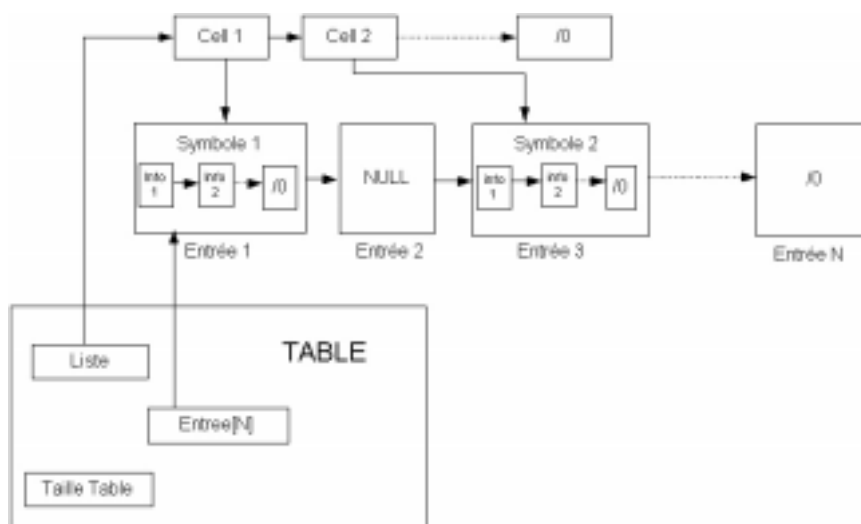
Figure 3.16 Table des symboles
