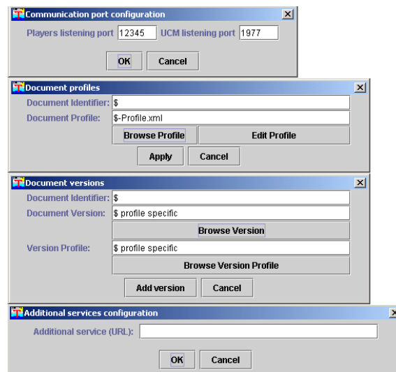
FIG. 3.8 – Menus du module ANM
