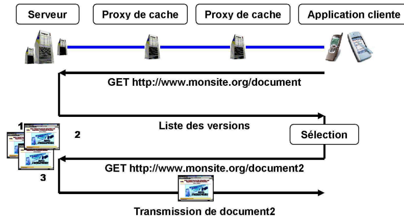
FIG. 2.8 – Modèle de la négociation transparente du contenu
