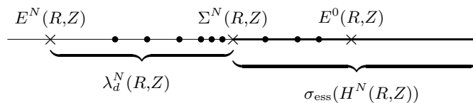
FIG. 1 – Forme générale du spectre de H^N(R,Z)
