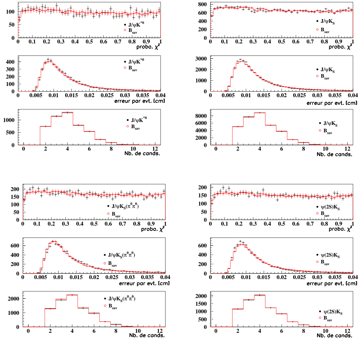
FIG. 8.6 – Événements simulés: comparaison entre les échantillons B_{sav} et CP, pour les événements J/\psi K^{*0}(K_S^0\pi^0) , J/\psi K_S^0(\pi^+\pi^-) , J/\psi K_S^0(\pi^0\pi^0) et \psi(2S)K_S^0 . Trois variables sont comparées: la probabilité de \chi^2 , l'incertitude pour chaque événement, et le nombre de candidats (traces chargées + K_S^0 et \Lambda ) ayant servi à la reconstruction du vertex du B_{tag} . Les distributions sont normalisées au même nombre d'entrées.
