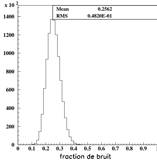
FIG. 7.6 – Distribution des tirages aléatoires de la fraction de bruit de fond.
