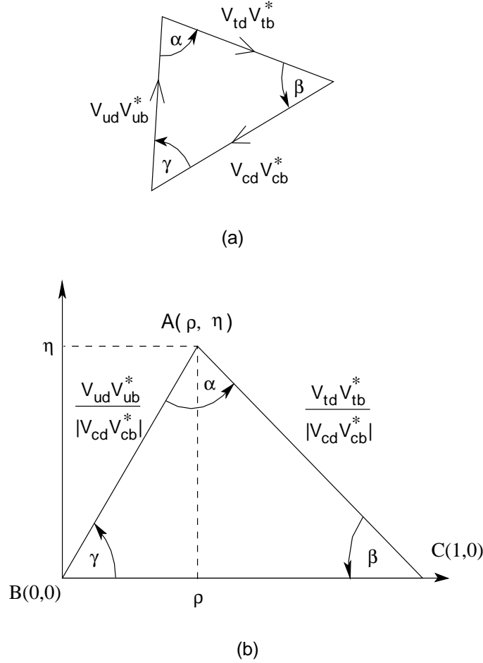
FIG. 2.3 – Représentation géométrique du triangle d'unitarité découlant de 2.21: en toute généralité (a); après rotation et normalisation à l'unité de la base \overline{BC} (b).
