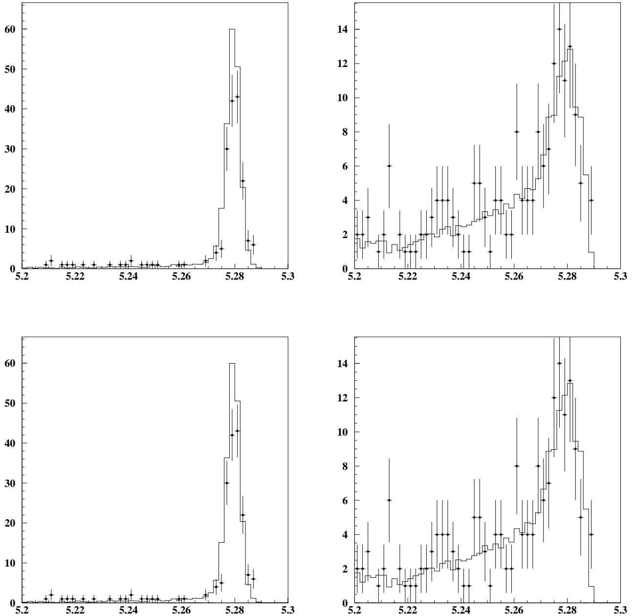
FIG. 7.5 – Distributions de M_{ES} (en \text{GeV}/c^2 ) pour les canaux J/\psi K^{*\pm}(K_S^0 \pi^\pm) (en haut) et J/\psi K^{*\pm}(K^\pm \pi^0) (en bas). A gauche: région du signal en \Delta E ; à droite: région du bruit de fond en \Delta E . Le Monte Carlo est renormalisé à la luminosité des données.
