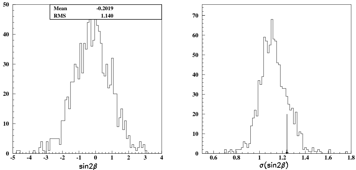
FIG. 10.6 – Résultats d'une étude "Toy Monte Carlo" sur le canal B^0 \rightarrow J/\psi K^{*0}(K_S^0\pi^0) : 1000 expériences sont générées, dans les mêmes conditions que les données. À gauche: distribution des valeurs obtenues de \sin 2\beta ; À droite: distribution des incertitudes correspondantes. La valeur générée de \sin 2\beta est -0.19. La flèche situe le résultat sur les données.
