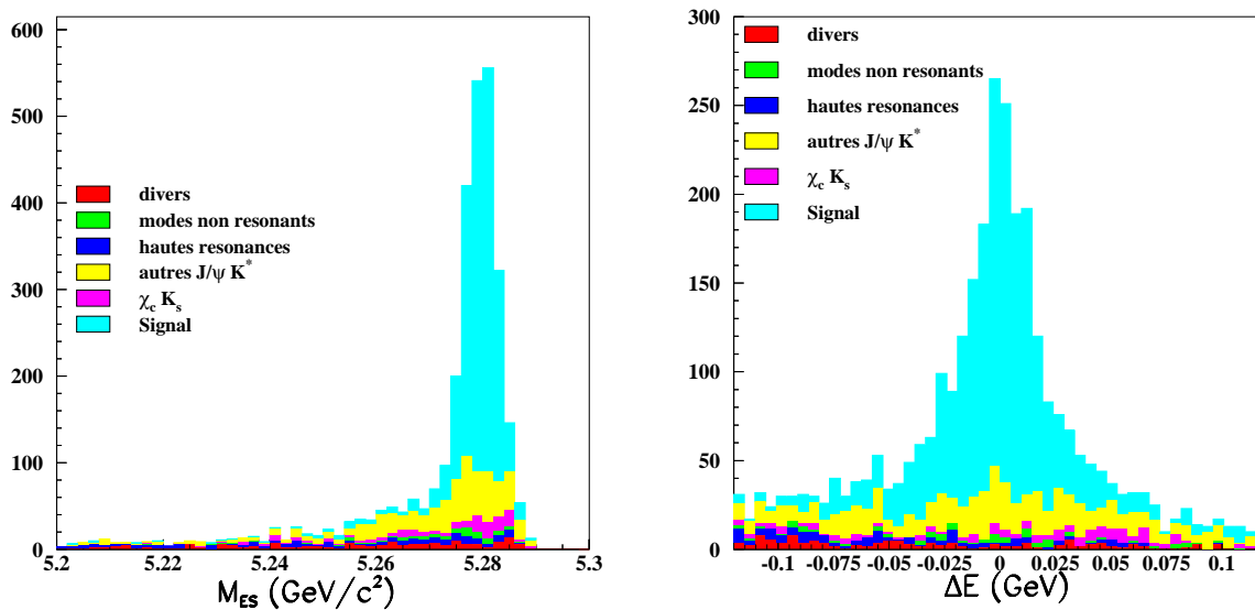
FIG. 7.3 – Distributions en M_{ES} et \Delta E pour les événements sélectionnés dans le canal J/\psi K^{*0}(K_S^0\pi^0) . L'échantillon de départ correspond à 600 \text{ fb}^{-1} J/\psi X générés avec la coupe p^* > 1.3 \text{ GeV}/c . Pour chaque distribution, la coupe sur l'autre variable cinématique est supposée.
