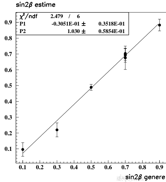
FIG. 10.7 – Comparaison entre les différentes valeurs de \sin 2\beta estimées et leur valeur générée, sur des échantillons simulés (c.f.table 10.8). Comme le montre la figure, ces points sont compatibles avec un alignement sur une droite de pente égale à 1 passant par l'origine.
