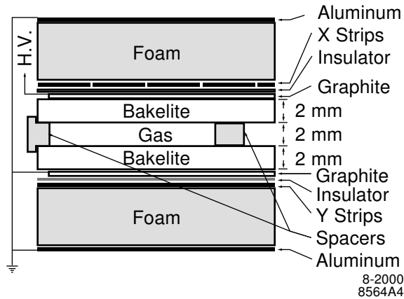
FIG. 4.7 – Schéma de principe d'une RPC.
