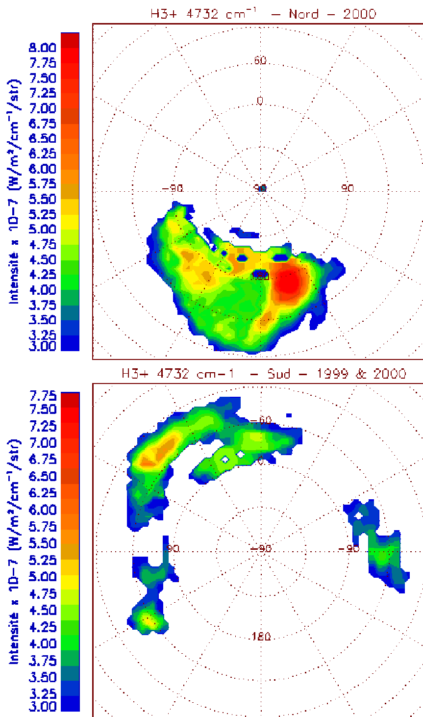
FIG. 9.3 : Emission de H_3^+ pour les cubes du filtre H_2 , calculée par l'intensité de la raie à 4732\text{ cm}^{-1} .
