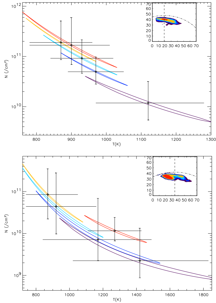
FIG. 9.17 : Domaines de confiance pour les cubes 5 (en bas, la longitude du méridien indiqué est 198°) et 9 (en haut, longitude 225). Pour chaque graphe, la couleur des domaines sont celles des zones correspondantes sur Jupiter (en médaillon).
