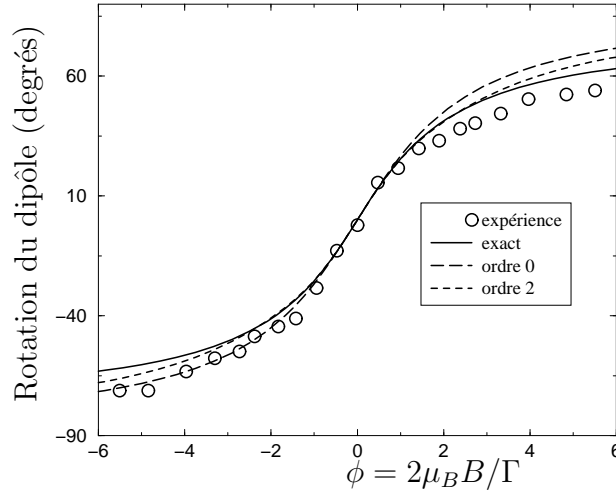
FIG. 3.5 – Angle de rotation de la polarisation diffusée vers l'arrière par rapport à la direction de la polarisation incidente. Les courbes pointillées et tiretées résultent des approximations du développement de la section efficace différentielle (3.38), en puissance de (g - g_e) à l'ordre 0 et à l'ordre 2. L'ordre 0 coïncide avec la rotation du dipôle pour une transition 0 – 1. La ligne continue représente le calcul exact à partir de (3.38) et les cercles sont les valeurs expérimentales mesurées avec des atomes de Rubidium, pour lesquels \phi = 1 correspond à B = 2.1 G.
