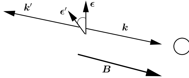
FIG. 3.4 – Schéma pour l'observation de la rotation du dipôle : une onde incidente polarisée linéairement et se propageant suivant \mathbf{B} éclaire un atome. On observe la polarisation du signal diffusé vers l'arrière à travers un analyseur linéaire.
