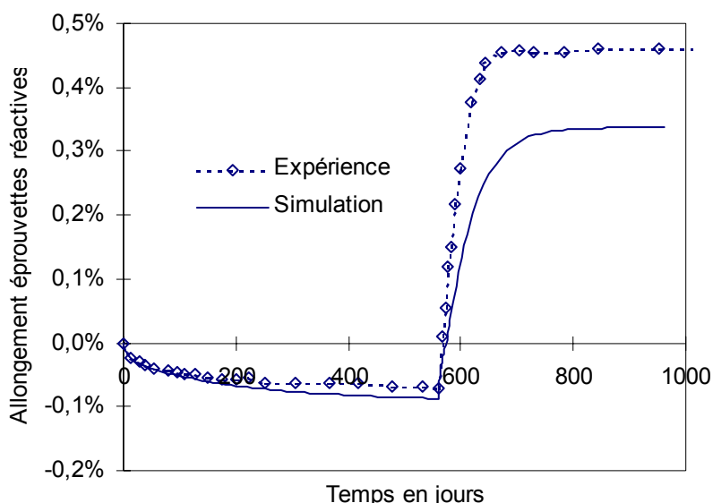
Figure 120 : allongements bruts expérimentaux et simulés d'après [LAR-2000]
