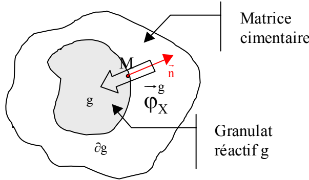
Figure 36 : granulat réactif au sein d'une matrice cimentaire
