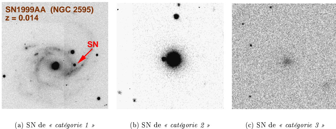
FIG. 6.5 – Exemples de supernovæ de catégories 1, 2 et 3 (de gauche à droite). SN1999aa (à gauche) est une supernova proche qui a explosé dans un bras de NGC2595. La luminosité de la galaxie hôte à l'emplacement de la supernova est faible, de même que ses variations spatiales. Une photométrie d'ouverture avec estimation d'un fond local variable est suffisante pour analyser cette supernova. SN1999bk (au centre) est plus éloignée et plus difficilement distinguable de sa galaxie hôte. Une photométrie d'ouverture n'est plus suffisante. Quant à SN1999at (à droite), seule une photométrie de soustraction peut permettre d'analyser les données.
