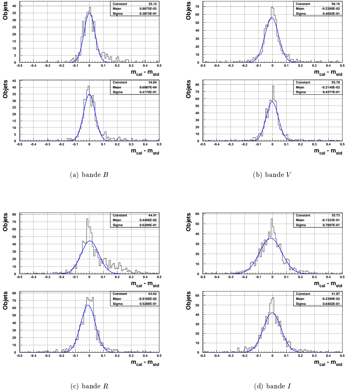
FIG. 6.26 – Dispersion des magnitudes calibrées des objets observés avec le télescope CFHT. On présente dans chaque bande bassante la dispersion des résidus de calibration avant (haut) et après (bas) application des termes de couleur déterminés section 6.5.4.
