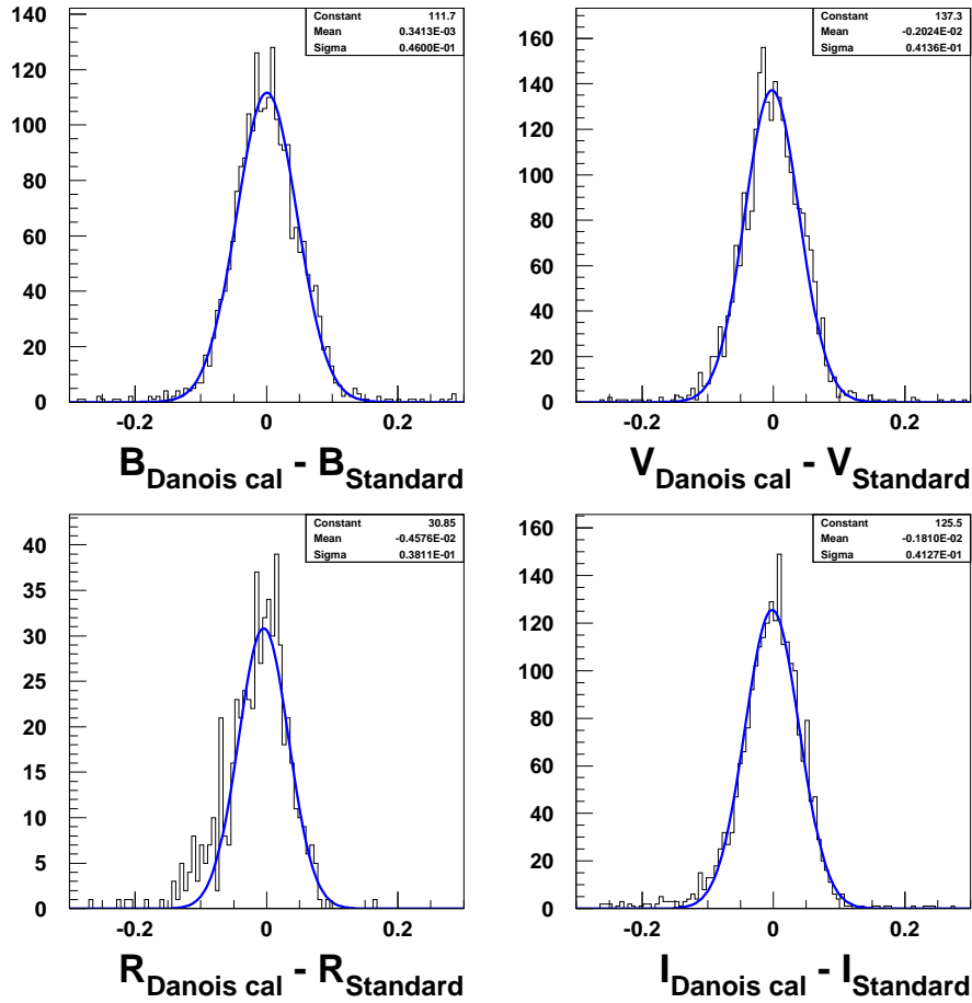
FIG. 6.17 – Télescope 1.54 m Danois : dispersion des magnitudes calibrées, pour les étoiles standard dont les flux ont été mesurés avec le télescope « danois » de 1.54 m. Les étoiles retenues pour cette figure sont de magnitudes comprises entre 15 et 19, dans la gamme de luminosité des SNe que nous étudions. La dispersion obtenue, indépendante de la bande passante, est de 4% environ. Aucun effet résiduel n'est visible, sauf dans la bande R, dans laquelle les magnitudes de certaines étoiles du catalogue sont incertaines.
