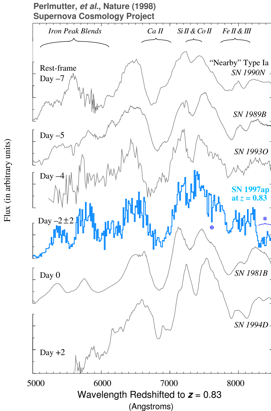
FIG. 2.7 – Spectre d’une supernova lointaine (SN1999ap, z \sim 0.83 ) comparé aux spectres de supernovæ proches pris sensiblement à la même période. Aucune différence notable, n’est observable, ce qui permet de penser que les SNIa proches et lointaines sont similaires. En particulier, on n’observe pas de raie d’absorption due à des poussières interstellaires. Une telle comparaison permet de dater la supernova à 1 ou 2 jours près.
