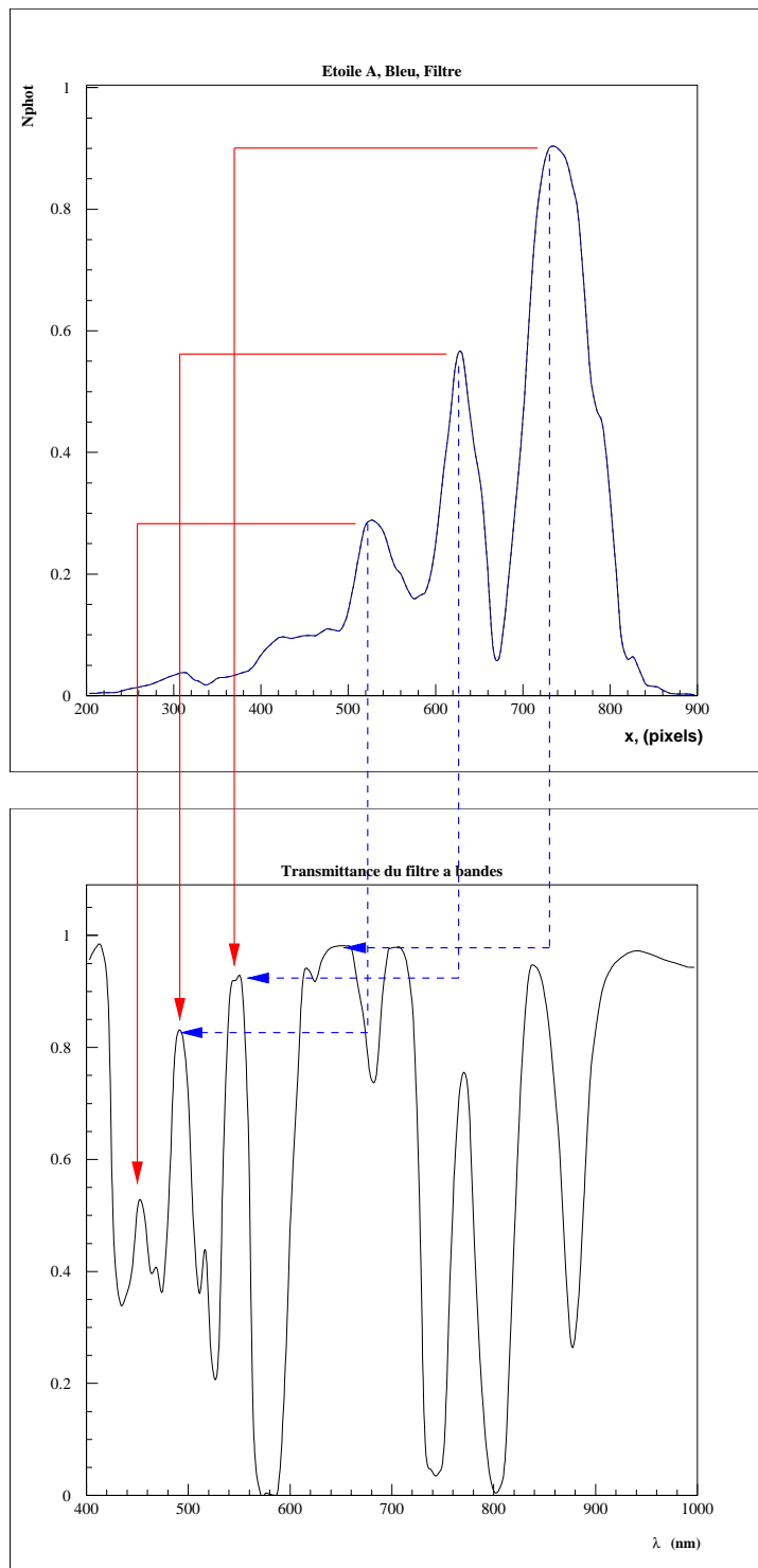
FIG. 4.4 – Illustration de l'indétermination en bleu. Nous comparons ici le spectre de l'étoile A1V pris sur le MARLY, dans la bande bleue, en utilisant le filtre à bandes, avec la transmittance de ce dernier. Il apparaît que les pics ( x = 523 , x = 625 , x = 743 ) peuvent aussi bien correspondre aux maximas ( \lambda = 453 nm, \lambda = 492 nm, \lambda = 547 nm) qu'aux maximas ( \lambda = 492 nm, \lambda = 547 nm, \lambda = 644 nm) du spectre.
