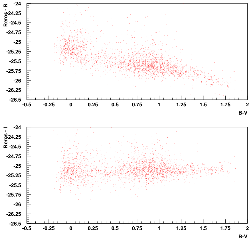
FIG. 4.21 – Comparaison des magnitudes \mathcal{R}_{EROS} et des magnitudes standard R et I. Le filtre \mathcal{R}_{EROS} est « plus rouge » (resp. « plus bleu ») que le filtre standard R (resp. I). Cependant, ici, la pente observée en comparant \mathcal{R}_{EROS} et I est presque nulle : les magnitudes \mathcal{R}_{EROS} sont donc très proches des magnitudes I (à une constante près).
