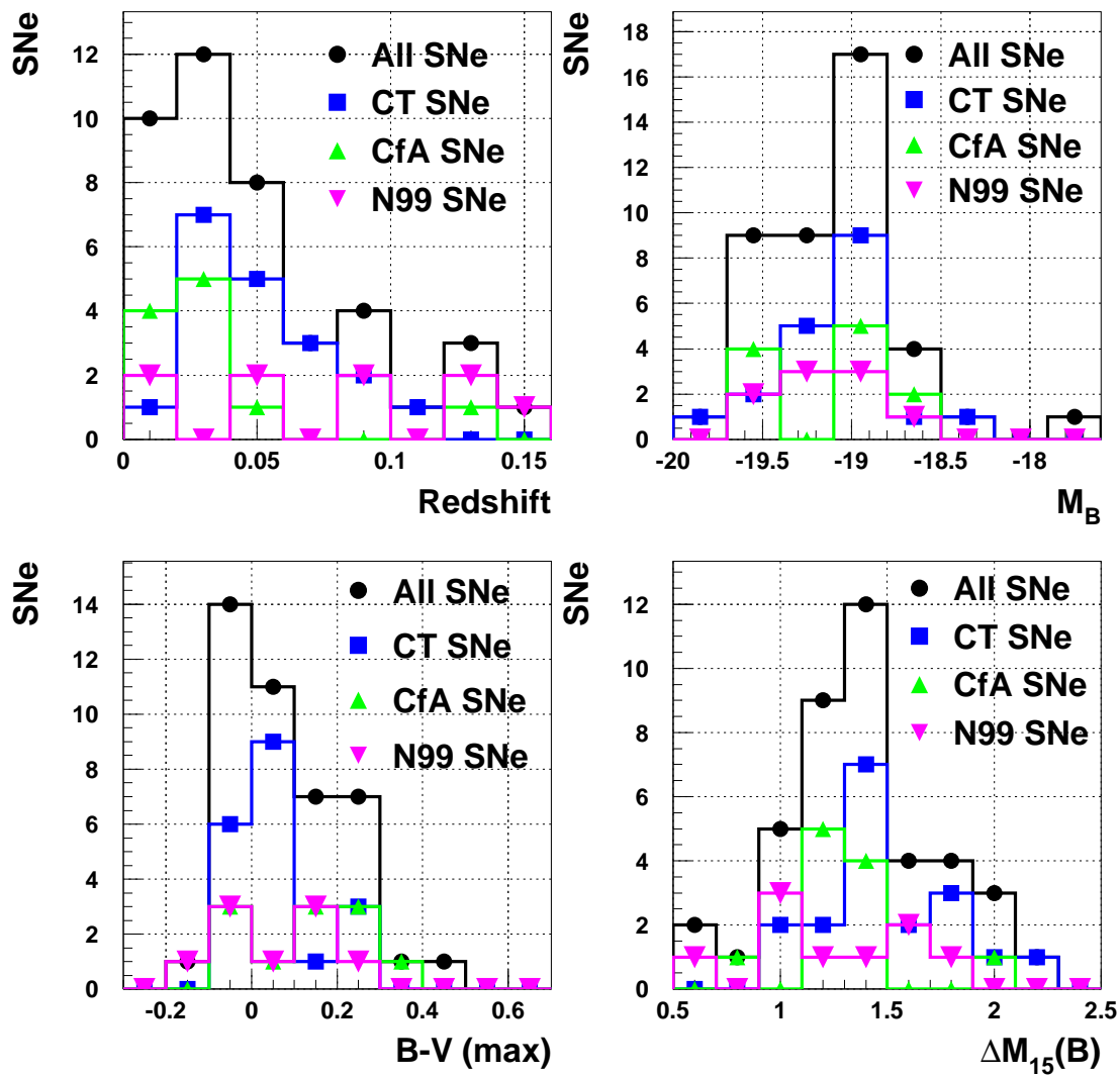
FIG. 8.8 – Distributions de z , M_{max} , (B - V)_{max} et \Delta m_{15} pour les SNIa proches découvertes et étudié par le Calán-Tololo (Hamuy et al., 1996a), le CfA (Riess et al., 1999) ainsi que les SNIa étudiées dans cette thèse (N99).
