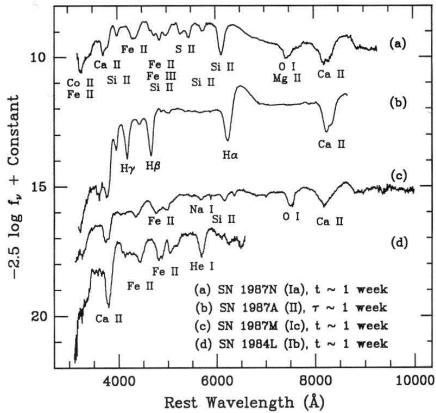
FIG. 2.2 – Spectres de supernovæ de type Ia/Ib/Ic et II. Les SNI sont identifiables par les fortes bandes d'absorption dues à la présence d'hydrogène (raie H\alpha notamment), qui sont absentes des SNIa. Les SNIa présentent de fortes bandes d'absorption dues à SiII et CaII . Du fer, du cobalt (et du nickel) sont également produits en quantités importantes. Les SNIb présentent des raies caractéristiques de l'hélium. Les SNIc ne semblent contenir ni silicium, ni hélium. Remarquer le profil P-Cygni que présentent la plupart des raies d'absorption (la raie H\alpha présente sur le spectre (b), par exemple). Son analyse détaillée permet de mesurer la vitesse d'expansion de l'enveloppe de la supernova (Filippenko, 1997).
