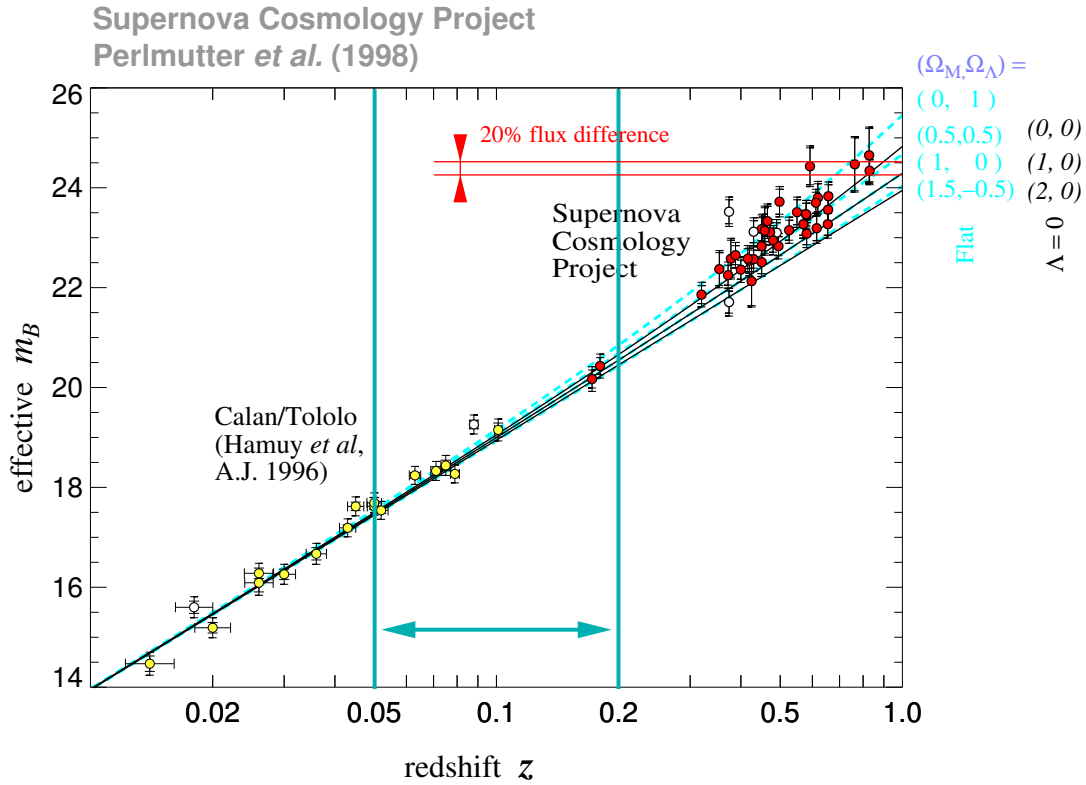
FIG. 1.3 – Diagramme de Hubble réalisé avec 27 SNIa proches ( z \leq 0.1 ) et 42 SNIa intermédiaires ou lointaines ( z \geq 0.2 ). Le lot de supernovæ proches a été constitué par le Calán Tololo Supernova Search tandis que les SNIa lointaines ont été découvertes par le Supernova Cosmology Project. Le paramètre de décélération mesuré est négatif ( q_0 \sim -0.55 ), ce qui indique que l'expansion est en accélération. Noter que cette mesure ne requiert pas de connaître avec précision la valeur de la magnitude absolue moyenne des SNIa. Nous avons indiqué sur la figure le domaine de décalage spectral sondé par EROS II (tiré de (Perlmutter et al., 1998)).
