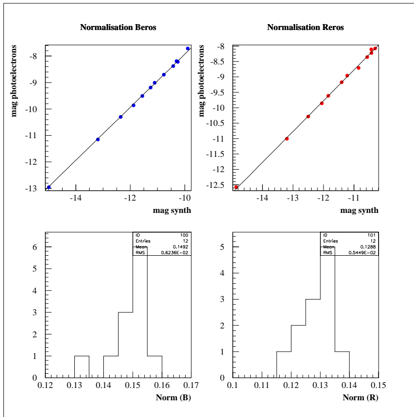
FIG. 4.24 – Comparaison des magnitudes observées ( m_{B|R}^{e^-} ) et synthétiques pour les étoiles de Landolt de la zone SA95 (ca136). En haut : magnitudes observées versus magnitudes synthétiques ; elles sont correctement alignées sur une droite de pente 1, dont l'ordonnée à l'origine est égale à -2.5 \log_{10}(N_{B|R}) . En bas, normalisations en bleues et rouges ( N = 10^{m^{obs} - m^{synth}} ).
