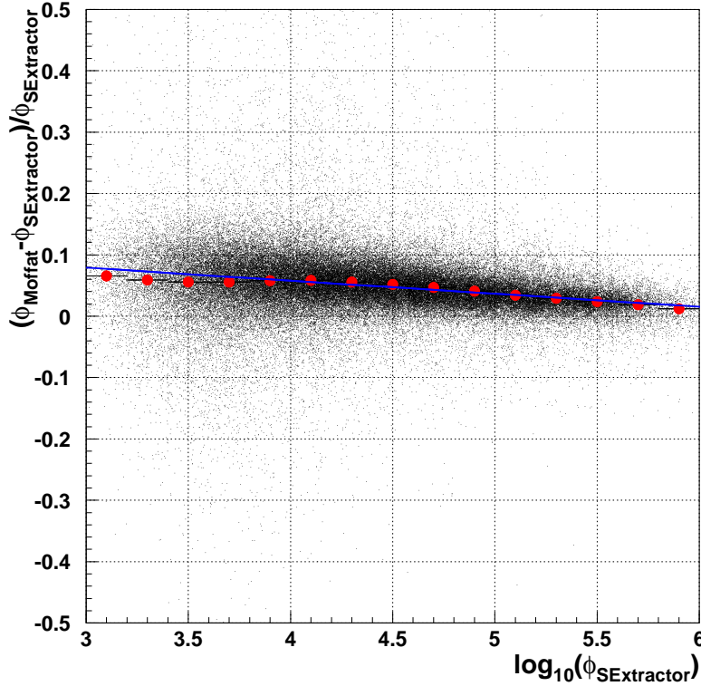
FIG. 6.7 – Comparaison du flux estimé par SExtractor et par une PSF de Moffat. On constate que une photométrie effectuée à l’aide d’une PSF de Moffat conduit à surestimer le flux des étoiles de 2 à 5%. Ce biais est corrigé en moyenne par le processus de calibration décrit section 6.5. Par contre, la dépendance en flux de ce biais aura tendance à dégrader notre résolution photométrique.
