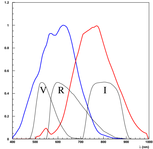
FIG. 3.3 – Transmittances du MARLY, déterminées au chapitre 4, et filtres standards VRI. Les normalisations sont arbitraires. Les filtres EROS sont beaucoup plus larges que les filtres standards. La voie \mathcal{B}_{EROS} se situe à peu près entre le V_j et le R_c . La voie \mathcal{R}_{EROS} est beaucoup plus proche de la bande I standard.
