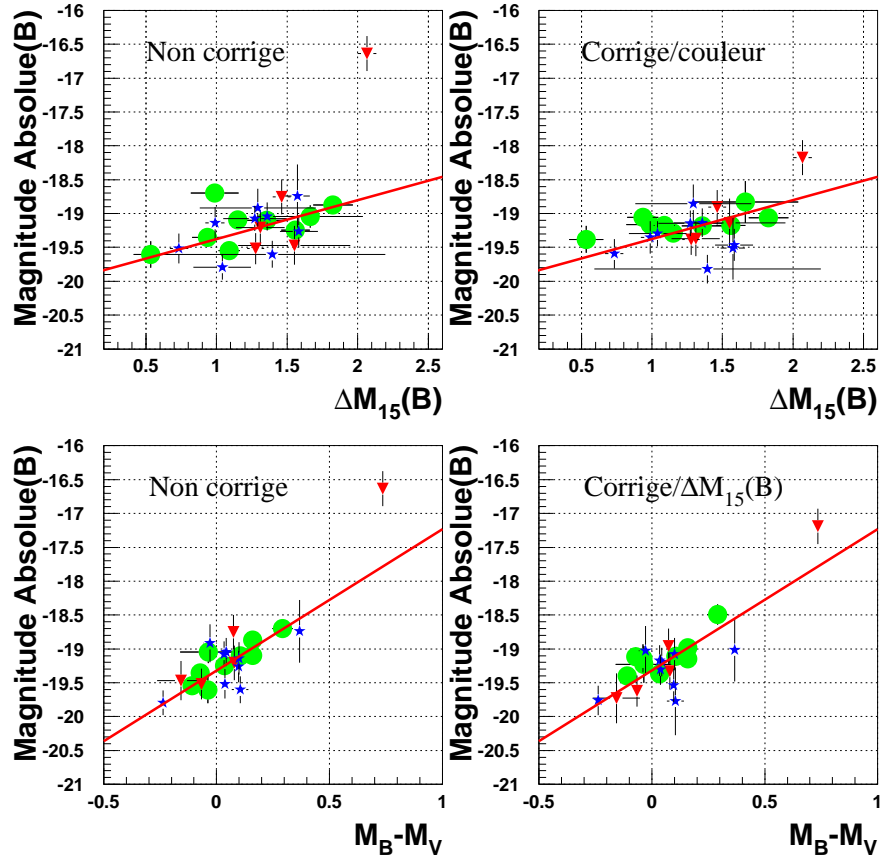
FIG. 8.10 – Corrélations M_{max} vs couleur et M_{max} vs. \Delta m_{15}(B) pour les SNIa découvertes en 1999 et les calibrateurs.
