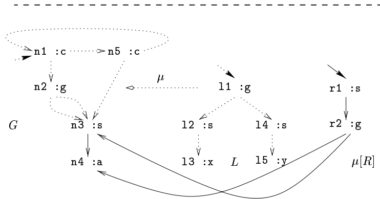
(a) Filtrage de L sur G_{|n2} avec l'homomorphisme \mu
