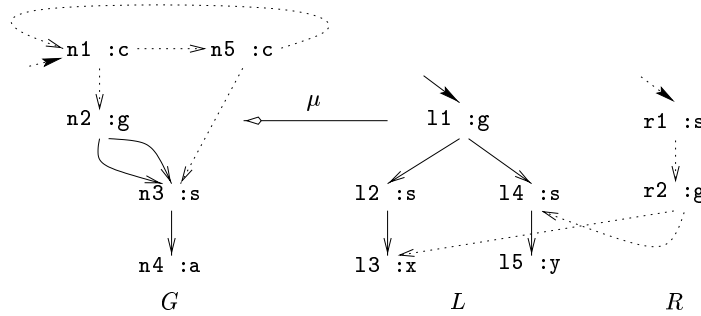
(a) Filtrage de L sur G_{|n2} avec l'homomorphisme \mu
