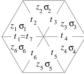
Fig. 9: Les 6 variables de liens et les 6 paires de spins autour d'un nœud.
