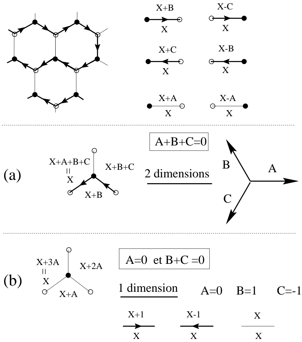
Fig. 20: Définition des variables de hauteur X pour le gaz de boucles sur réseau hexagonal. La règle utilise explicitement le bicoloriage des nœuds du réseau hexagonal. Dans le cas de boucles compactes, seul l'environnement (a) est rencontré (modulo des symétries évidentes), et la cohérence des définitions des hauteurs impose A + B + C = 0 . Dans le cas de boucles non compactes, la présence de nœuds non visités avec l'environnement (b) impose de plus que A = 0 , auquel cas B = -C ( = 1 par exemple) et les règles deviennent insensibles au bicoloriage des nœuds du réseau hexagonal.
