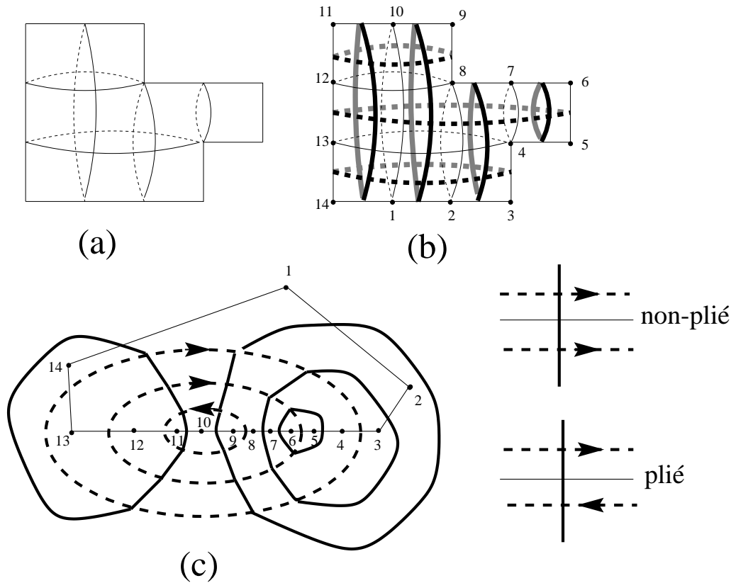
Fig. 54: Exemple de quadrangulation planaire pliable (a) en représentation sphérique. Les boucles compactes noires et blanches correspondantes (b) sont entièrement fixées. Seule leur orientation reste arbitraire. Les mêmes boucles en représentation planaire forment une configuration du modèle GFPL 2 . L’orientation des boucles blanches détermine les liens horizontaux pliés selon la règle représentée à droite. Une règle similaire détermine les liens verticaux pliés en fonction de l’orientation des boucles noires (non représentée ici). Pour la configuration de boucles considérée, les liens du “périmètre” joignant les nœuds notés 1 à 14 sont toujours pliés quelle que soit l’orientation des boucles noires et blanches . Les autres liens peuvent ou non être pliés. Par exemple, le choix particulier d’orientation des boucles blanches représenté en (c) correspond à avoir fait un pli horizontal entre les points 12 et 8 sur la représentation (b), pliant ainsi quatre liens.
